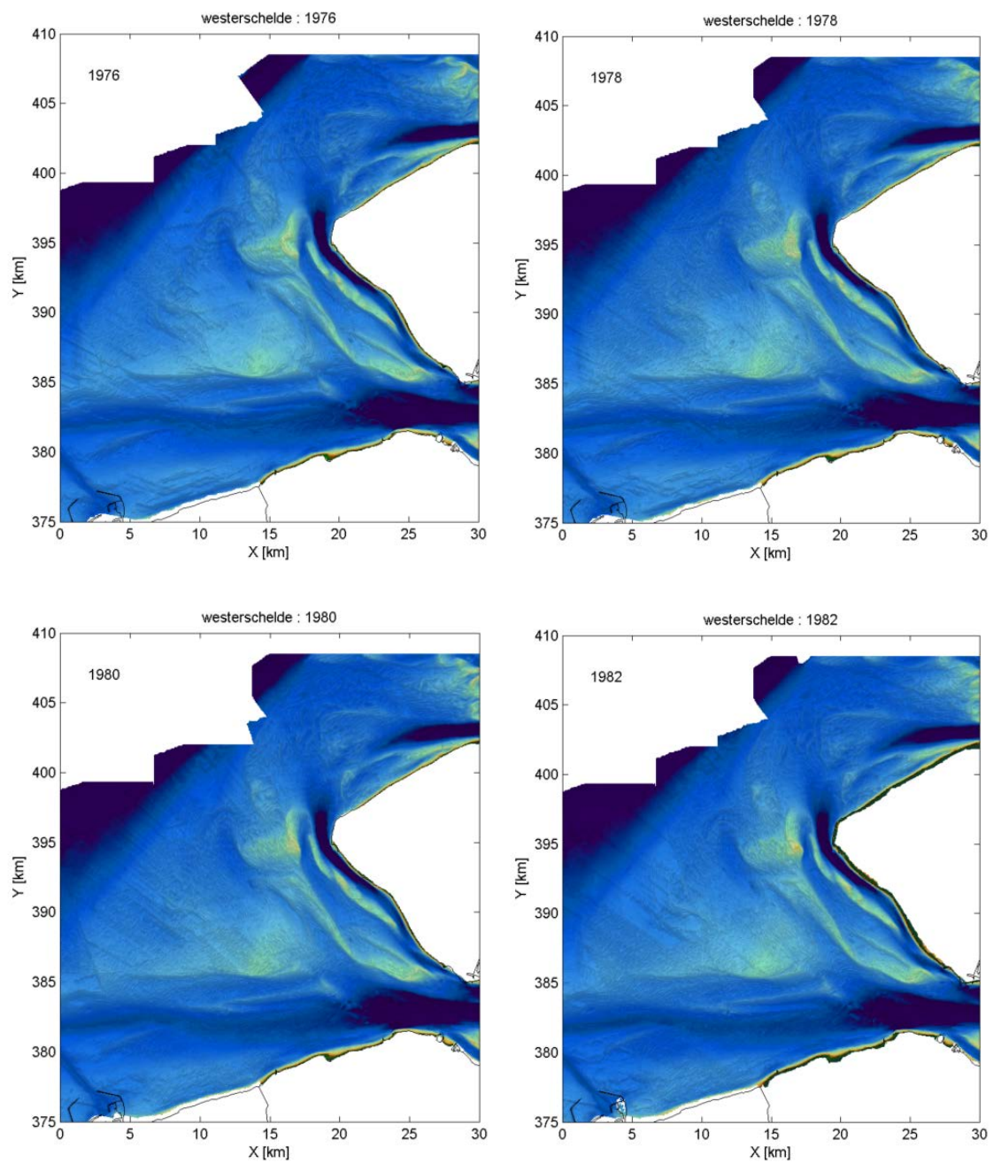
Figuur A.2 Samengestelde (geselecteerde) kaarten Westerscheldedemoning 1976, 1978, 1980, 1982
