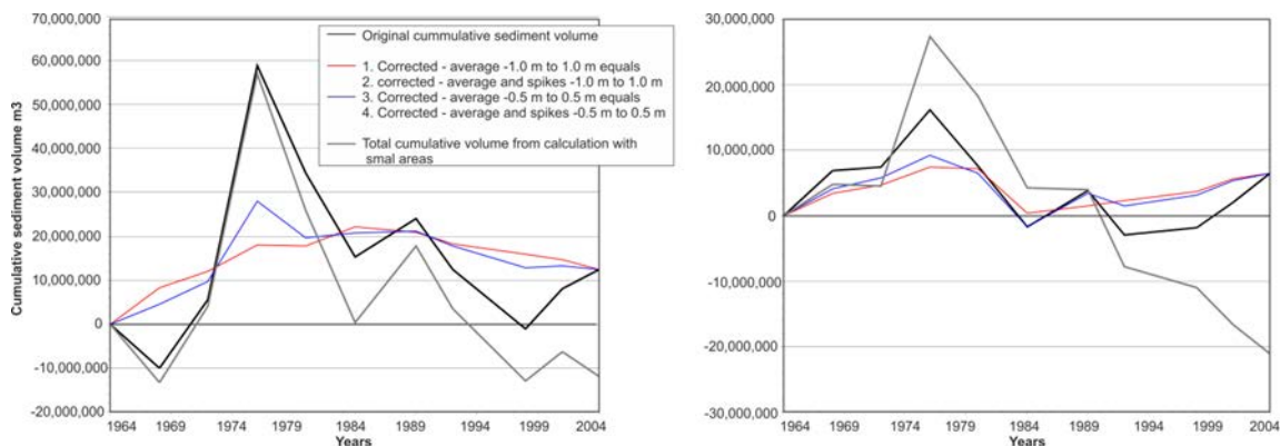
Figuur 3.4 Sedimentbalans Westerscheldemonding voor deelgebieden: Vlake van de Raan (links) en Wielingen (rechts). Gebaseerd op Cleveringa et al. (2008).
