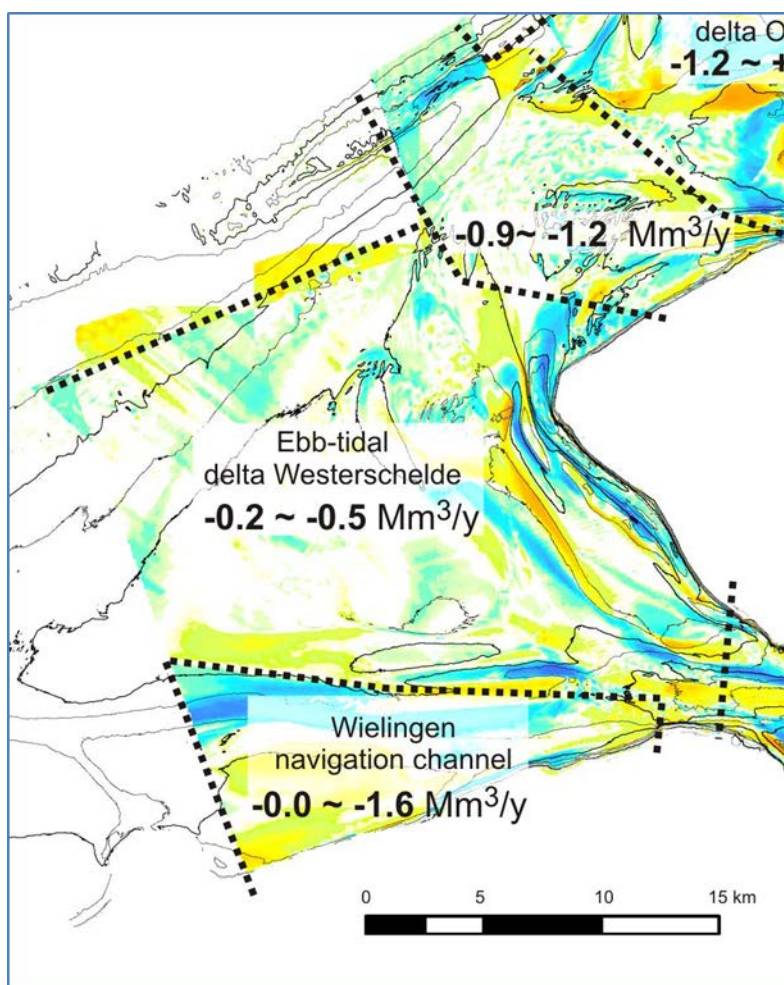
Figuur 3.3 Trend van volumeverandering in de periode 1976/1980 tot 2004 voor de verschillende deelgebieden van de Westerscheldemonding (gebied 5: buiten delta Westerschelde en gebied 6: Wielingen). De onderliggende kaart geeft het sedimentatie-erosie patroon over de periode 1964-2004). Overgenomen uit Cleveringa (2008).
