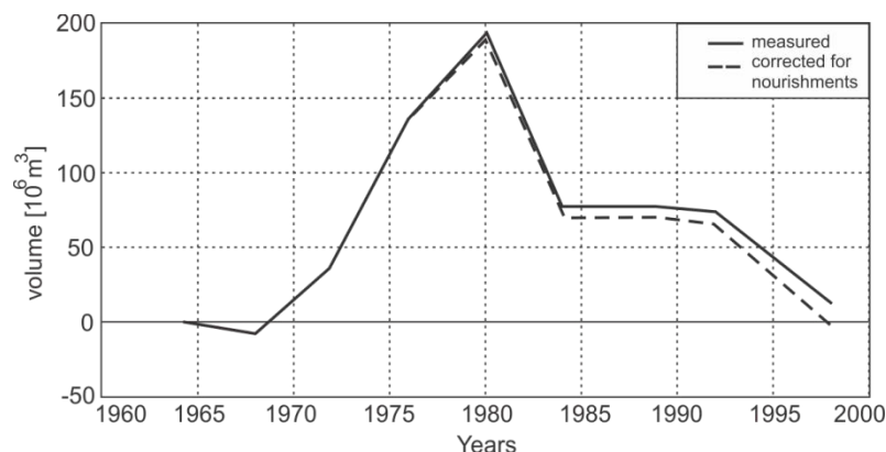
Figuur 3.2 Zandvolumeverandering van de Westerscheldemonding (Walburg, 2005). Zie Figuur 2.1 (rode polygoon 4) voor afbakening balansgebied.
