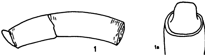
Fig. 1. Caecum clarkii Carpenter; Zeeland, Cadzand. Lengte 2,2 mm; doorsnede mondopening 0,45 mm; doorsnede bij septum 0,35 mm; lengte septumuitsteeksel (zie fig. 1a) 0,14 mm.
