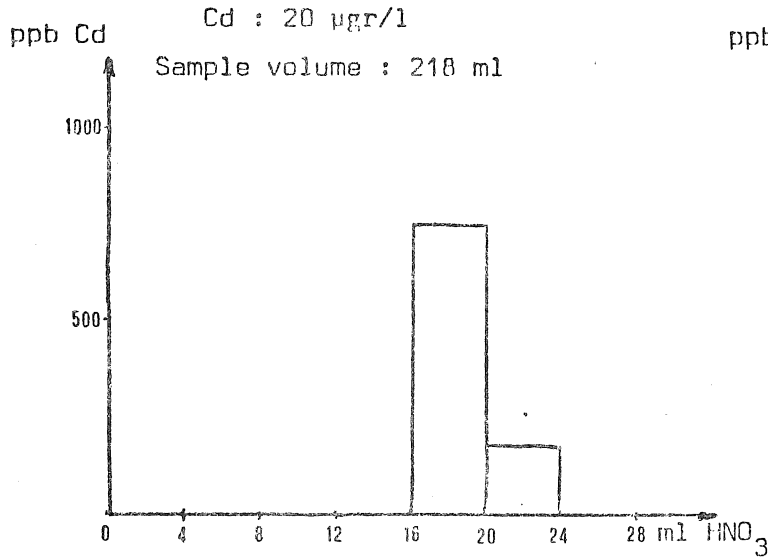
Fig. 3 : Cadmium elution
