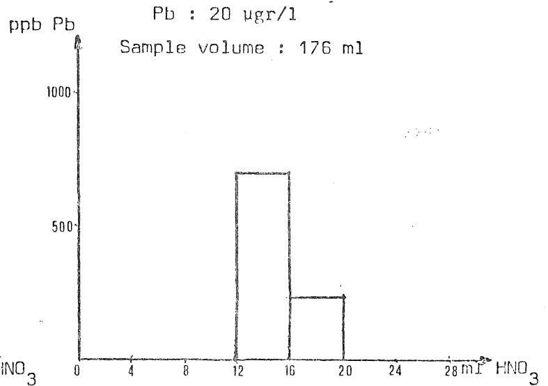
Fig. 4 : Lead elution
