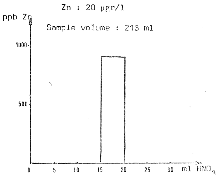
Fig. 1 : Zinc elution
