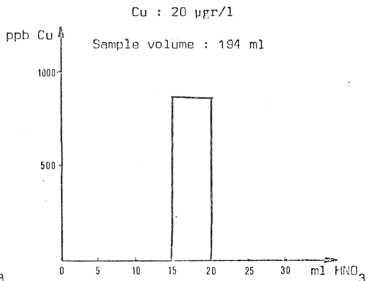
Fig. 2 : Copper elution
