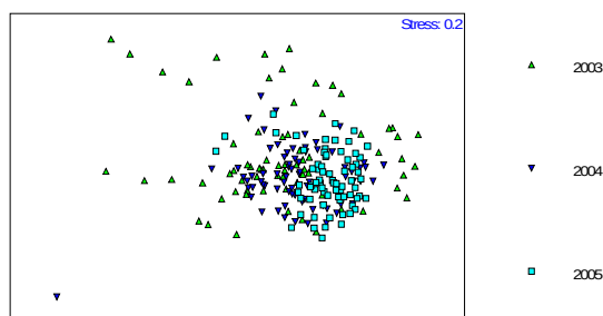
Jassa marmorata
