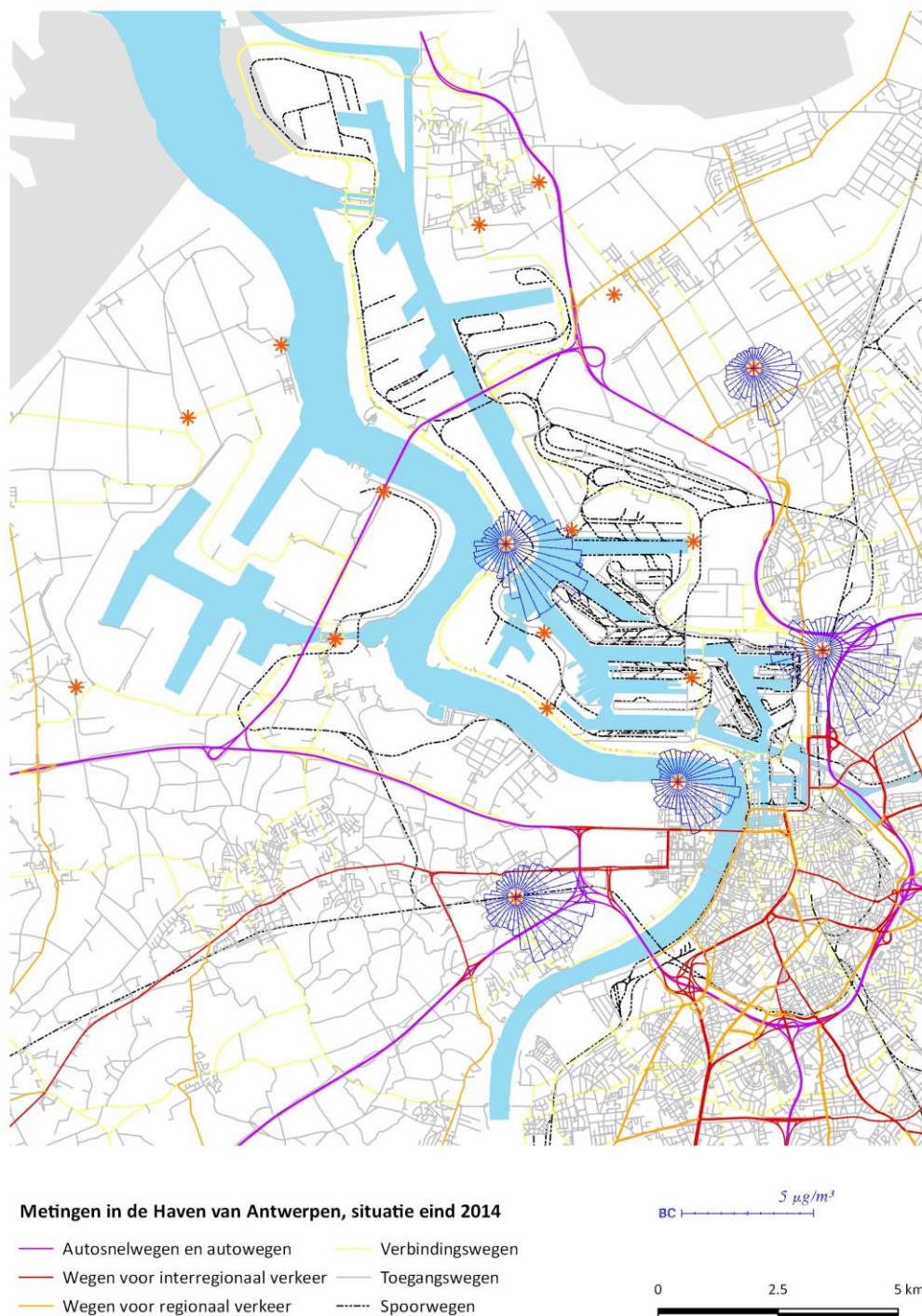
Figuur 30: Pollutierozen gemiddelde concentraties zwarte koolstof in het Antwerpse havengebied in 2014
