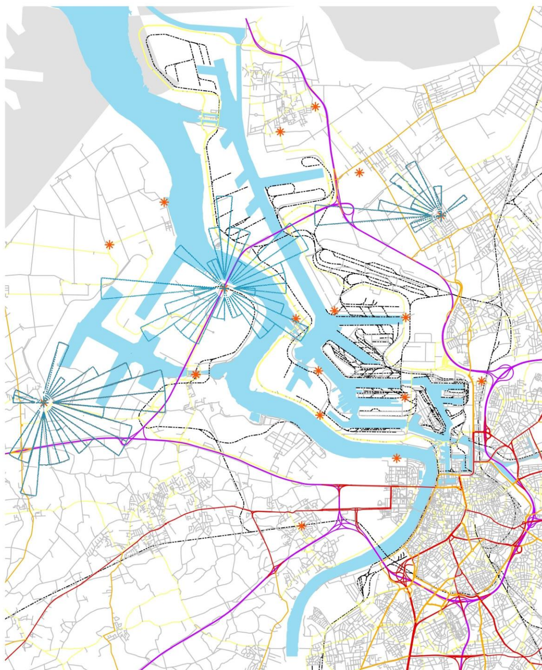
Figuur 28: Zeropollutierozen gemiddelde PM 2,5 -concentratie in Antwerpse havengebied in 2014
