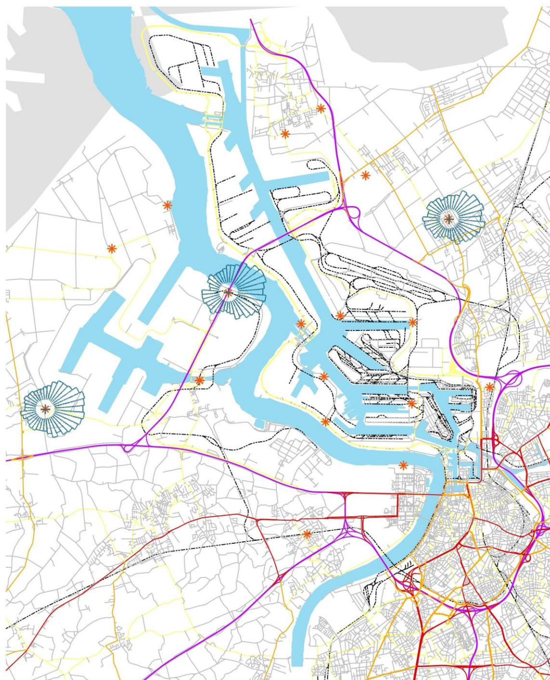
Figuur 27: Pollutierozen gemiddelde PM 2,5 -concentraties in het Antwerpse havengebied in 2014
