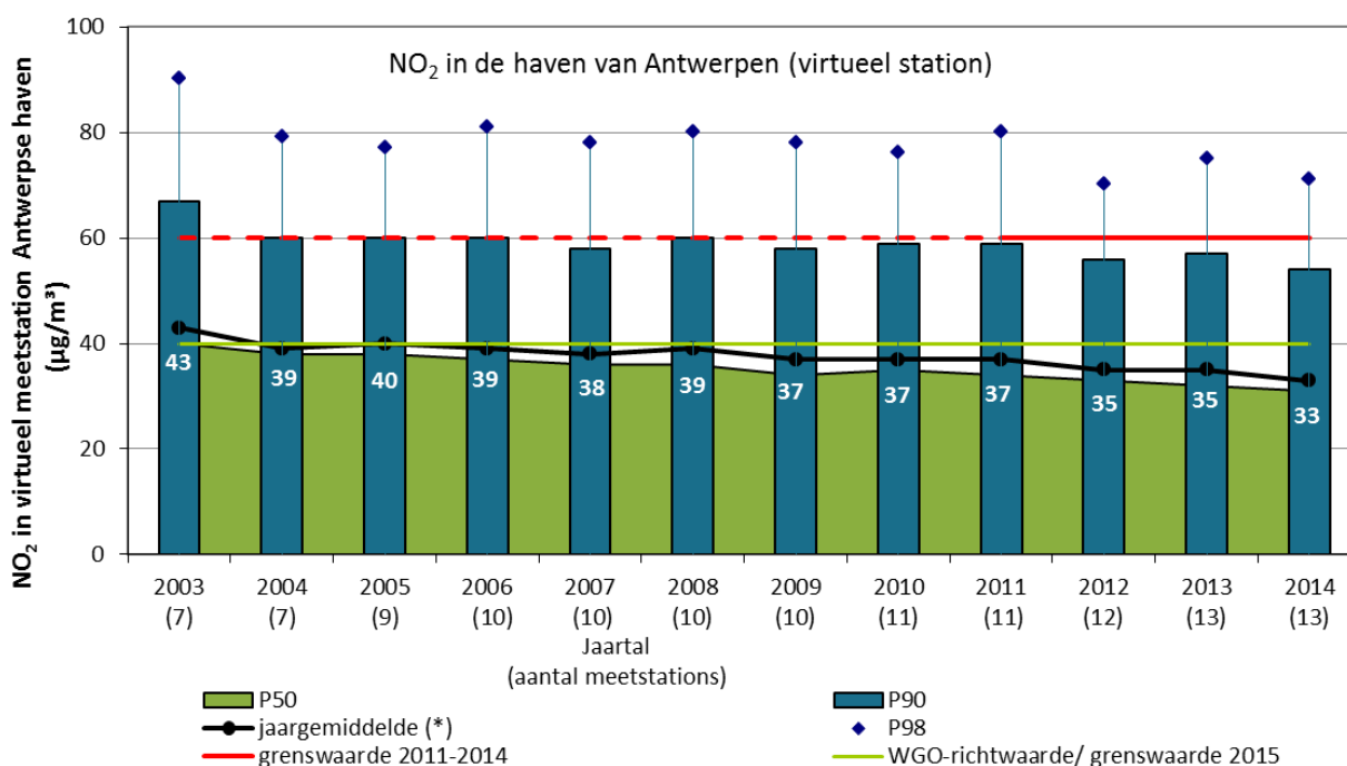
Figuur 12: Evolutie NO 2 -jaargemiddelde in het Antwerpse havengebied (2003-2014)
