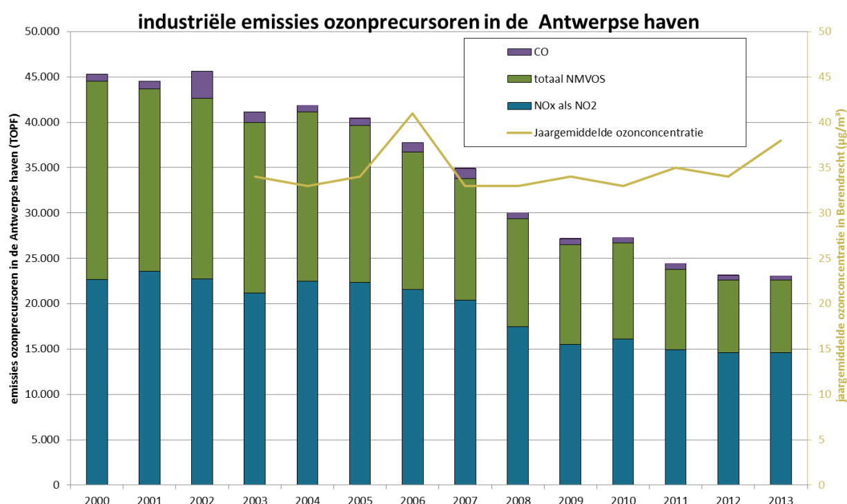
Figuur 32: Industriële emissies van ozonprecursoren in het Antwerpse havengebied (2000-2013)
