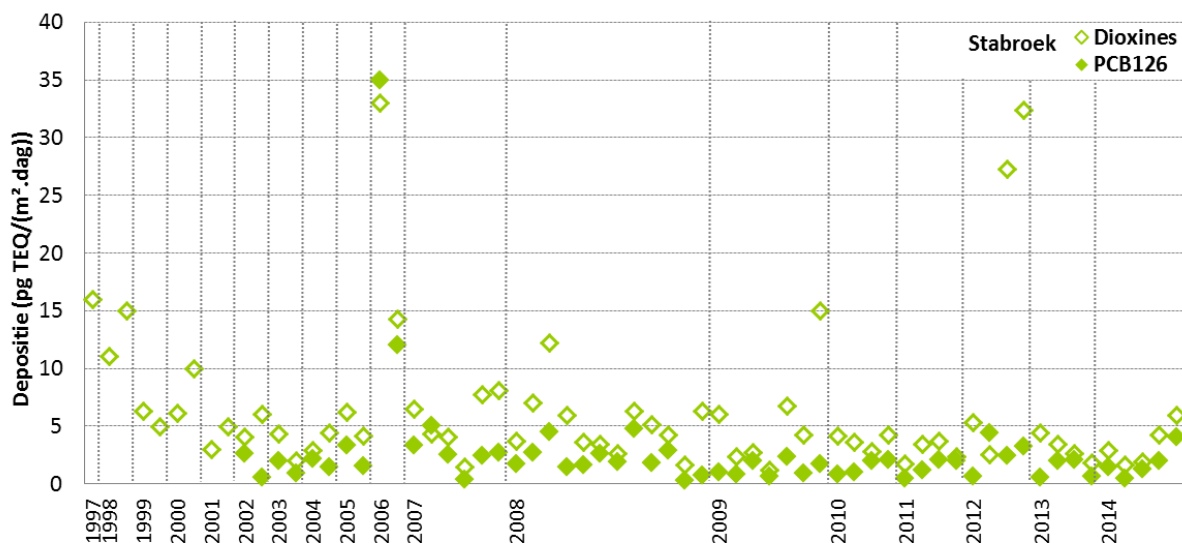
Figuur 39: Trend depositie dioxines en PCB126 op meetplaats R833 in Stabroek (agrarisch gebied)
