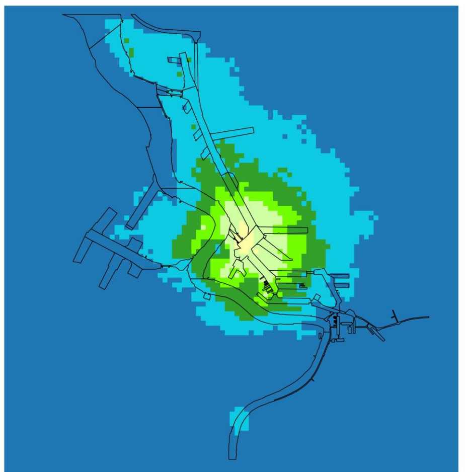
Figuur 6: Gemodelleerd SO 2 -jaargemiddelde in de Antwerpse haven in 2014
