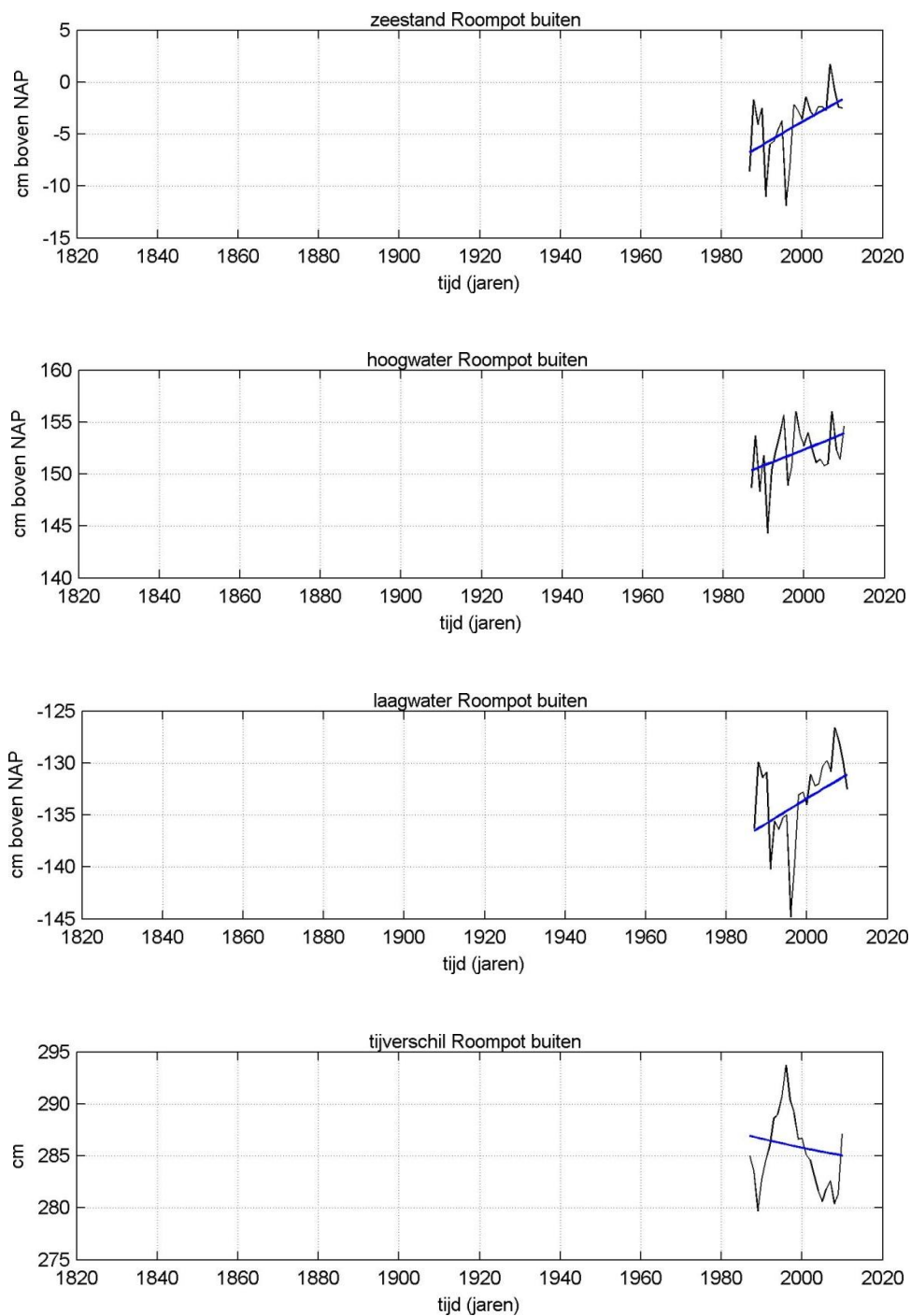
Figuur C.11 Verloop jaargemiddelde zeenniveaus Roombot buiten
