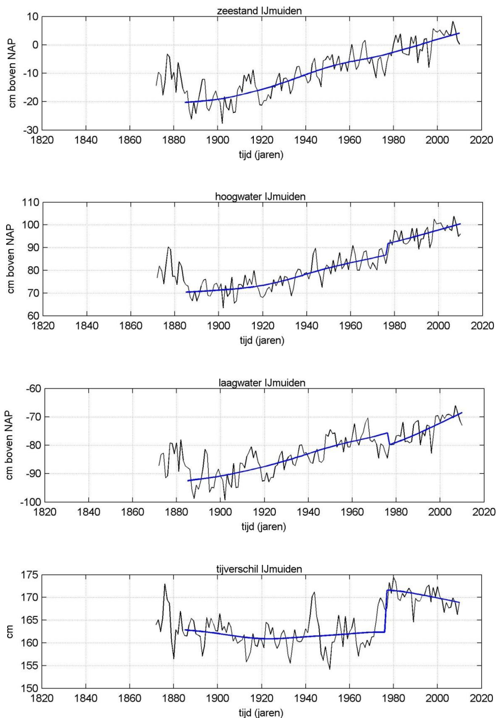
Figuur C.16 Verloop jaargemiddelde zeenniveaus IJmuiden Analyseperiode vanaf 1885
