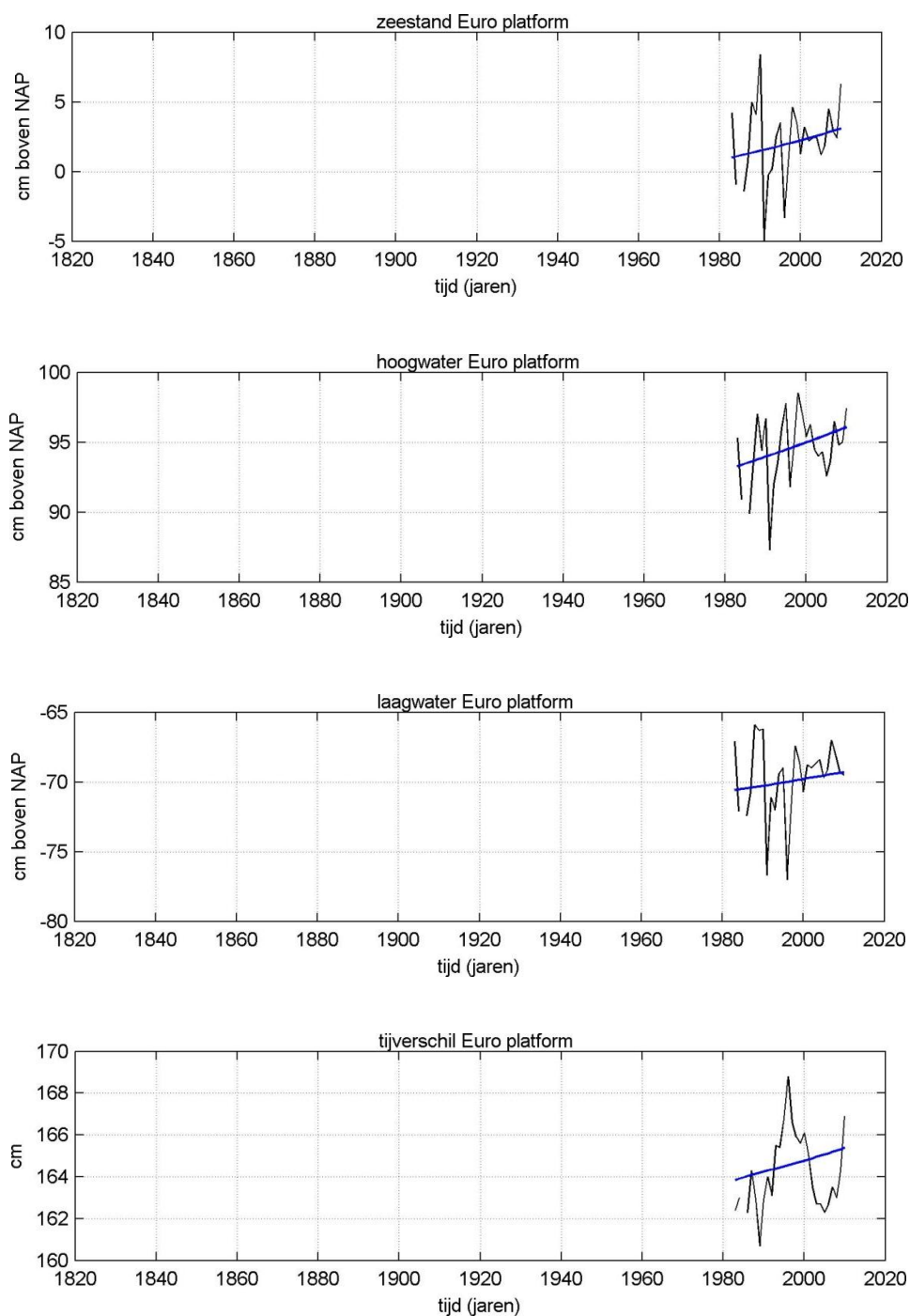
Figuur C.35 Verloop jaargemiddelde zeenniveaus Euro platform. Data t.o.v. op zeker tijdstip bepaalde lokale gemiddelde zeespiegel. NAP ter plaatse niet ingemeten.
