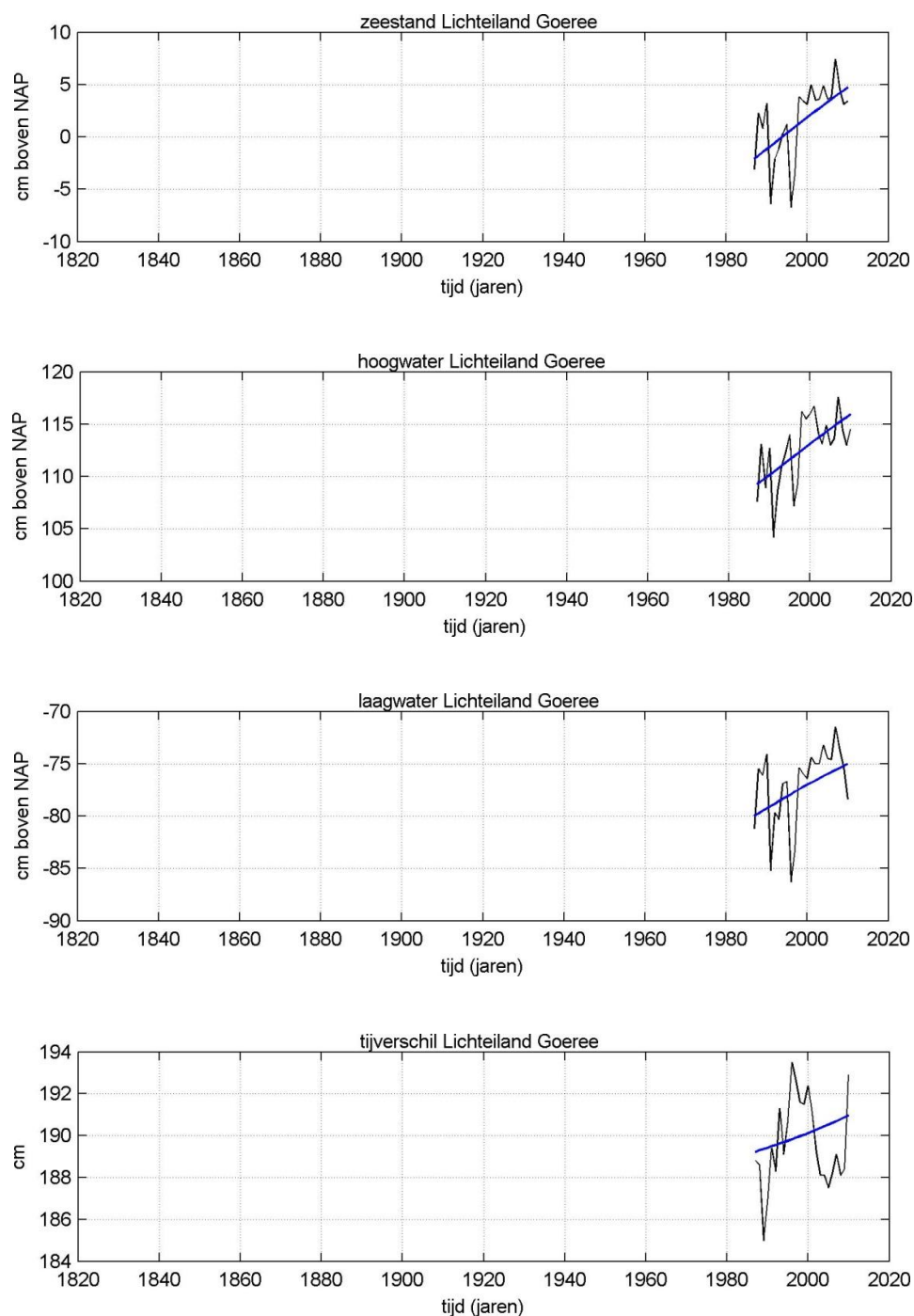
Figuur C.37 Verloop jaargemiddelde zeenniveaus Lichteiland Goeree. Data t.o.v. op zeker tijdstip bepaalde lokale gemiddelde zeespiegel. NAP ter plaatse niet ingemeten.
