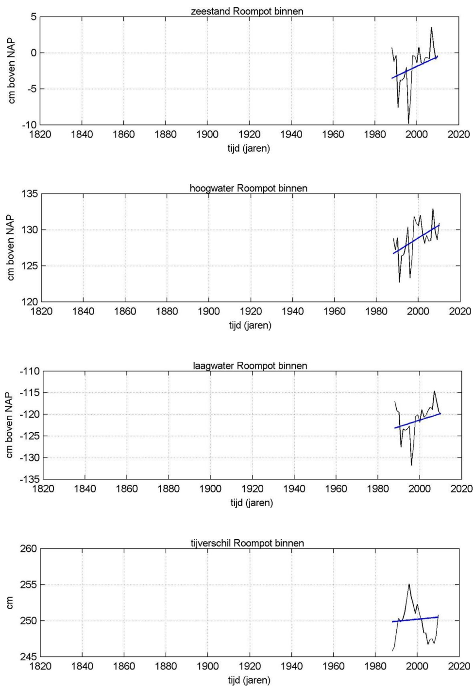
Figuur C.10 Verloop jaargemiddelde zeeniveaus Roombot binnen
