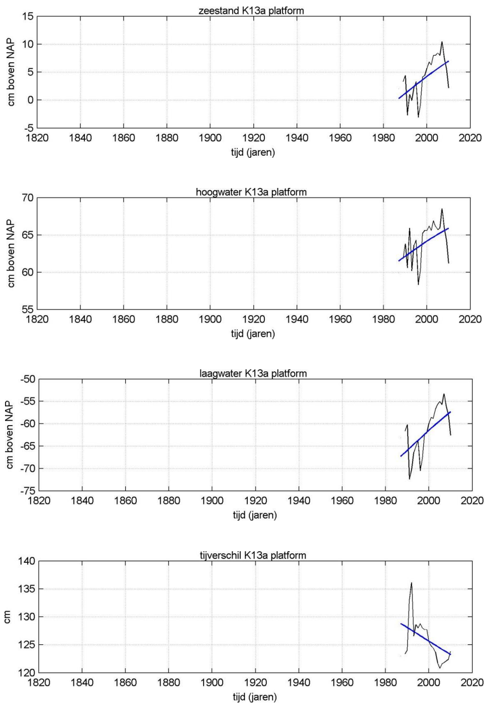
Figuur C.36 Verloop jaargemiddelde zeenniveaus K13a platform. Data t.o.v. op zeker tijdstip bepaalde lokale gemiddelde zeespiegel. NAP ter plaatse niet ingemeten.
