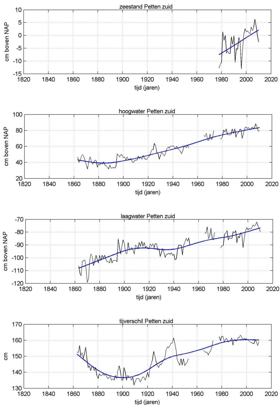
Figuur C.17a Verloop jaargemiddelde zeenniveaus Petten zuid
