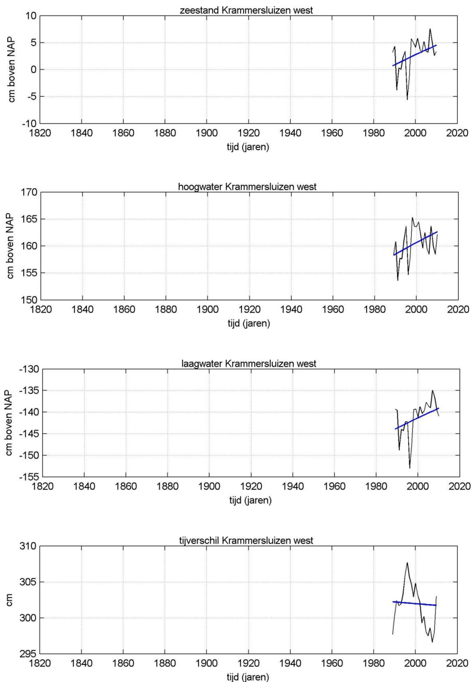
Figuur C.9 Verloop jaargemiddelde zeenniveaus Krammersluizen west
