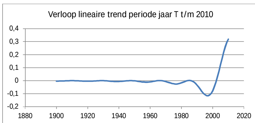
Figuur 3.2.4 Verloop van de lineaire trend in de sinusoïde van Figuur 3.1.1 over de periode vanaf jaar T tot en met jaar 2010.
