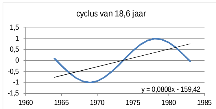
Figuur 3.2.2 De lineaire trend in een knopencyclus over de periode 1964-1983, waarbij de amplitude van het sinusvormige signaal is gesteld op 1.
