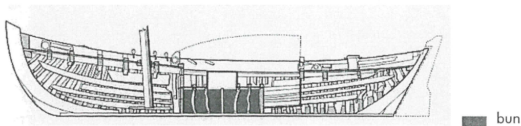
Fig. 2. Reconstructie-longsdoorsnede van een 16de-eeuws, karveel gebouwd waterschip met een lengte van 20 m. (tekening NISA)
