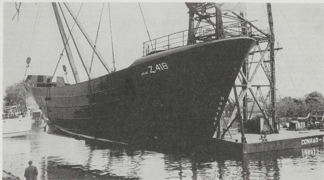
De Z.419 op het ogenblik van de tewaterlating. Men bemerkt de enorme hefkransen die het vaartuig neerlaten.
