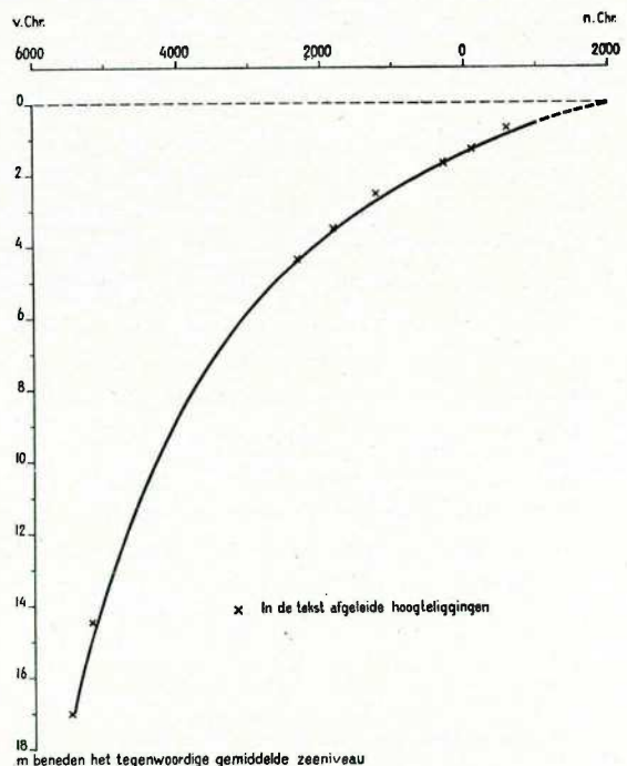
De zeespiegelstijging in West-Nederland na 6000 jaar v. Chr. naar Bennema 1954.
