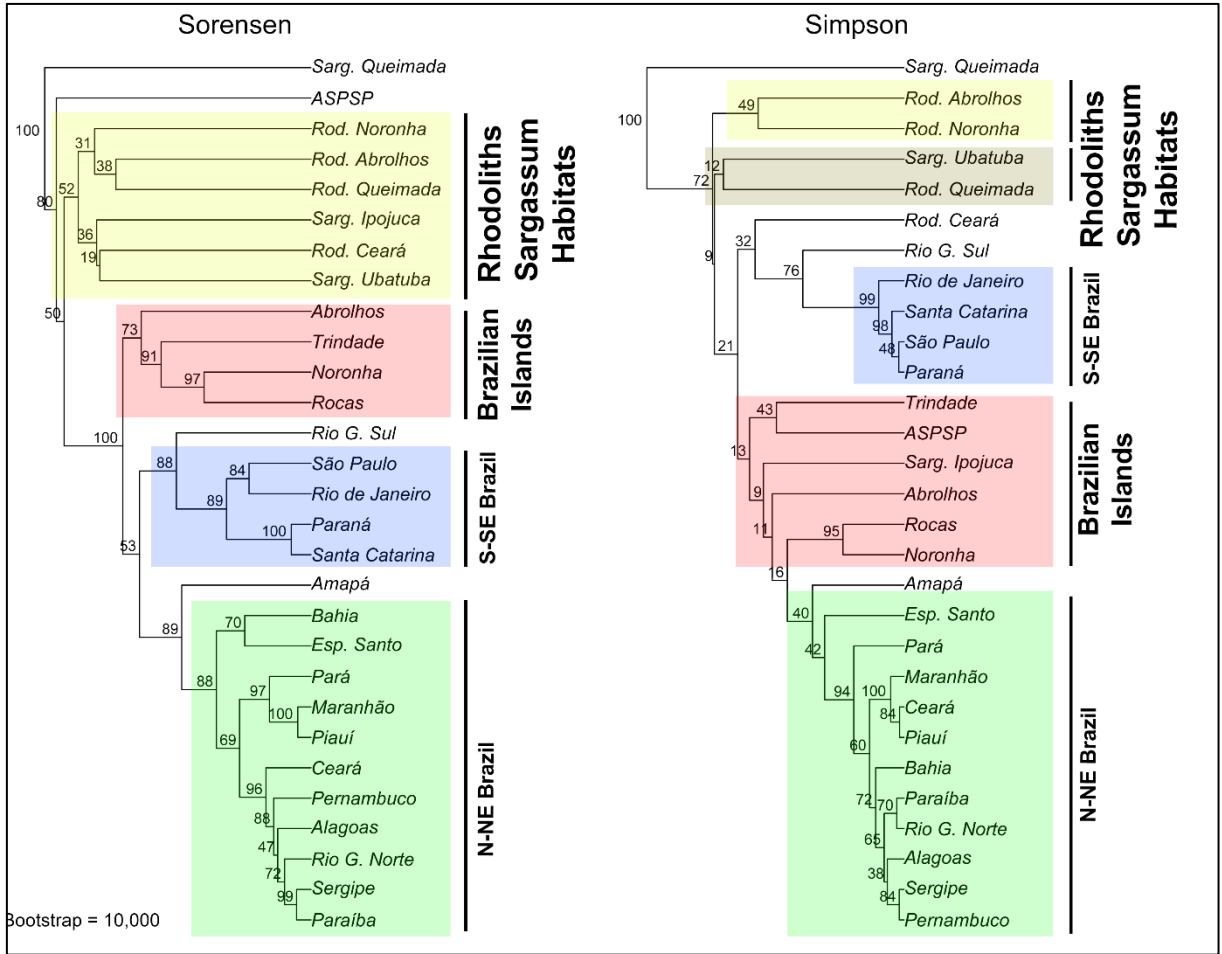
Figura 30. Dendrograma biogeográfico de Gastropoda
