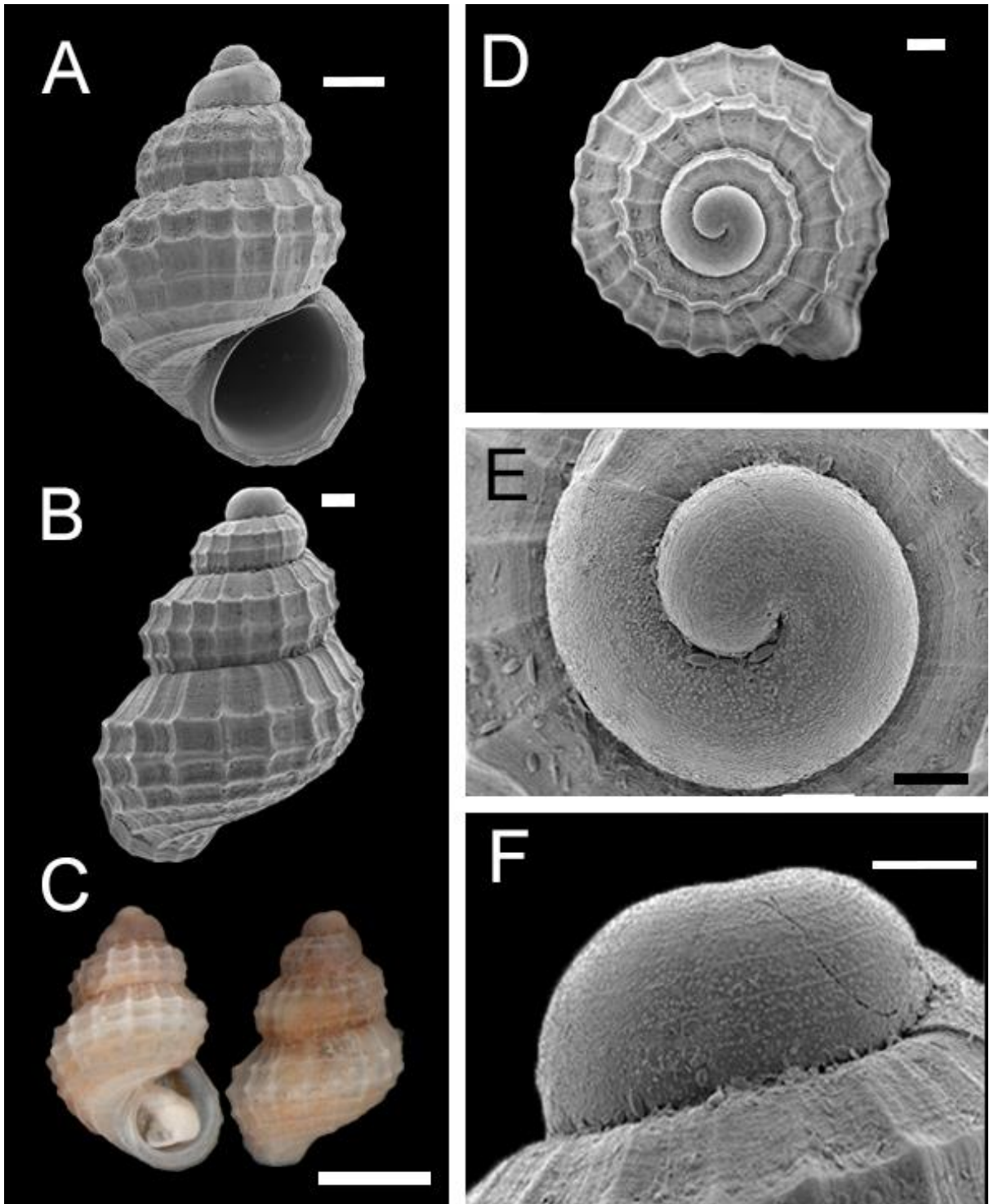
Figura 11. Alvania auberiana (Rissoidae). Eletromicrofotografia da (A) vista apertural, (B) vista abapertural, (C) aspecto conchiliológico da coloração do animal coletado e fixado em álcool 70% observada em estereomicroscópio, (D) vista apical para contagem do número de voltas, (E) detalhe observado na protoconcha do espécime com pústulas (F) detalhe da escultura espiral da protoconcha formando linhas multiseriadas. Escalas: A= 200 \mu m; B= 100 \mu m; C=500 \mu m; D= 100 \mu m; E-F= 50 \mu m.
