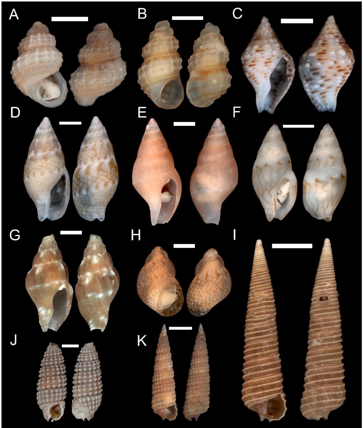
Figura 5. Fotomicrografias das espécies de gastrópodes associados aos rodólitos das três ilhas estudadas. (A) Rissoidae: Alvania auberiana , (B) Simulamerelina caribaea ; (C) Columbellidae: Columbela mercatoria , (D) Zafrona idalina , (E) Zafrona idalina (variação), (F) Astyris lunata , (G) Anachis fenneli ; (H) Phasianellidae: Eulithidium affine ; (I) Cerithiopsidae: Seila adamsii , (J) Cerithiopsis cf. gemmulosa , (K) Cerithiopsis flava . Escalas: A-B= 500 µm; C= 2000 µm; D-H= 1000 µm; I= 2000 µm; J= 500 µm; K= 1000 µm.
