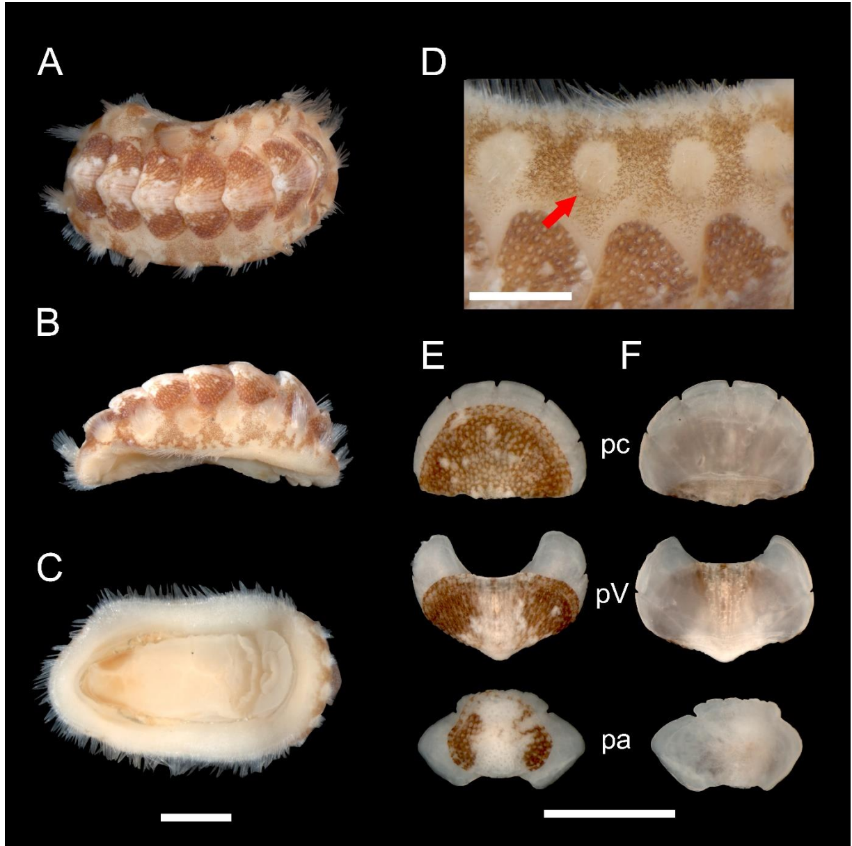
Figura 20. Acanthochitona sp. (Acanthochitonidae). (A) Vista dorsal do indivíduo íntegro, (B) vista lateral direita; (C) vista ventral, (D) detalhe dos tufos de espinhos no cinturão (seta), (E) vista dorsal das placas, (F) vista ventral das placas; placa cefálica (pc); placa intermediárias V (pV), placa anal (pa), boca (bo), cabeça (ca), brânquias (b), cinturão (c). Escalas: A-E= 1000 \mu m.
