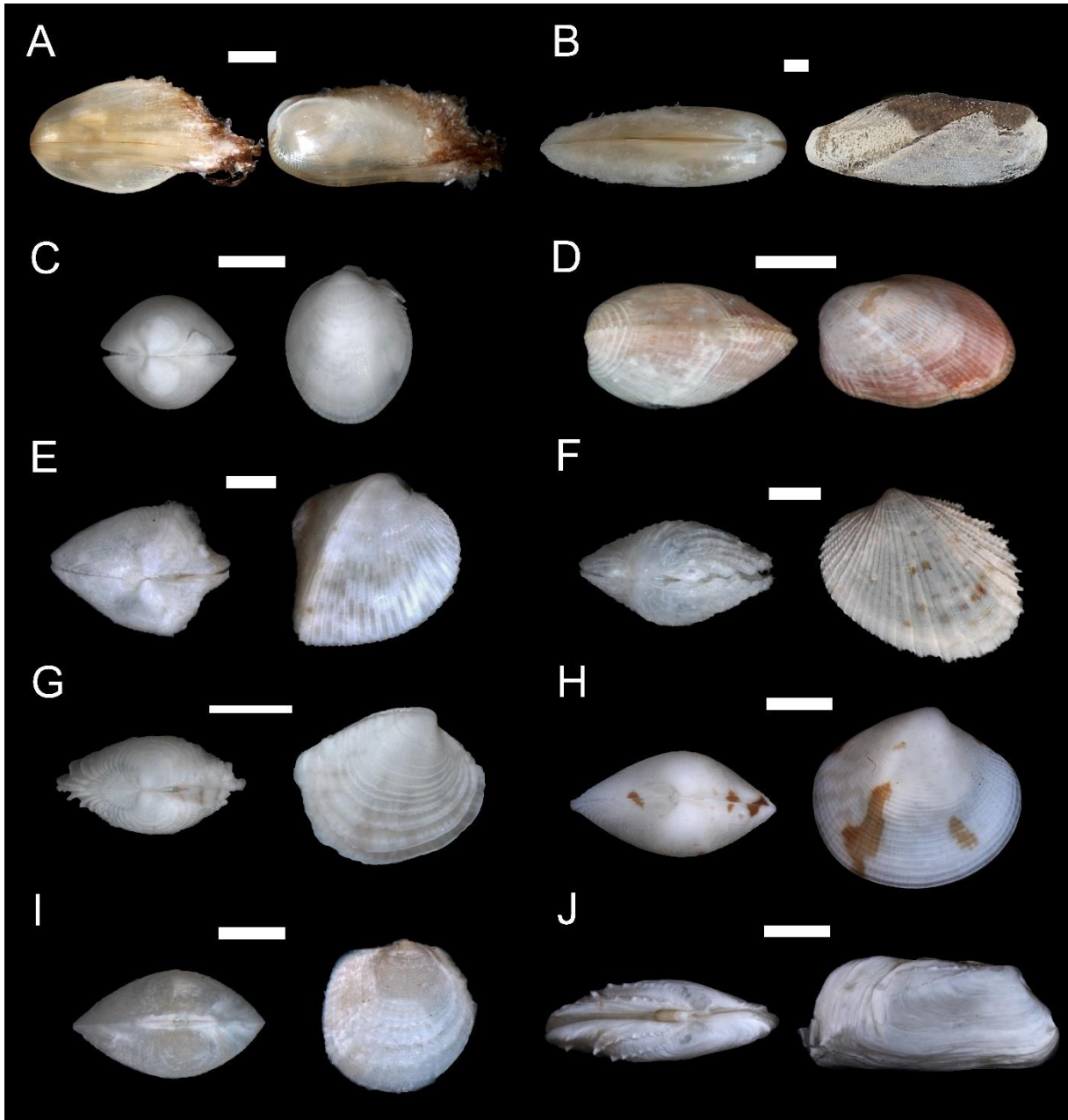
Figura 16. Fotomicrografias das espécies de Bivalvia associados aos rodolitos. (A) Mytilidae: Gregariella sp., (B) Leiosolenus bisulcatus , (C) Crenella decussata , (D) Musculus laterallis ; (E) Cardiidae: Americardia media , (F) Papyridea semisulcata ; (G) Veneriidae: Chioninae, (H) Gouldia cerina ; (I) Limopsidae: Limopsidae 1; (J) Lyonsiidae: Entodesma sp. Escalas: A-D = 1000 \mu m; E-F = 500 \mu m; G-H = 1000 \mu m; I = 500 \mu m; J = 1000 \mu m.
