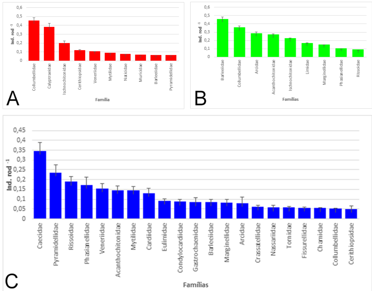
Figura 29. Assembleias de moluscos em (A) Queimada Grande (B) Fernando de Noronha e (C) Arquipélago de Abrolhos encontradas a partir dos resultados da MRT baseado na dominância de cada uma das Famílias encontradas.
