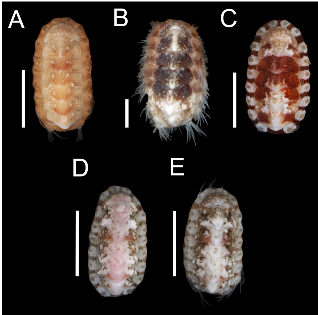
Figura 19. Variação policromática em A. terezae com as 5 variações encontradas associadas aos rodolitos. Escala A-E: 1000 \mu m.
