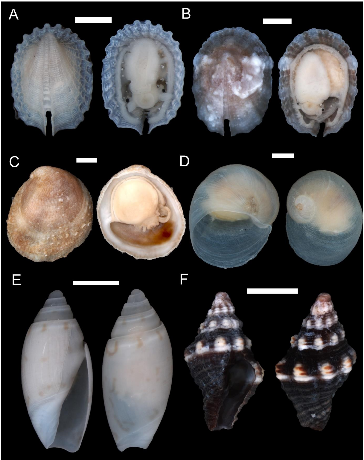
Figura 9. Fotomicrografias das espécies de gastrópodes associados aos rodólitos das três ilhas estudadas. (A) Fissurellidae: Emarginula sp. 1, (B) Emarginula sp. 2; (C) Calyptraeidae: Bostrycapulus aculeatus ; (D) Naticidae: Sinum perspectivum ; (E) Olividae: Olivella nivea ; (F) Pisaniidae: Engina turbinella . Escalas: A= 500 µm B= 1000 µm; C= 2000 µm; D= 500 µm; E= 1000 µm; F= 2000 µm.
