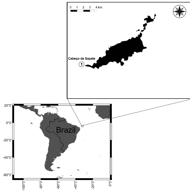
Figura 1. Localização do Arquipélago de Fernando de Noronha no Atlântico Sul (modificada de Matheus et al. , 2019).
