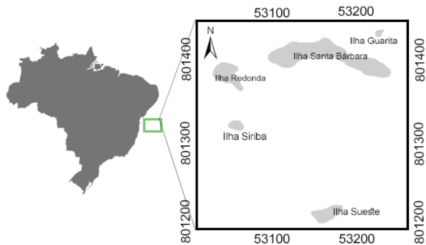
Figura 2. Localização do Arquipélago de Abrolhos no Atlântico Sul e suas cinco ilhas (modificada de Schaefer et al. 2006).
