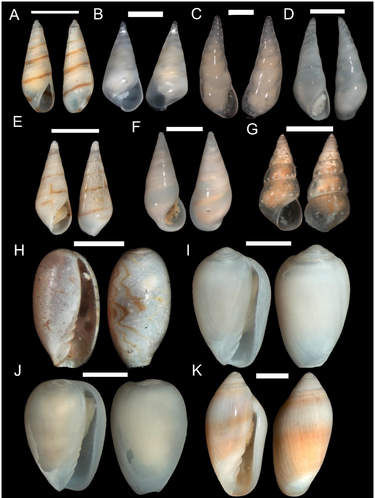
Figura 7. Fotomicrografias das espécies de gastrópodes associados aos rodólitos das três ilhas estudadas. (A) Eulimidae: Hemiliostraca auricincta , (B) Melanella sp., (C) Vitreollina sp. 1, (D) Vitreollina sp. 2, (E) Eulima fulvocincta ; (F) Zebinidae: Zebina sp.; (G) Litiopidae: Alaba incerta ; (H) Marginellidae: Marginellidae 1, (I) Marginellidae 2, (J) Marginellidae 3, (K) Volvarina albolineata . Escalas: A = 500 \mu m; B = 1000 \mu m; C-K = 500 \mu m.
