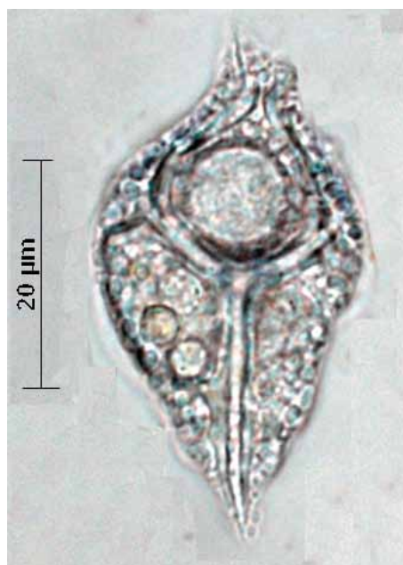
Fig. 7. LM of Hermesinum adriaticum
