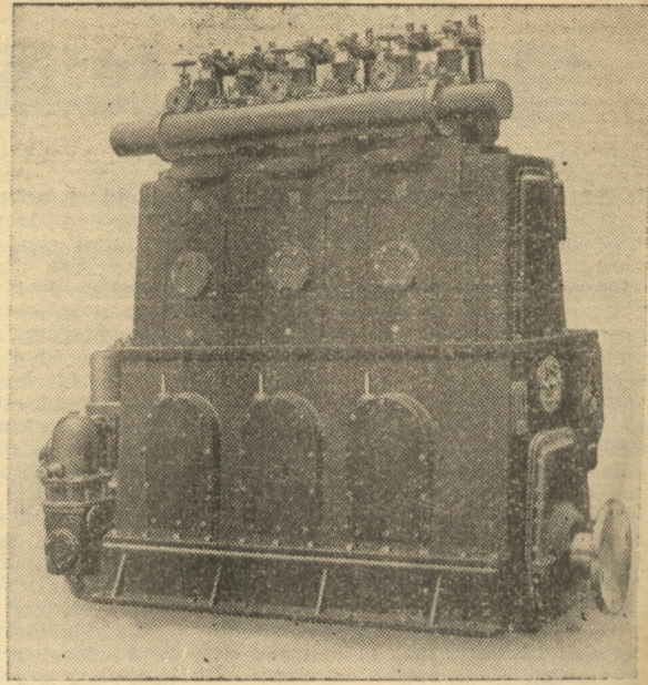
Scheepsdieselmotor 3 cyl. 4 toeren
