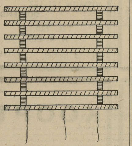
Ligging der kaders met een tussenruimte van minstens 10 cm, voor de oesters en van minstens 20 cm, voor de mosselen.
