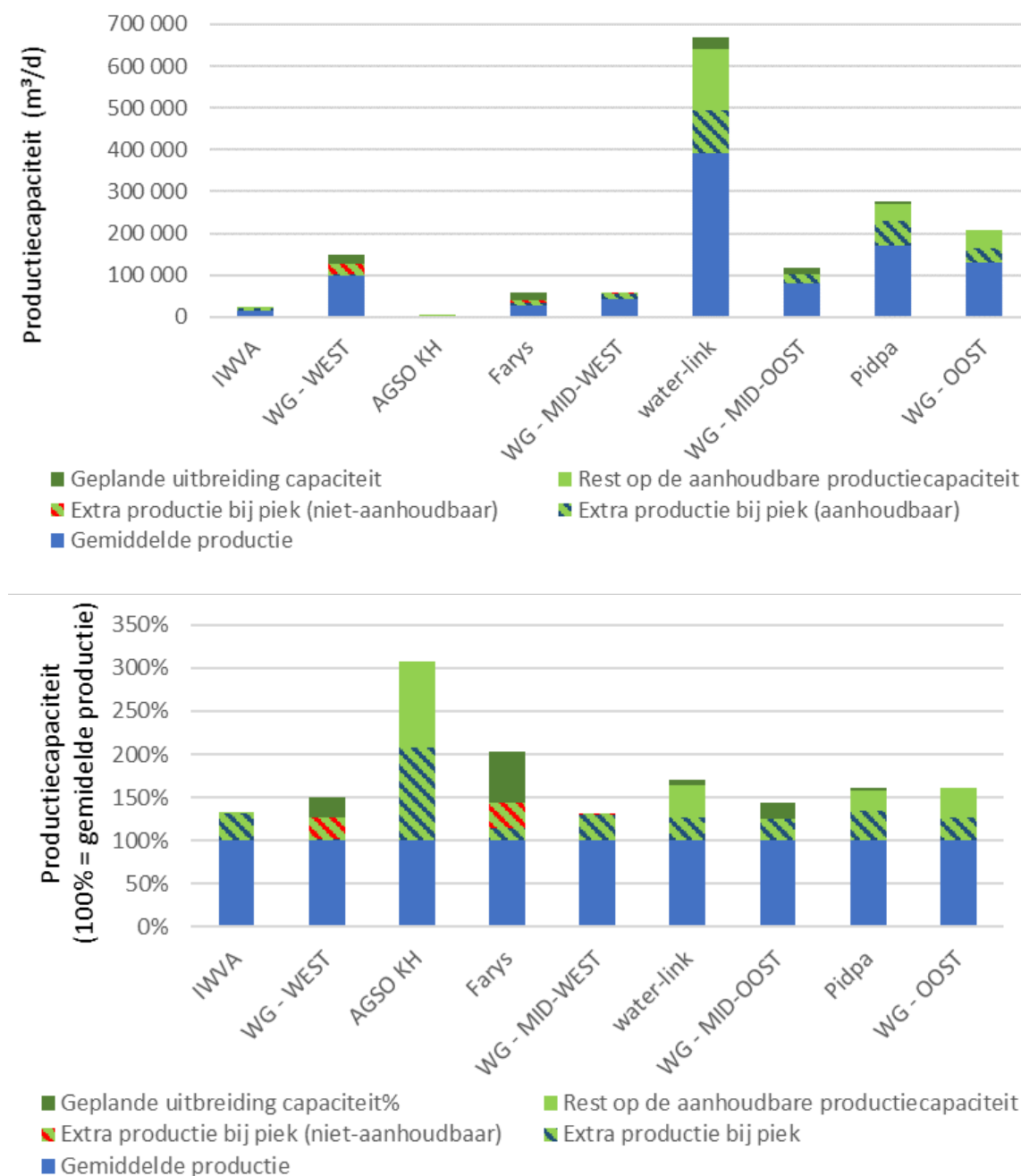
Figuur C: de maximale productiecapaciteit opgedeeld in gemiddelde productie, aanhoudbare productie, niet-aanhoudbare productie en resterende capaciteit met daarbovenop de geplande goedgekeurde uitbreidingen (bovenaan in absolute cijfers, onderaan in relatieve cijfers)
