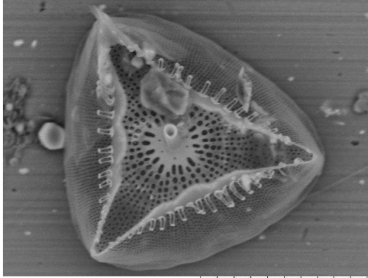
Ditylum sp. (SEM, valve view, x2.5, 30 \mu m scale)
