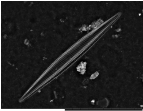
Nitzschia sp. (SEM, valve view, x1.8k, 50 µm scale)
