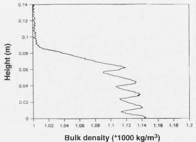
Figuur 4: Densiteitsprofiel van een mengsel met Scheldeslib 3 en 41% zand.
