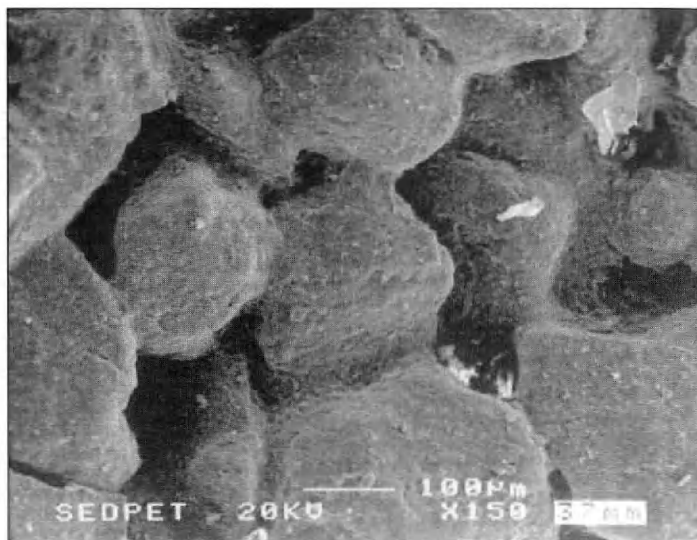
Foto 4: Een cohesief kaolinetmengsel met een slibgehalte van 15%.
