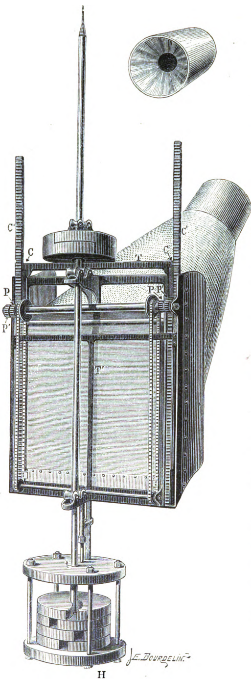
Fig. 31. Courtinen-Schliessnetz geschlossen, an die Oberfläche steigend. Oben das losgelöste Sammelgefäß von der Oeffnung aus gesehen, um die zum Zurückhalten der gefangenen Thiere bestimmte Falle aus Seidengaze zu zeigen.
