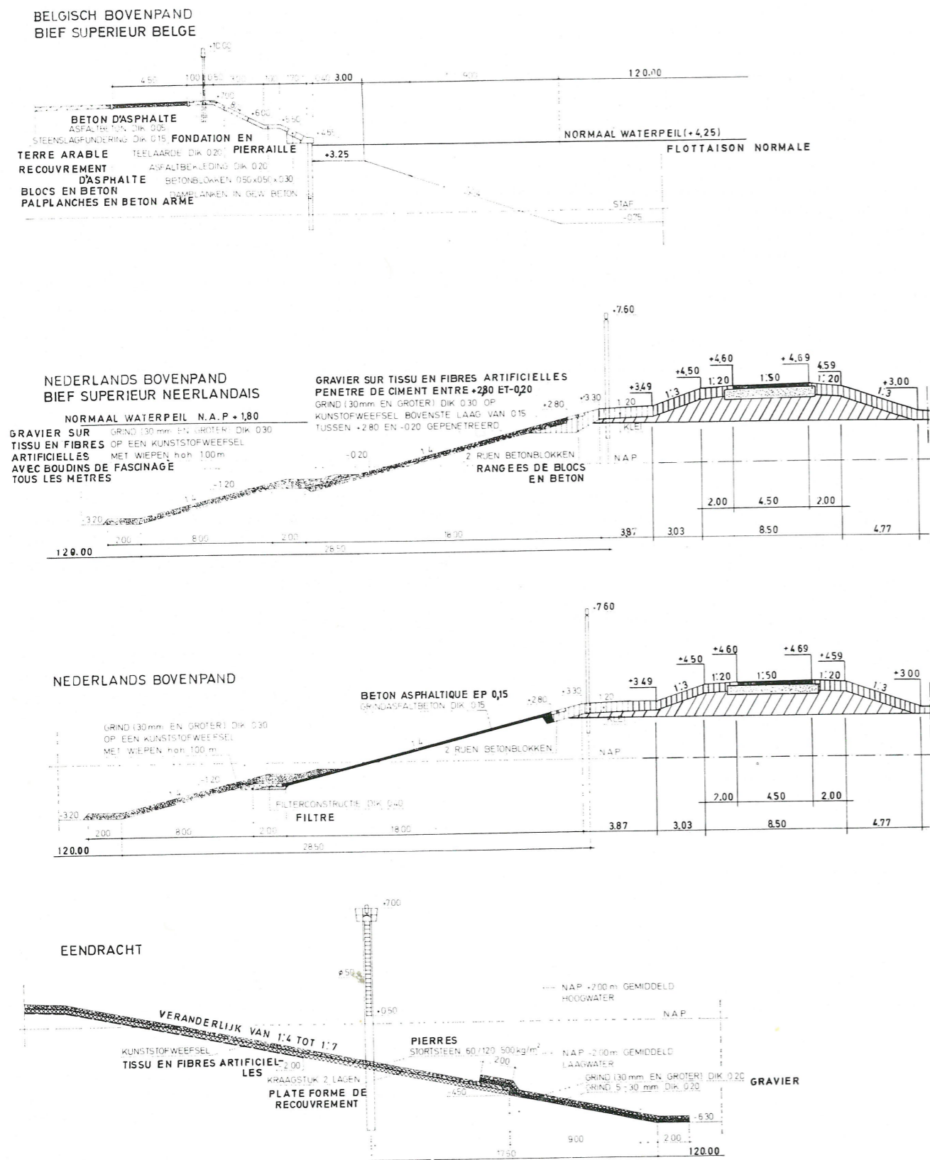
Fig. 4. — Consolidations de talus.
