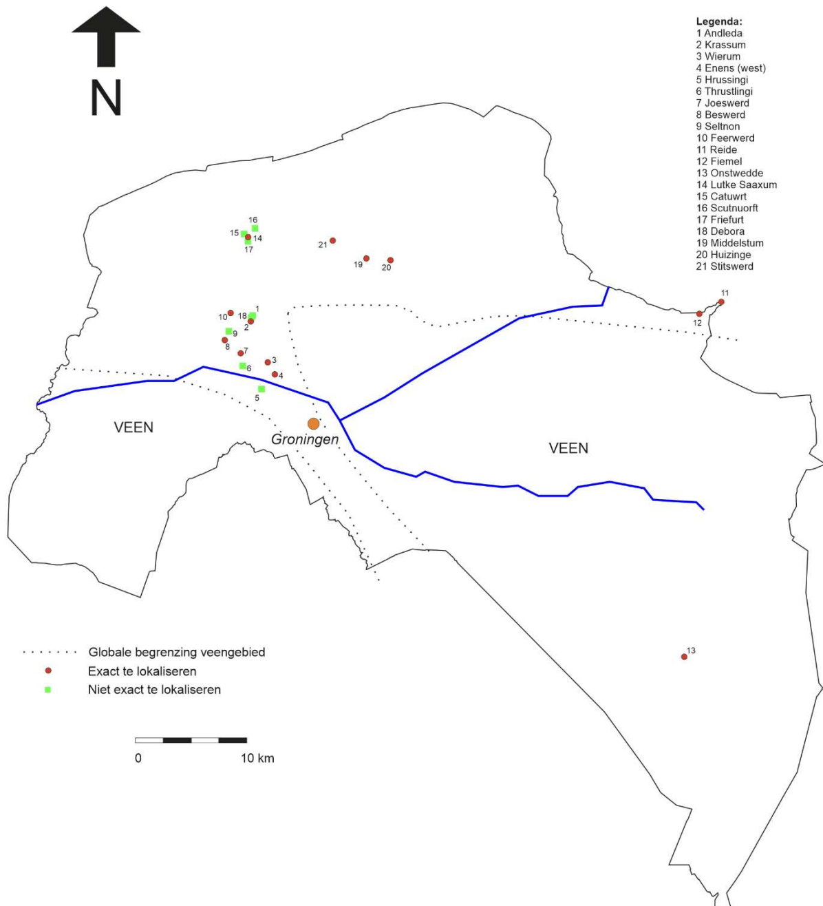
Figuur 3.10 Locaties van de Groninger toponiemen, genoemd in de goederenlijsten van Fulda en Werden uit de periode 800-900, die exact of bij benadering te lokaliseren zijn.
