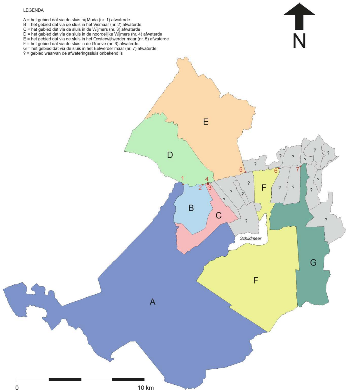
Figuur 6.2 De afwateringseenheden in het Generale zijlvest der Drie Delfzijen in 1470.
