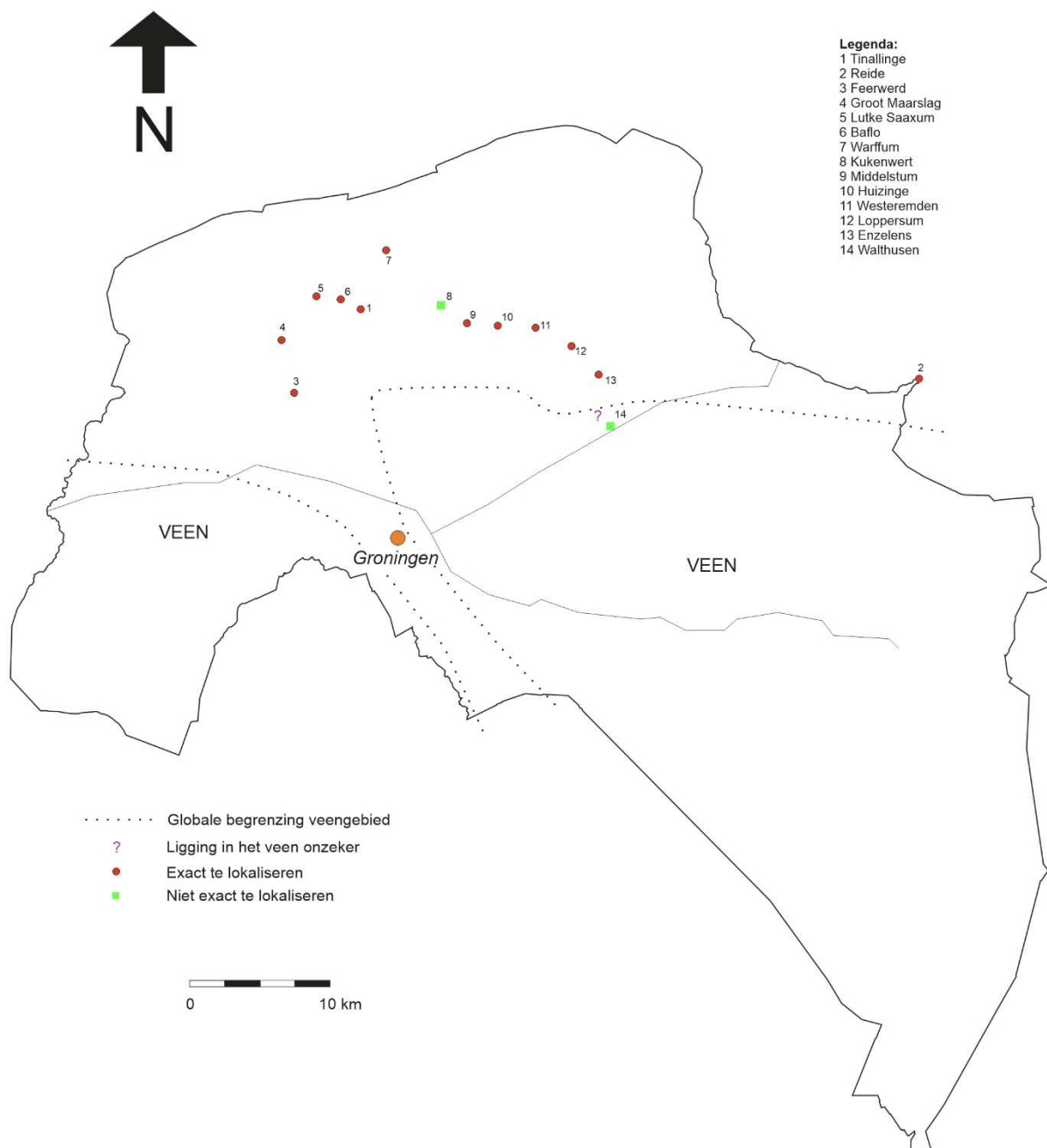
Figuur 3.11 Locaties van de Groninger toponiemen, genoemd in de goederenlijsten van Fulda en Werden uit de periode 900-975, die exact of bij benadering te lokaliseren zijn.
