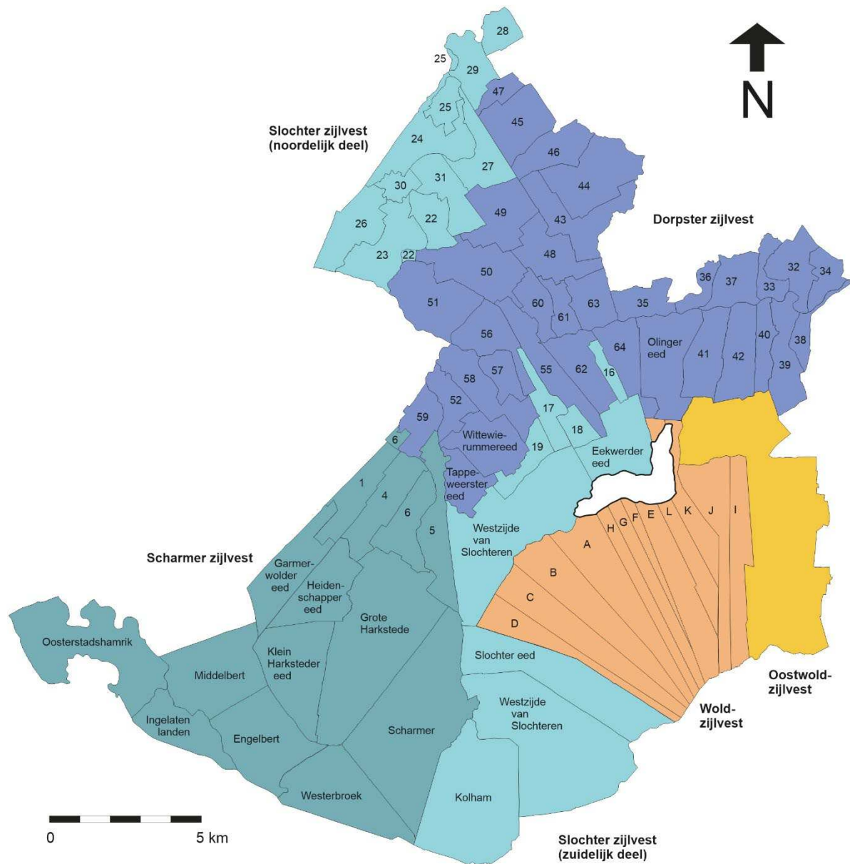
Figuur 5.2 Het Generale zijlvest der Drie Delfzijlen, het Woldzijlvest en het Oostwoldzijlvest rond 1750 (naar Siemens 1954). De letter- en cijferaanduidingen komen overeen met die in de tabellen 5.1 en 5.2.
