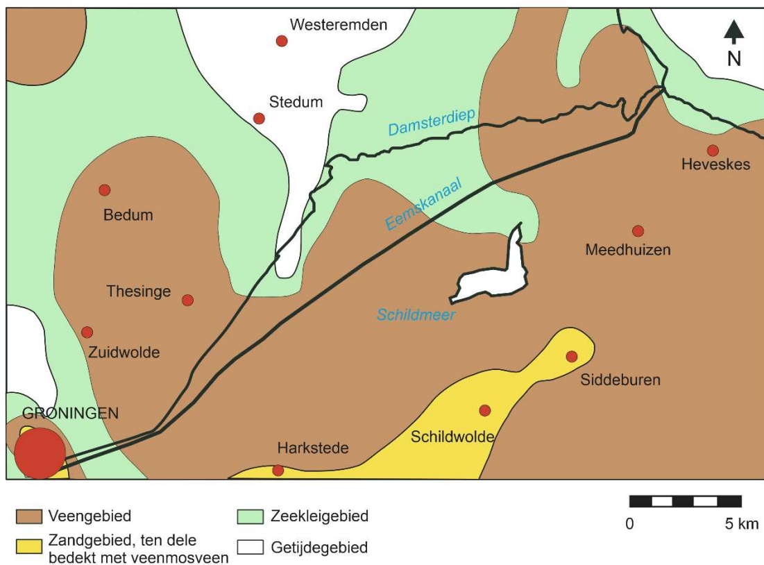
Figuur 2.7 Paleogeografische kaart van het onderzoeksgebied en nabije omgeving van omstreeks 2600 BP (naar Roeleveld 1974, 106).
