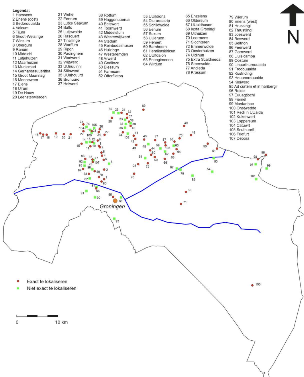
Figuur 3.9 Locaties van de Groninger toponiemen, genoemd in de goederenlijsten van Fulda en Werden uit de periode 800-1050, die exact of bij benadering te lokaliseren zijn.
