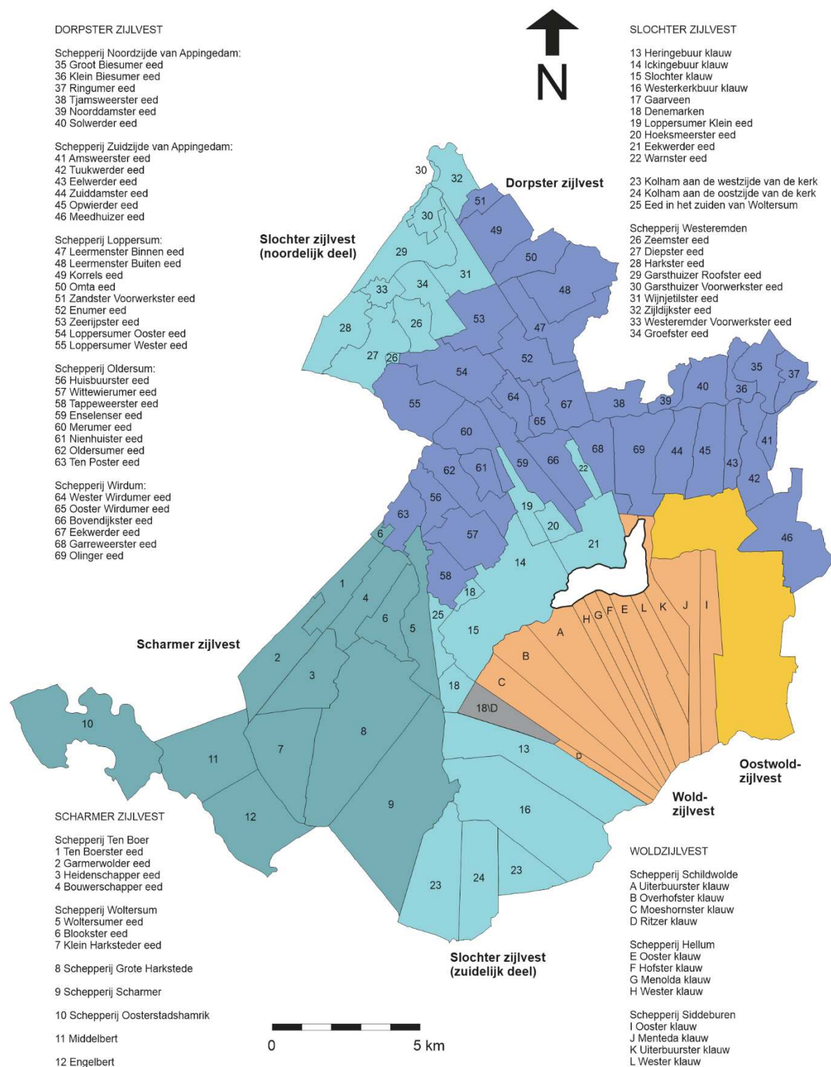
Figuur 5.3 Het Generale zijlvest der Drie Delfzijen, het Woldzijlvest en het Oostwoldzijlvest rond 1470.
