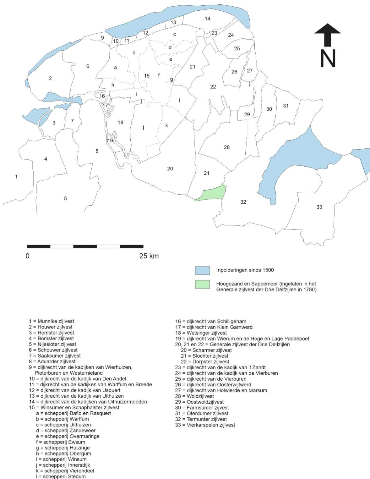
Figuur 5.1 De zijlvesten en dijkrechten in Groningen rond 1750 (naar Siemens 1955, Siemens 1962 en Siemens 1974).
