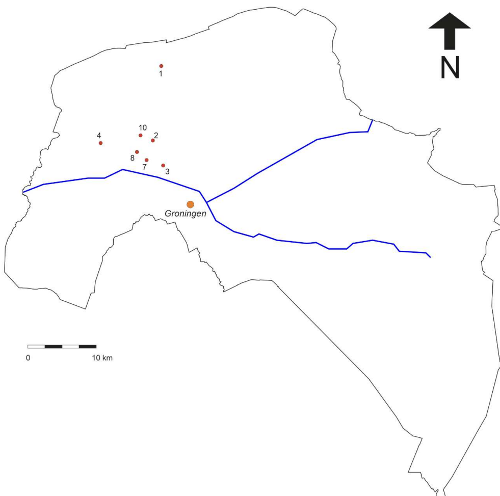
Figuur 3.5 De locaties van toponiemen in de huidige provincie Groningen, genoemd in een goederenlijst van de abdij Werden uit omstreeks of kort na 890 (bijlage 1, nr. 12), die door Künzel e.a. (1989) exact gelokaliseerd zijn. De nummers corresponderen met die in tabel 3.4. Niet afgebeeld zijn de nrs. 5, 6 en 9.
