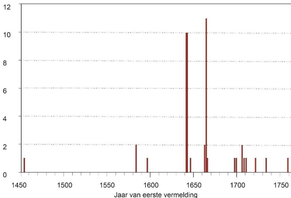
Figuur 6.5 Histogram van de eerste vermeldingen van watermolens in Groningen in de periode 1450-1765.
