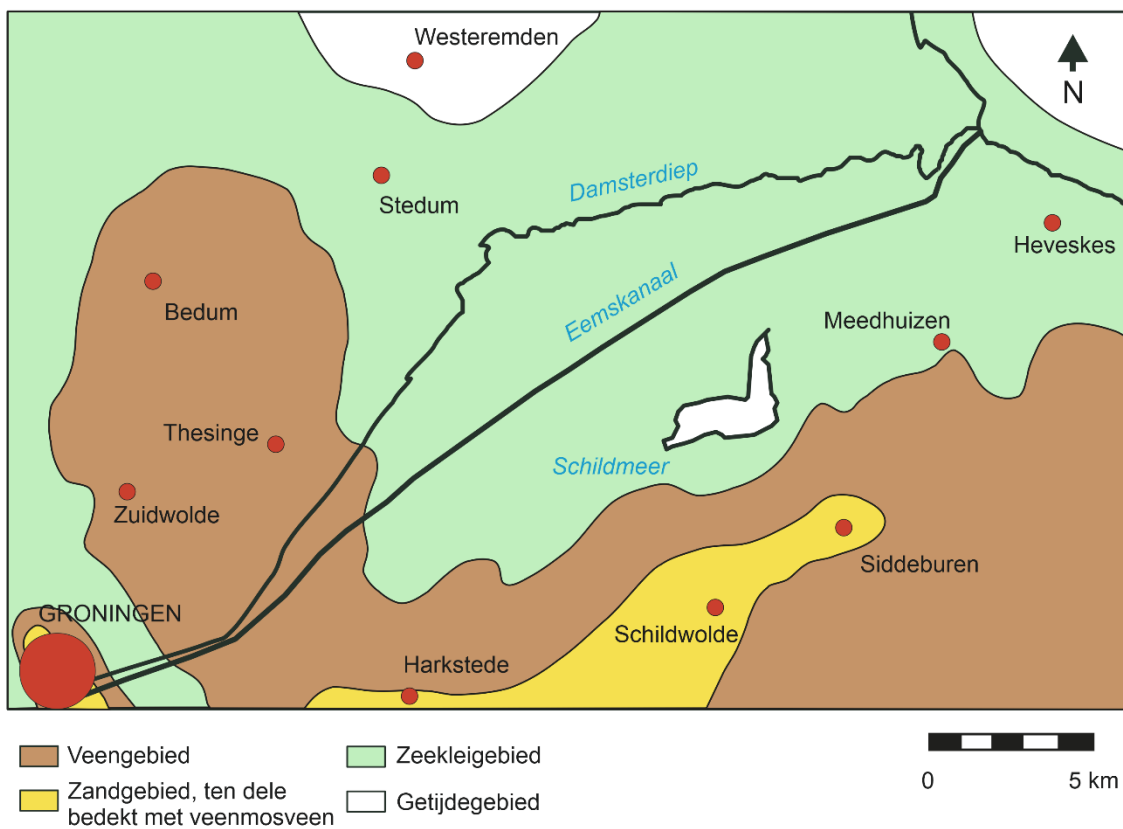
Figuur 2.8 Paleogeografische kaart van het onderzoeksgebied en nabije omgeving van omstreeks 2000 BP (naar Roeleveld 1974, 110).
