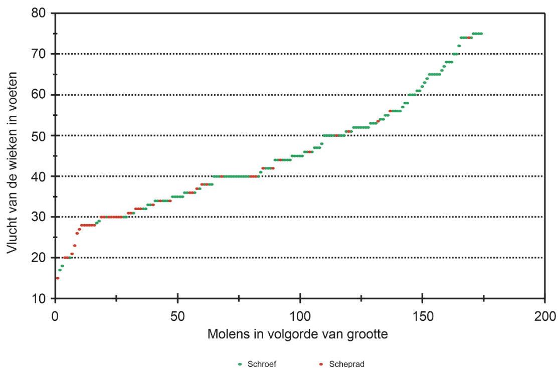
Figuur 7.2 De vlucht van de windwatermolens in en bij de Wolden in december 1811, weergegeven in volgorde van grootte.
