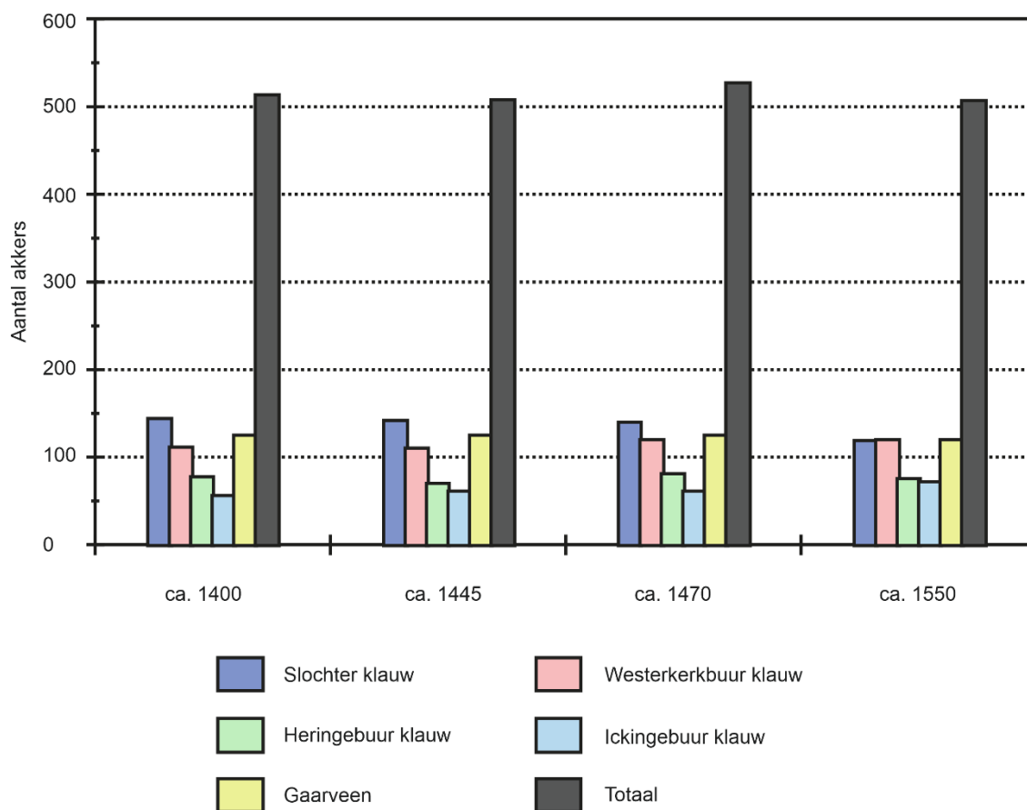
Figuur 6.7 Het aantal akkers in vijf klauwen van het Slochter zijvest gedurende de periode ca. 1400-ca. 1550.
