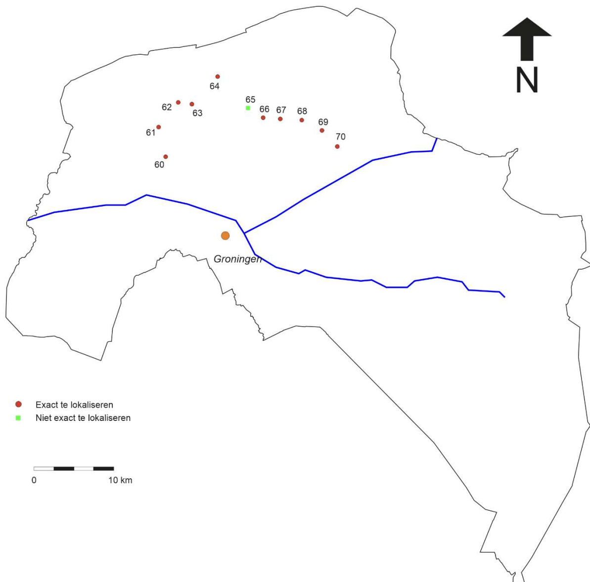
Figuur 3.8 De locaties van toponiemen in de huidige provincie Groningen, genoemd in een goederenlijst van de abdij Werden uit 944 (bijlage 1, nr. 14), die door Künzel e.a. (1989) exact gelokaliseerd zijn, alsmede de (niet exact aan te geven) locatie van Kukenwert.
