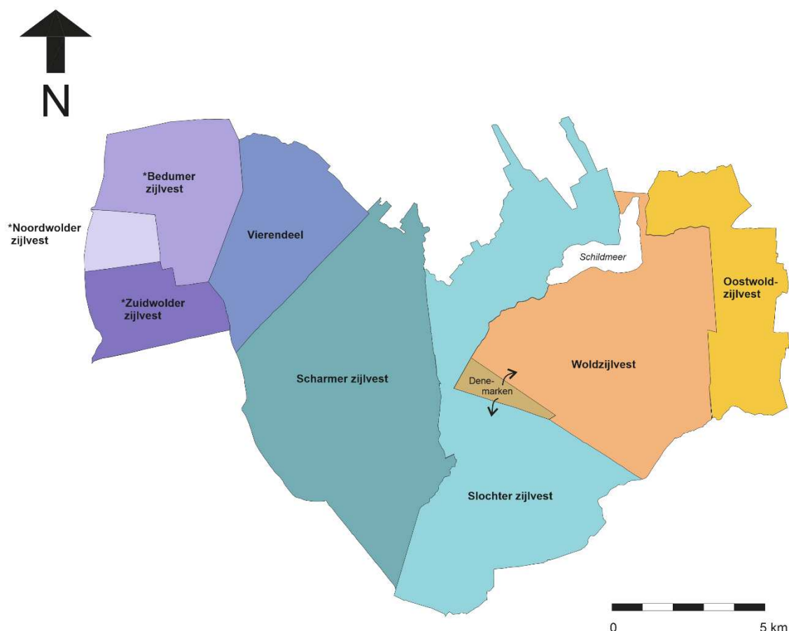
Figuur 5.7 De vermoedelijke grenzen van de Acht zijlvesten in het vierde kwart van de 14e eeuw. In het Winsumer zijlvest is slechts éénmaal een gebied ingelaten, en wel het kerspel Noorddijk in het jaar 1408 (zie noot 251).
