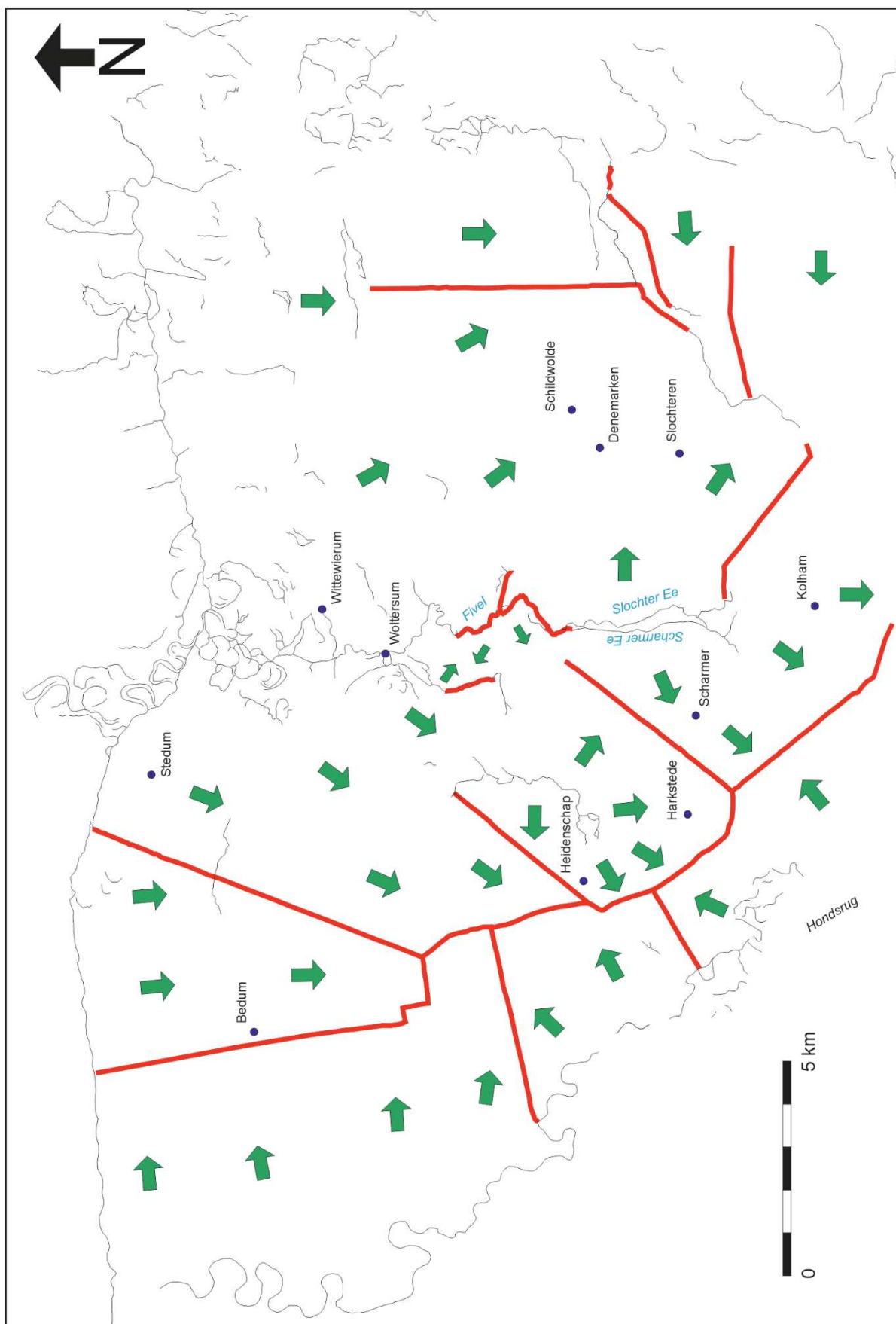
Figuur 4.3 Reconstructie van de ontginningsrichting in de diverse delen van het onderzoeksgebied en zuidoost Hunsingo aan de hand van figuur 4.1, alsmede het geheel van lijnen waar kavelcomplexen op elkaar stoten.
