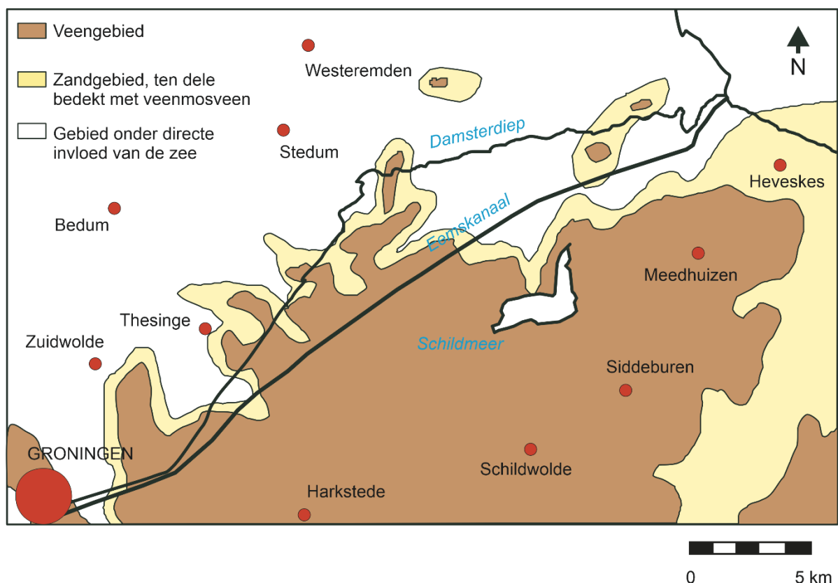
Figuur 2.2 Paleogeografische kaart van het onderzoeksgebied en nabije omgeving van omstreeks 5400 BP (naar Roeleveld 1974, 97).
