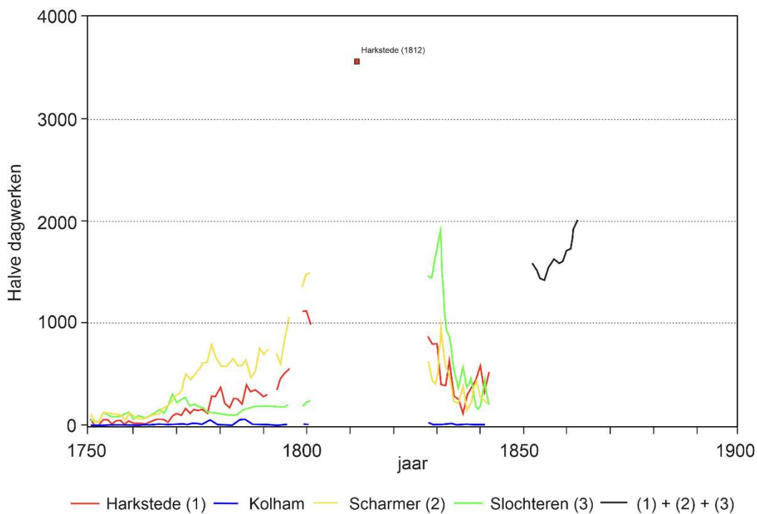
Figuur 7.6 De hoeveelheden gewonnen turf in de (voormalige) kerspelen Harkstede, Kolham en Scharmer en in de gemeente Slochteren gedurende de periode 1750-1900.
