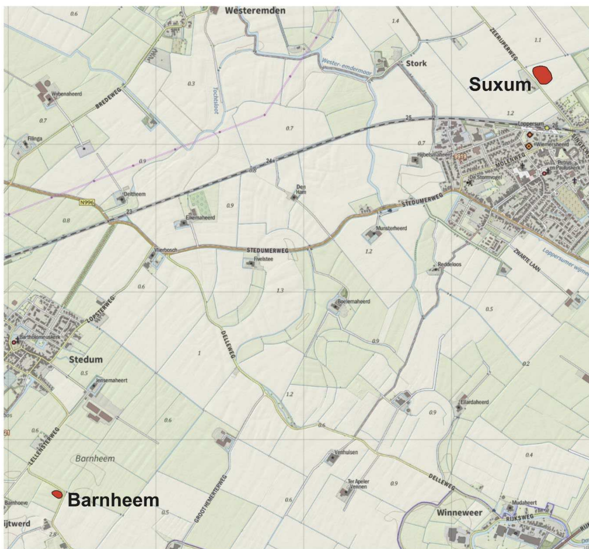
Figuur 3.3 Uitsnede van de topografische kaart van Nederland met daarop aangegeven de terpen Barnheem en Suxum.
