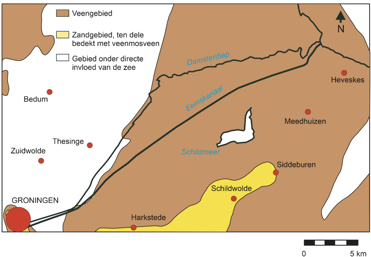
Figuur 2.6 Paleogeografische kaart van het onderzoeksgebied en nabije omgeving van omstreeks 3200 BP (naar Roeleveld 1974, 103).
