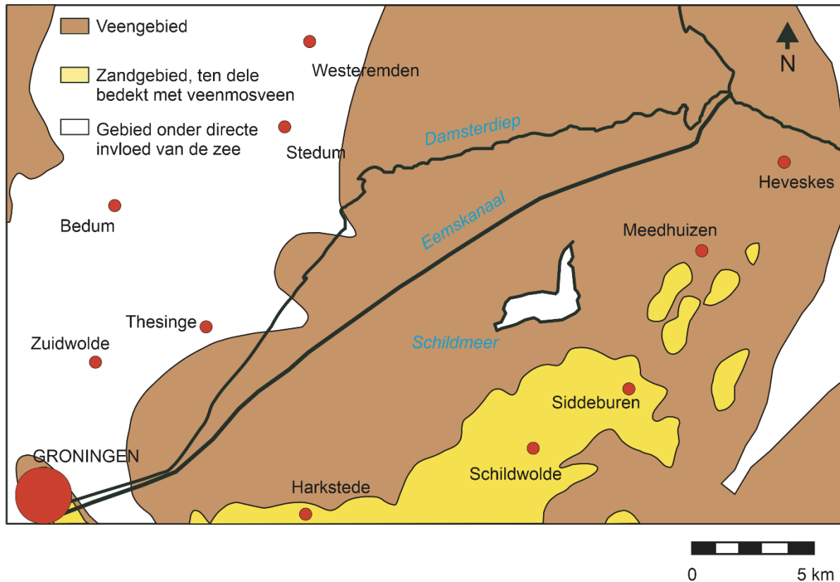
Figuur 2.4 Paleogeografische kaart van het onderzoeksgebied en nabije omgeving van omstreeks 3650 BP (naar Roeleveld 1974, 99).
