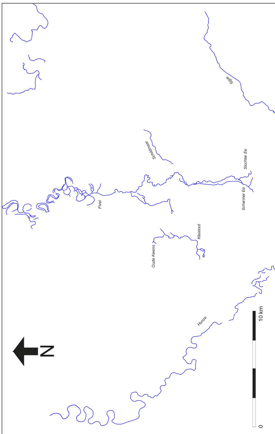
Figuur 6.1 Reconstructie van het natuurlijk afwateringspatroon vlak vóór het begin van de ontginningen.
