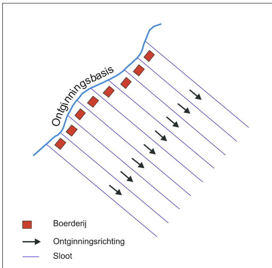
Figuur 1.6 Schematische voorstelling van de ontginning van een veengebied.
