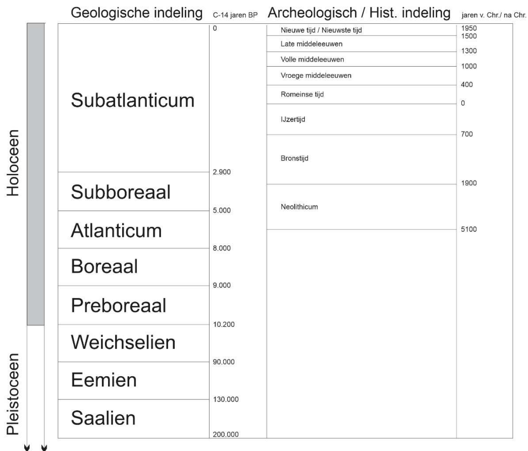
Figuur 2.1 Geologische en archeologisch/historische tijdschaal (naar Koster 1980). De dikte van de balken is niet indicatief voor de duur van de verschillende perioden. Over de exacte tijdsgrenzen van de perioden binnen de middeleeuwen bestaan vele opvattingen (De Boer e.a. 1989, 13-21). Om praktische redenen zijn hier, en vanzelfsprekend ook in de tekst, de jaren 400, 1000, 1300 en 1500 als cesuren gekozen.
