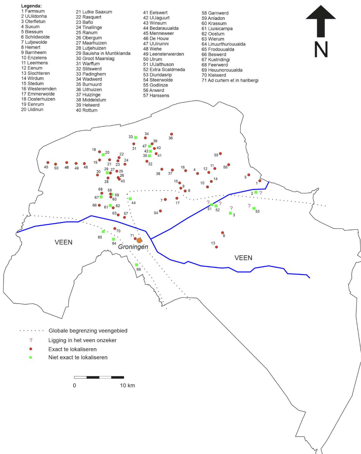
Figuur 3.14 Locaties van de Groninger toponiemen, genoemd in de goederenlijsten van Fulda en Werden uit de periode 1025-1050, die exact of bij benadering te lokaliseren zijn.
