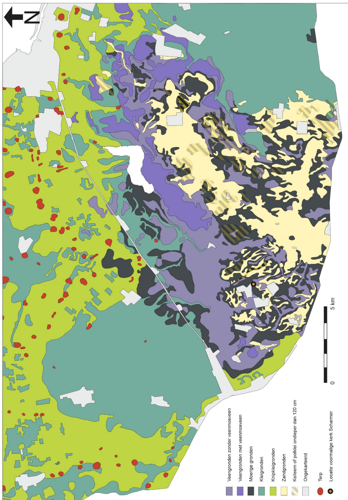
Figuur 1.4 Vereenvoudigde bodemkaart van de Wolden en omgeving (naar Stiboka 1973 en Stiboka 1986).
