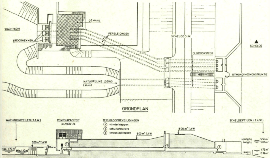
Doorsnede pompgemaal - polder Grebergen
