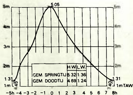
Gemiddelde tij-kromme te Dendermonde
