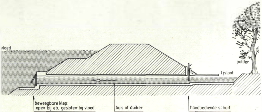
Schema uitwateringssluis
