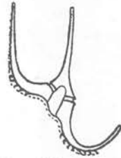
Fig. 136. C. horridum Gran X 150.
