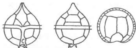
Fig. 123. P. pellucidum (Bergh). Ventral, dorsal and antapical views. X 400.
