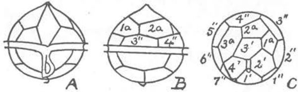
Fig. 111. P. subpunctulatum Wailes. A, ventral; B, dorsal; C, apical view. X 400.
