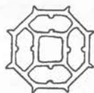
Fig. 22. D. octangulatus Wailes X 450.
