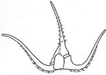
Fig. 135. C. longipes (Bailey) X 150.
