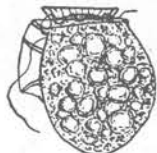
Fig. 66. D. lenticulata Pavillard X 400.
