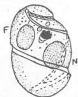
Fig. 30. Pou-chetia maxima K. & S. X 250. F, a food particle; N, nucleus.
