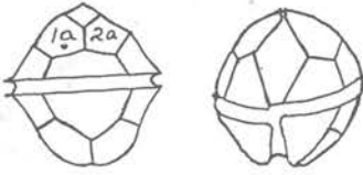
Fig. 92. P. avellana Meunier X 400.
