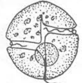
Fig. 41. G. flavum K. & S. X 1000.
