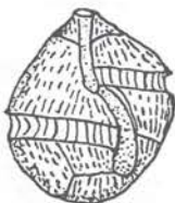
Fig. 78. G. scrippsae Kofoid X 600.
