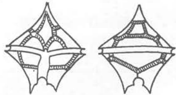
Fig. 114. P. divergens Ehrenb. X 300.
