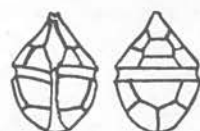
Fig. 102. P. trochoideum (Stein) X 550.
