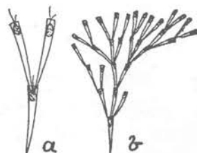
Fig. 17. Dinobryon balticum Schütt. A, X 125; B, X 75.
