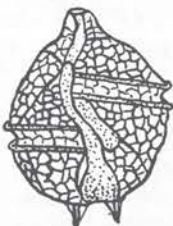
Fig. 80. G. digitale (Pouchet) X 500.
