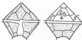
Fig. 108. P. obtusum Karsten; X 350.
