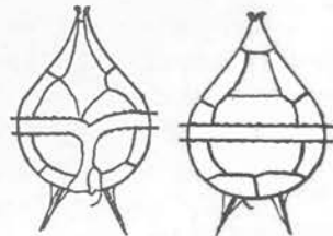
Fig. 118. P. micrapium Meunier X 500.
