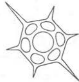
Fig. 19. Distephanus speculum (Ehrenb.) X 500.
