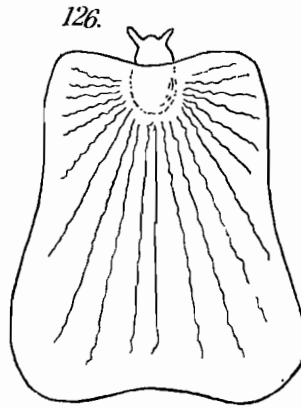
Fig. 125. Placobranchus guttatus STIMPSON Fig. 126. — Allure de Placobranchus guttatus avec les lobes plissés étalés
