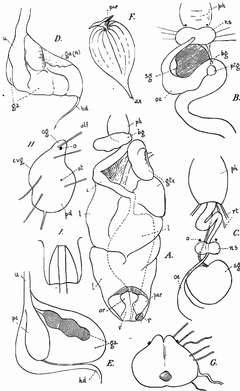
Fig. 6. Dendrodoris elongata BABA. — a. Ensemble des organes, r, papille rénale \times 22 ; b. Partie antérieure du tube digestif \times 3,3 environ (la glande sanguine est enlevée); c. Partie antérieure du tube digestif avec œsophage rejeté en arrière, sg, glande ptyaline; d. Ensemble des conduits génitaux et des glandes annexes en vue dorsale; e. Les mêmes, schématisés, avec le canal hermaphrodite un peu rejeté vers la gauche; f. Papille rénale, ax, orifice rénal externe \times 20 ; g. Système nerveux central, face dorsale \times 10 ; h. Le même, face droite; i. Disposition schématique de la trompe et de l'œsophage.
