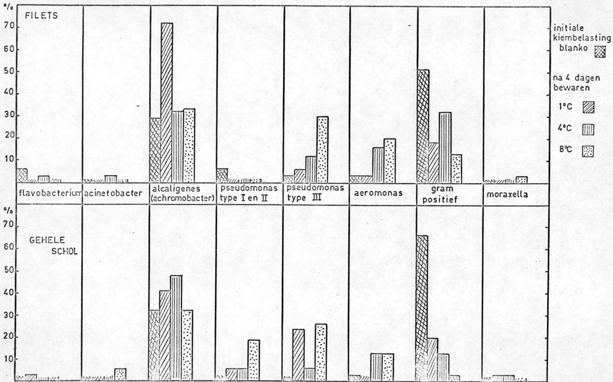
Fig. 4 - Differentiatieschema van de mikroflora aanwezig op voorverpakte schol bij de aanvang en op het einde van de proefperiode.
