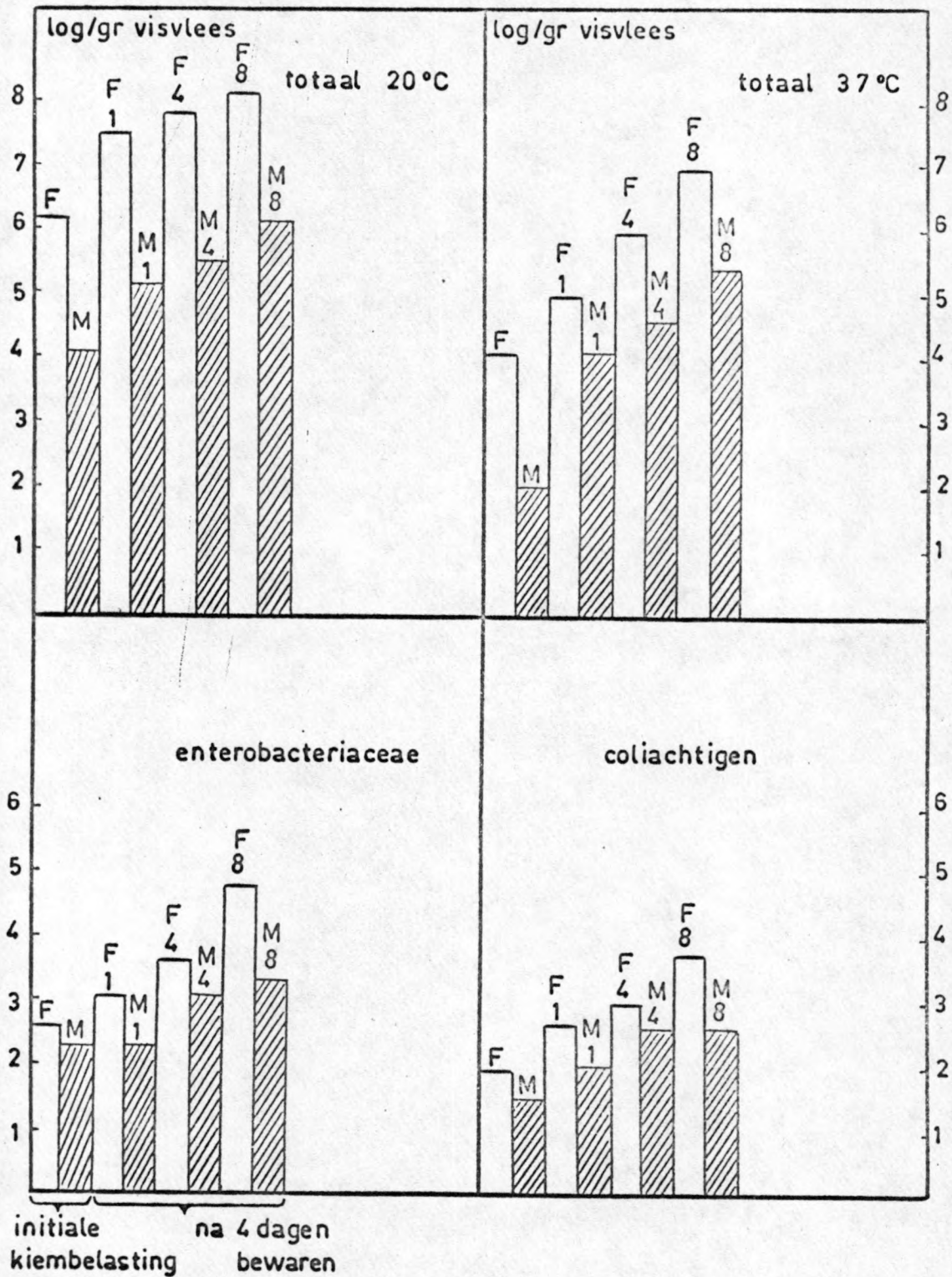
Fig. 5 - Resultaten van de tellingen van de aërobe bak erieën (inkubatietemperatuur 20° en 37°C), de Enterobacteriaceae en de coli-achtigen aanwezig op de voorverpakte gehele (M) en gefilleerde (F) na 0 en na 4 dagen onder koelwijze A (1), B (4) en C (8).
