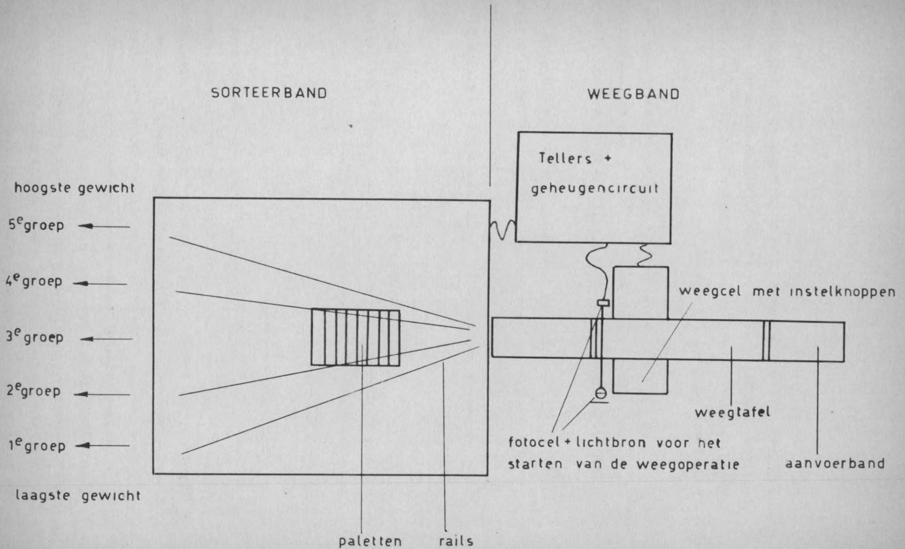
FIGUUR 1 Schematische voorstelling van de trieerinstallatie CL 500 - W - 5
