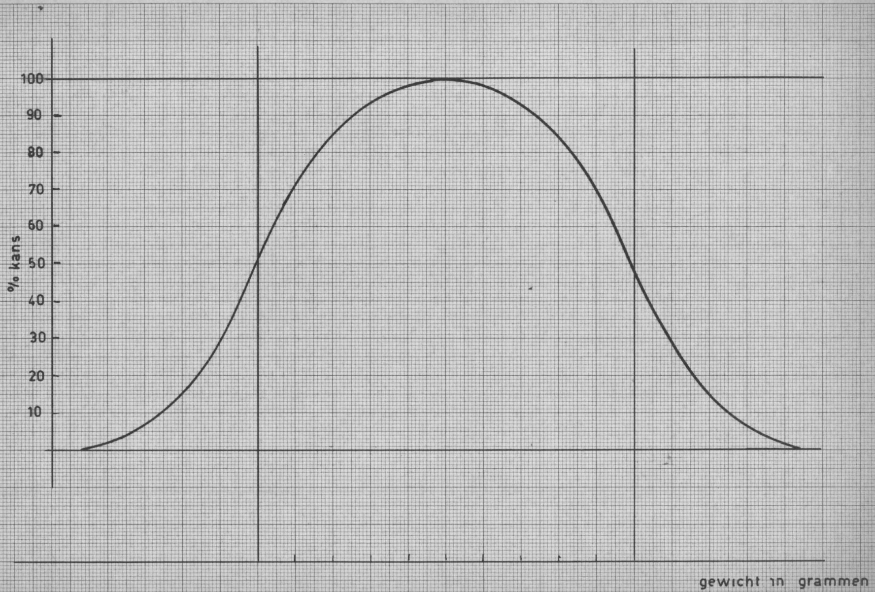
FIGUUR 6 GEWICHTSFREKWENTIE VERDELING BIJ HET NAT WEGEN - KLASSEBREEDTE 10g
