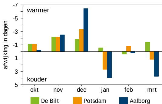
Figuur 3.4. Weersomstandigheden in Noord- en Oost-Europa in 2020/21, afgeleid uit het aantal vorstdagen (min. temperatuur < 0 °C) in Aalborg (Jutland, Denemarken) en Potsdam (Brandenburg, Duitsland). Weergegeven is de afwijking in dagen ten opzichte van de waarde in 2000/01-2019/20. Ter vergelijking is ook de situatie in De Bilt NL weergegeven. / Weather characteristics in northern (Aalborg, Denmark) and eastern (Potsdam, eastern Germany) Europe in 2019/20. Shown is the number of days with minimum temperatures below zero, expressed as the deviation in days from averages in 2000/01-2019/20. The Netherlands (De Bilt) is shown for comparison. Bron / data courtesy: DWD (Potsdam) and NOAA (Aalborg).
