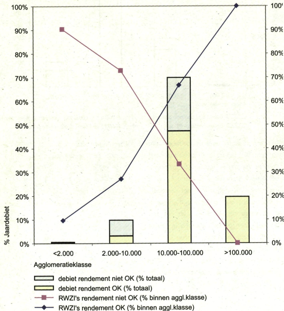
Figuur 27 - globale toetsing van de RWZI-effluenten aan de doelstelling voor het zuiveringsrendement voor fosfor (min. 70%)
