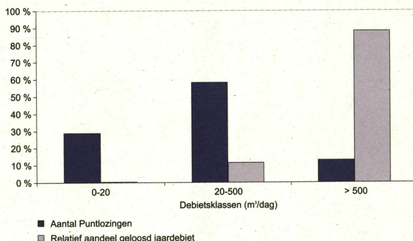
Figuur 10 - lozingsprofiel van de bemonsterde puntlozingen in 2003
