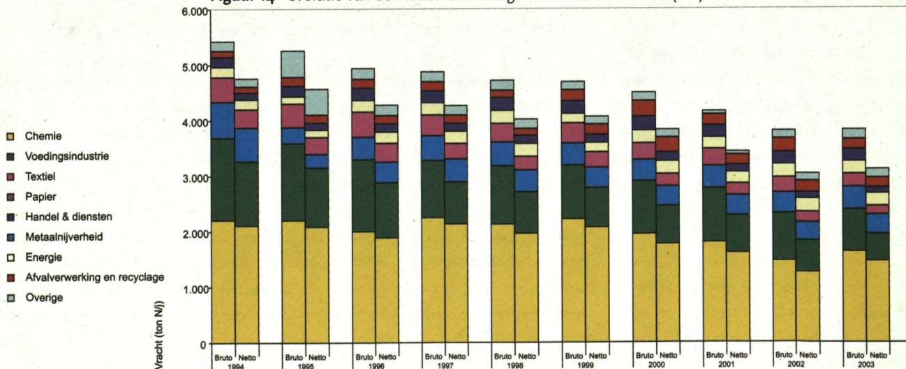
Figuur 14 - evolutie van de industriële lozingen voor totaal stikstof (N t)
