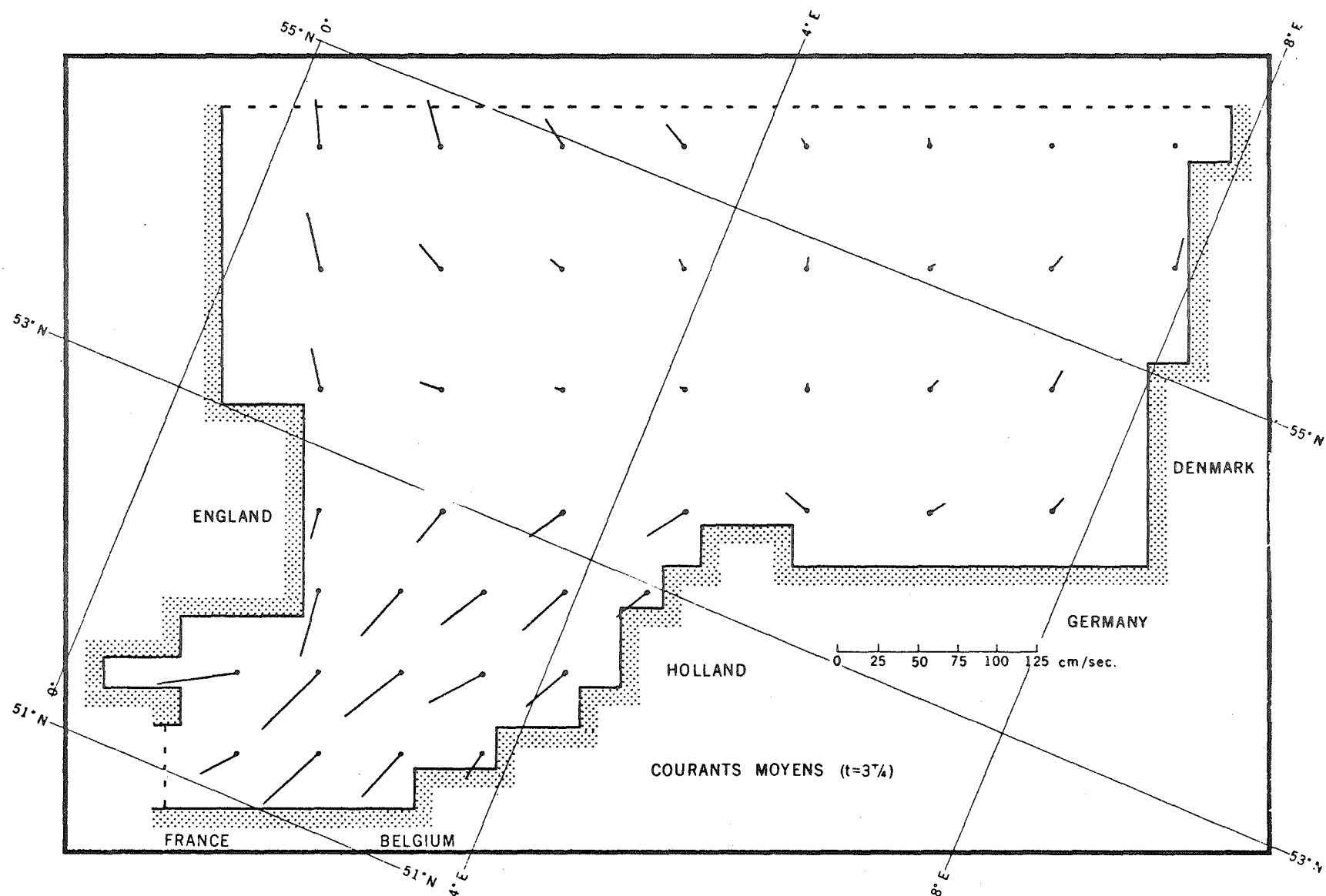
fig. 14.- Champ de vitesse calculé à t_{Gr} = \frac{3I}{4} dans le Southern Bight.
