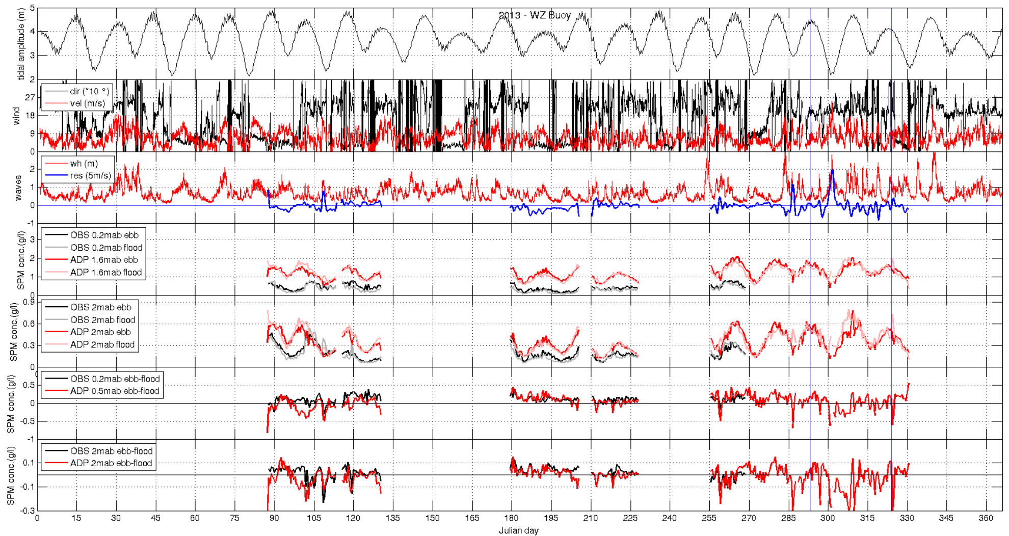
Figuur 5.12: WZ-Boei 2013, getijamplitude, windrichting (dir) en snelheid (vel, significante golfhoogte (wh), gemiddelde golfperiode (wp) en residuele alongshore stroming (res), verschil tussen eb- en vloedgemiddelde SPM concentratie dicht tegen de bodem en 2 m boven de bodem.
