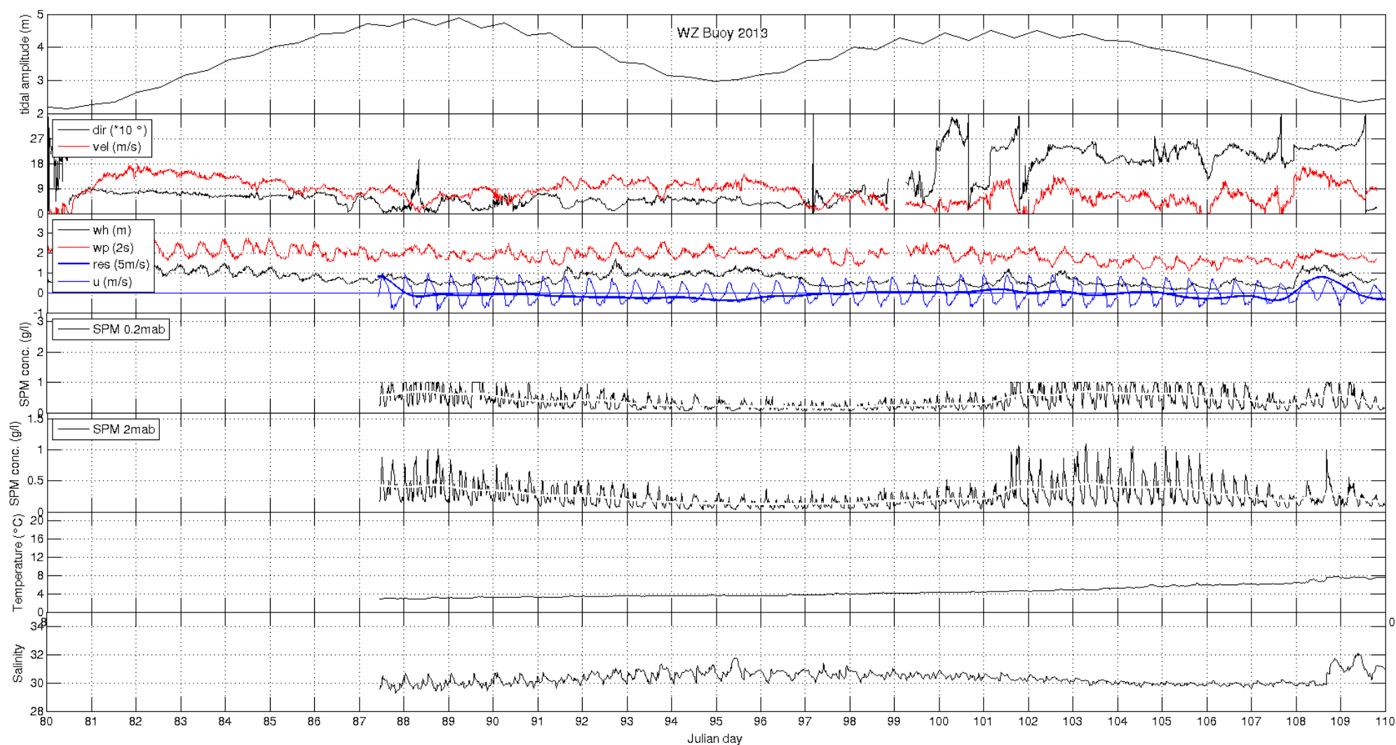
Figuur A4.1: WZ Boei 2013, getijamplitude, windrichting (dir) en snelheid (vel, significante golfhoogte (wh), gemiddelde golfperiode (wp, waarde gedeeld door 2), alongshore stroming (u, vloed is positief) en residuele alongshore stroming (res, waarde vermenigvuldigd met 5), OBS SPM concentratie op 0.2 en 2 m boven de bodem (witte lijn toont low-pass gefilterde SPM concentratie zonder getijsignaal), saliniteit, temperatuur.
