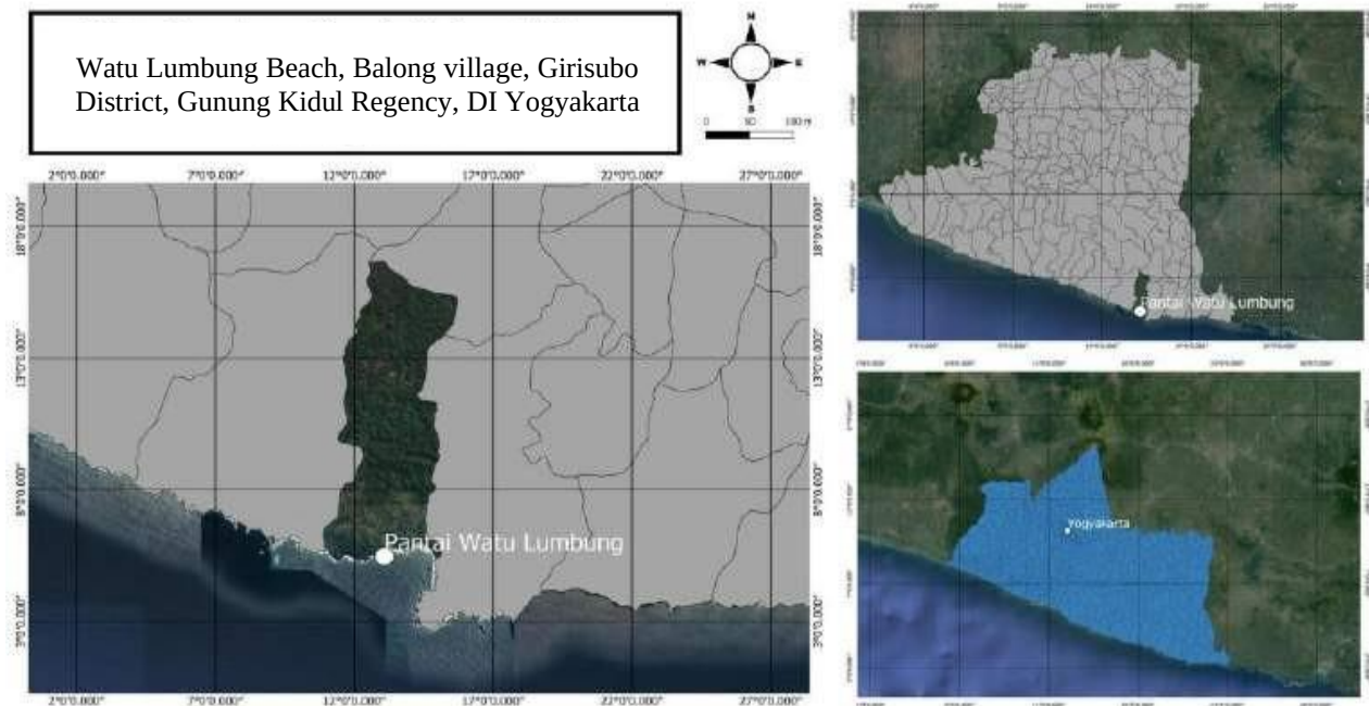
Fig. 1. Study sites in Watu Lumbung Beach, Gunungkidul
