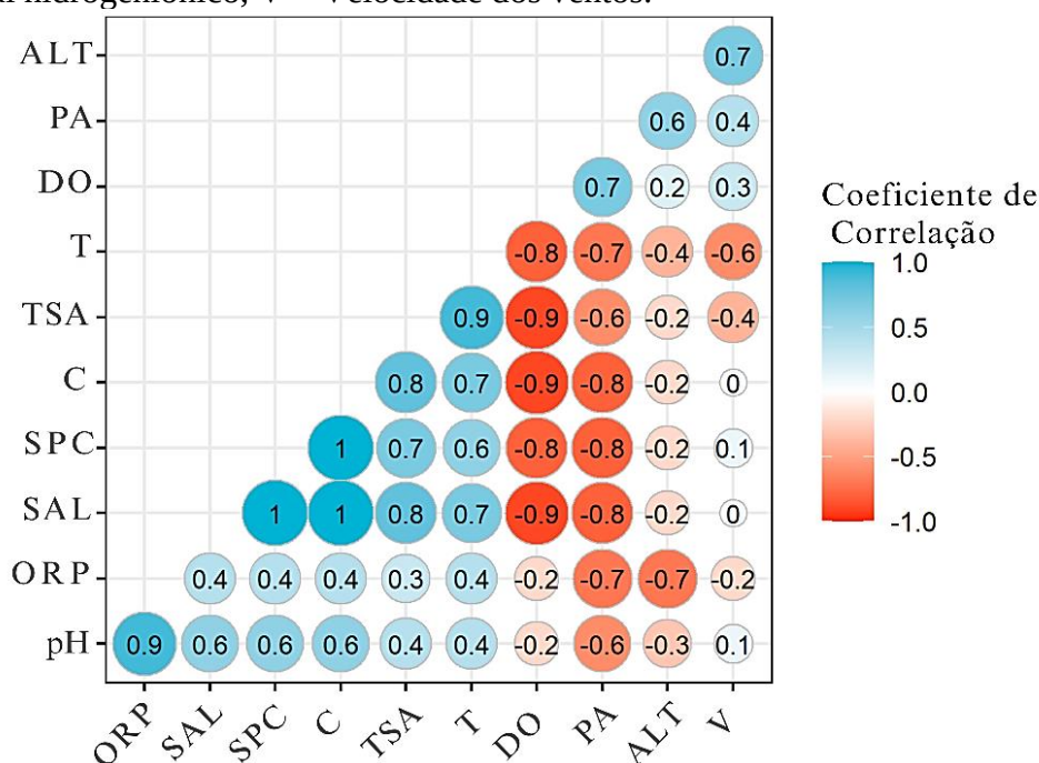
Figura 16: Matriz de correlação baseada no coeficiente de Pearson construída a partir dos valores das variáveis abióticas registradas nas campanhas de amostragem realizadas nos costões rochosos estudados. Onde ALT = Altura das ondas, PA= Precipitação acumulada, DO = Oxigênio dissolvido, T = Temperatura, TSA = Temperatura superficial da água, C = Condutividade, SPC = Condutância específica, SAL = Salinidade, ORP = Potencial redox e pH = Potencial hidrogeniônico, V = Velocidade dos ventos.
