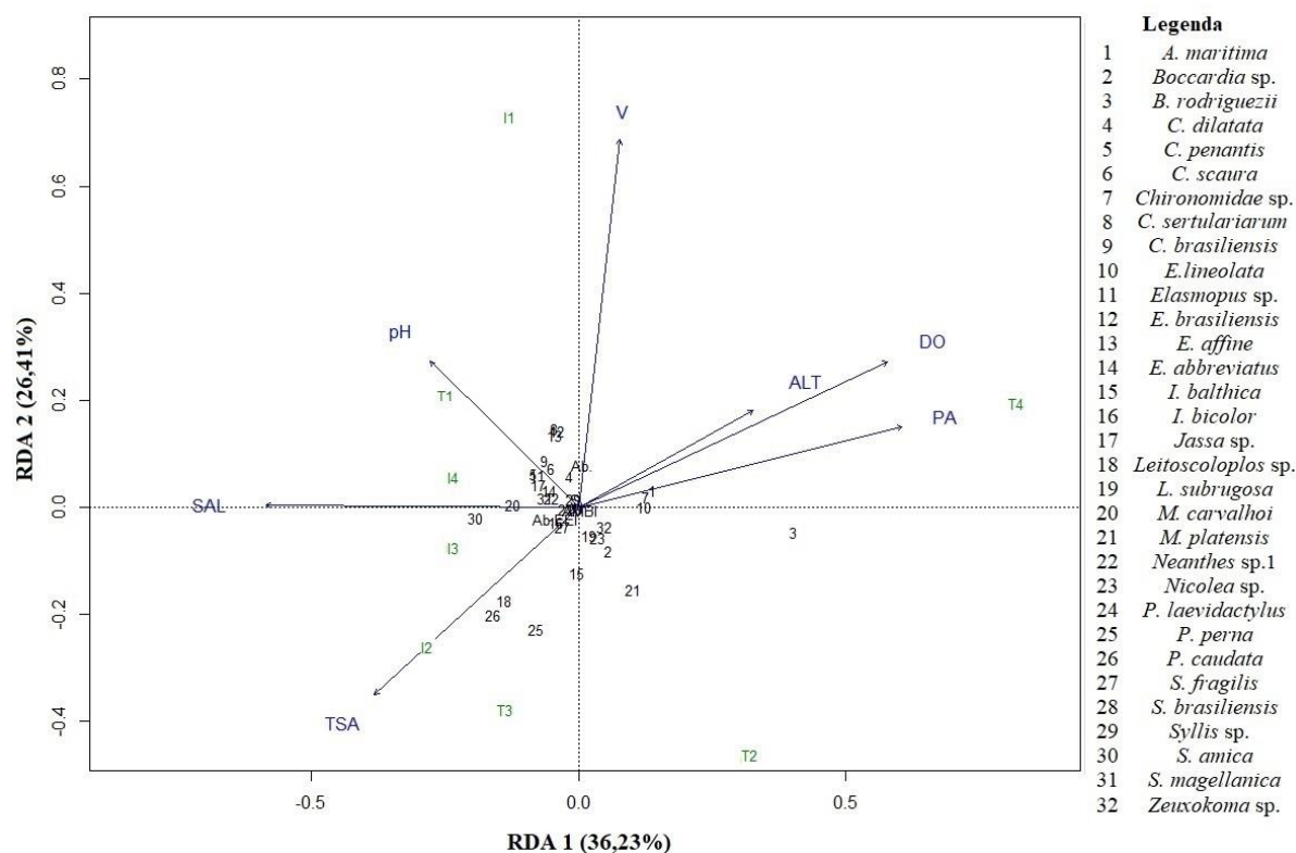
Figura 17: Representação dos dois principais eixos explicativos resultantes da Análise de Redundância (RDA) construída com os preditores abióticos e variáveis resposta registrados para os costões rochosos estudados. Onde I1, I2, I3 e I4 correspondem às campanhas realizadas em Imbituba e T1, T2, T3 e T4 correspondem às campanhas realizadas em Torres, ALT = Altura das ondas, DO = Oxigênio dissolvido, PA = Precipitação acumulada, pH = Potencial hidrogeniônico, SAL = Salinidade, TSA = Temperatura na superfície da água e V = Velocidade dos ventos.
