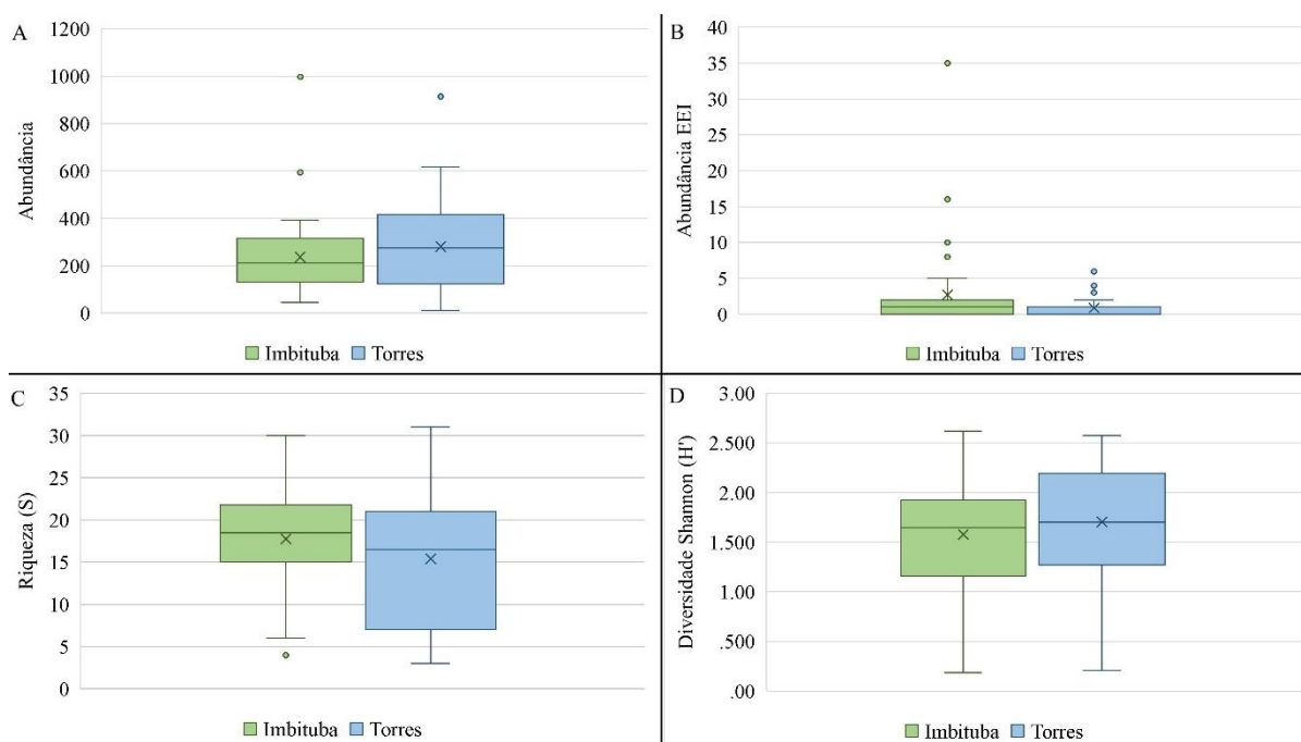
Figura 10: Bloxpots demonstrando a distribuição dos dados de abundância total, abundância de EEI, Riqueza (S) e Diversidade ( H' ) para o costão rochoso da praia da Ribanceira, Imbituba e da praia da Cal, Torres.
