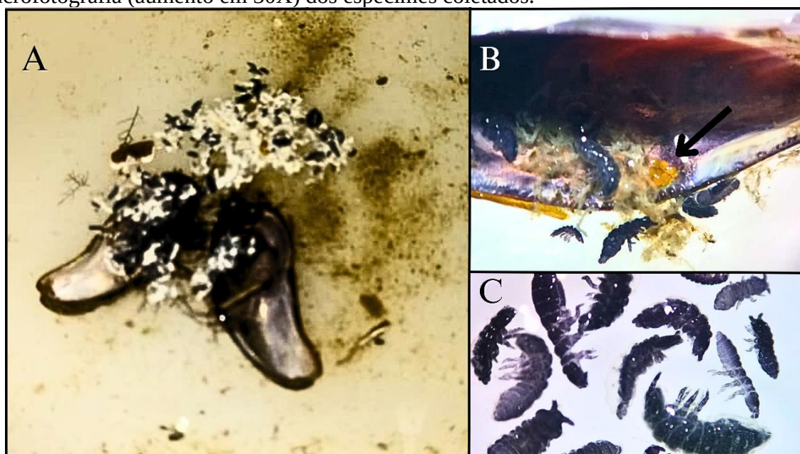
Figura 8: Imagens evidenciando as valvas de B. rodriguezii abertas durante triagem de um ponto amostral contendo os colêmbolos A. cf. maritima (A), macrofotografia (aumento em 20X) da valva com os ovos (apontado pela seta), exúvias e indivíduos de A. cf. maritima (B), e macrofotografia (aumento em 30X) dos espécimes coletados.
