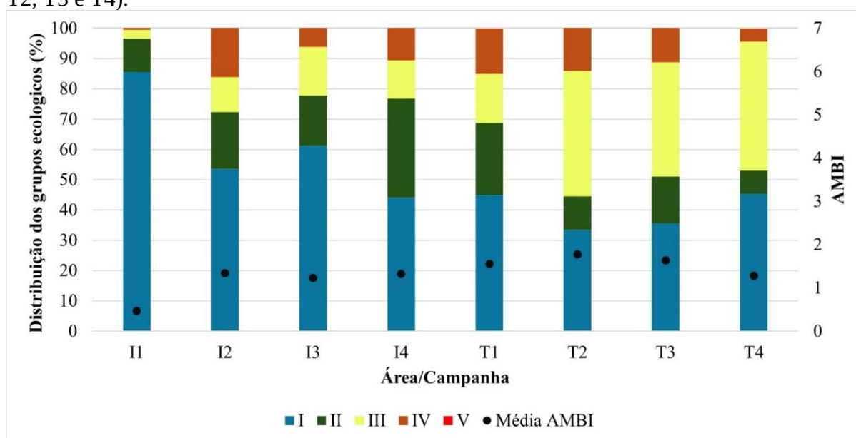
Figura 14: Proporção dos grupos ecológicos dos macroinvertebrados coletados e média AMBI em cada campanha na praia da Ribanceira, Imbituba (I1, I2, I3 e I4) e praia da Cal, Torres (T1, T2, T3 e T4).
