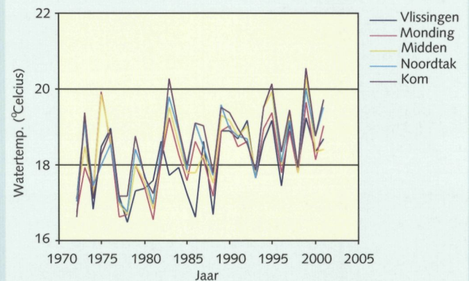
Figuur 5.1b: Gemiddelde watertemperatuur over de zomerperiode berekend voor de vier deelgebieden in de Oosterschelde.
