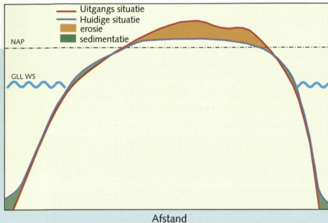
Figuur 4.4: Schematische weergave van de aanpassing van de platen aan het gedempt getij in de Oosterschelde (GLLWS betekent Gemiddeld Laag Laag Water Springtij, dit is de laagste laagwaterlijn, deze komt slechts af en toe voor).
