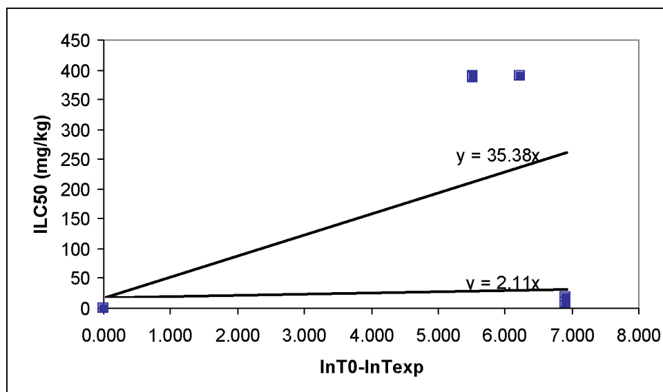
Figuur 4.1: ILC_{50} - \ln T relatie van fluorantheen voor vissen.
