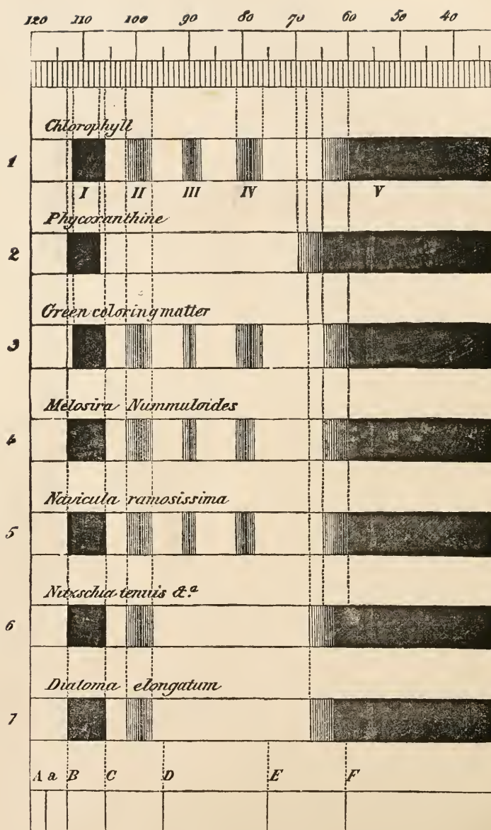
FIG. 3. — Spectre donné par certaines diatomées et par la chlorophylle. (d'après M. P. Petit. — Cliché de la Royal microscopical Society de Londres.)
