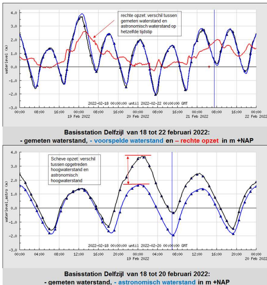
Figuur 24: Verschuivingen in getijwaterstand
