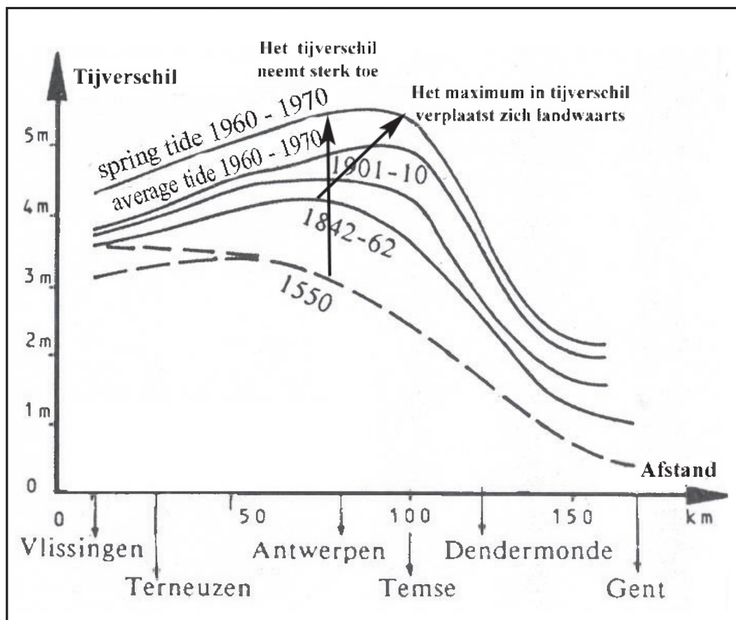
Figuur 2. Evolutie van het tijverschil van 1550 tot 1970. De pijlen geven aan hoe in de buurt van Antwerpen het tijverschil toeneemt en het maximum in tijverschil zich landwaarts verplaatst (bron: Coen, 1988).
