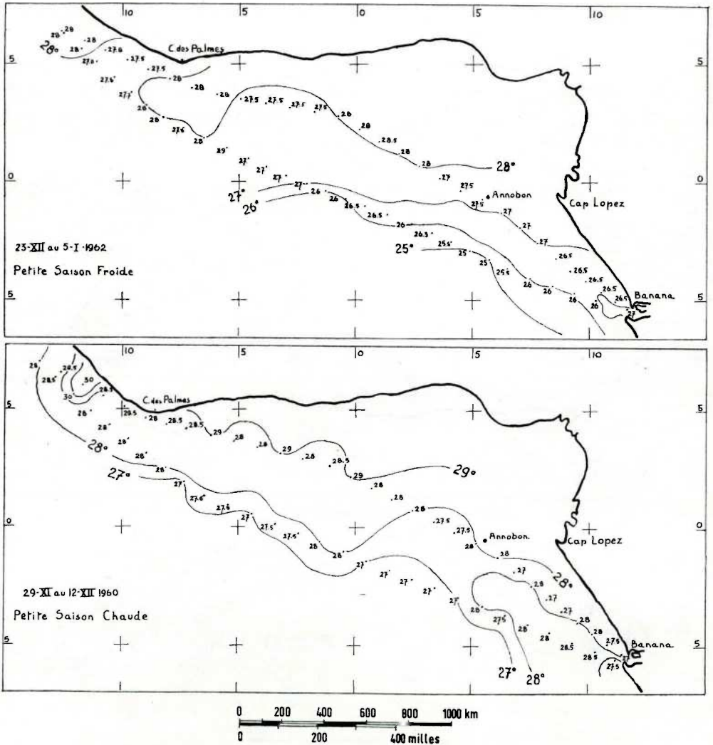
FIG. 7 C-D. — Déplacement des isothermes au cours des saisons marines, montrant la « pulsation » des eaux guinéennes
