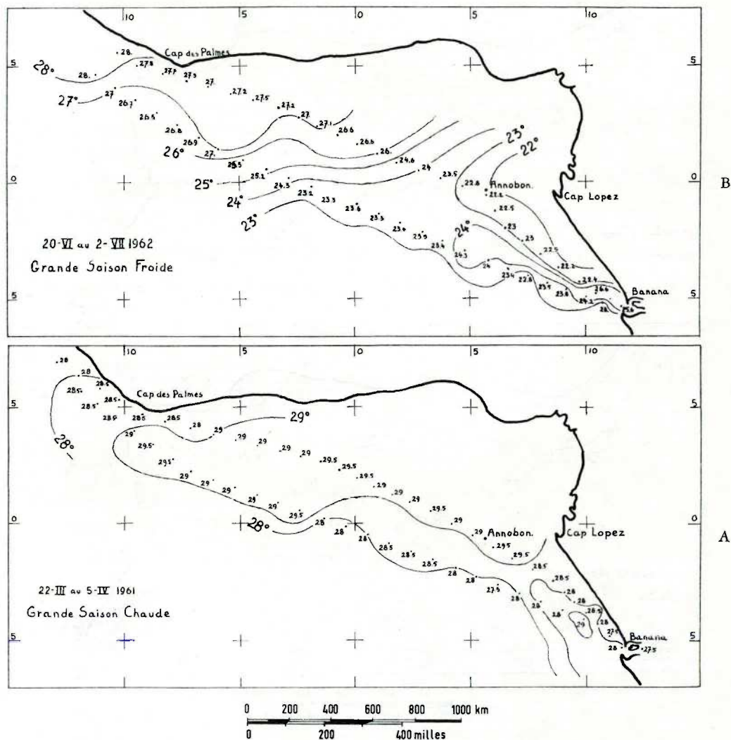
FIG. 7 A-B. — Déplacement des isothermes au cours des saisons marines, montrant la « pulsation » des eaux guinéennes
