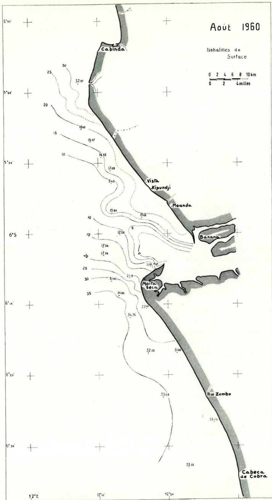
FIG. 35. — Août 1960. Isohalines de surface
