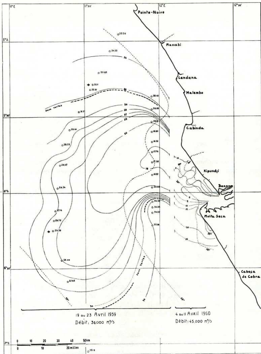
FIG. 44. — Situation de surface en avril 1959 au large, et à la côte en 1960
