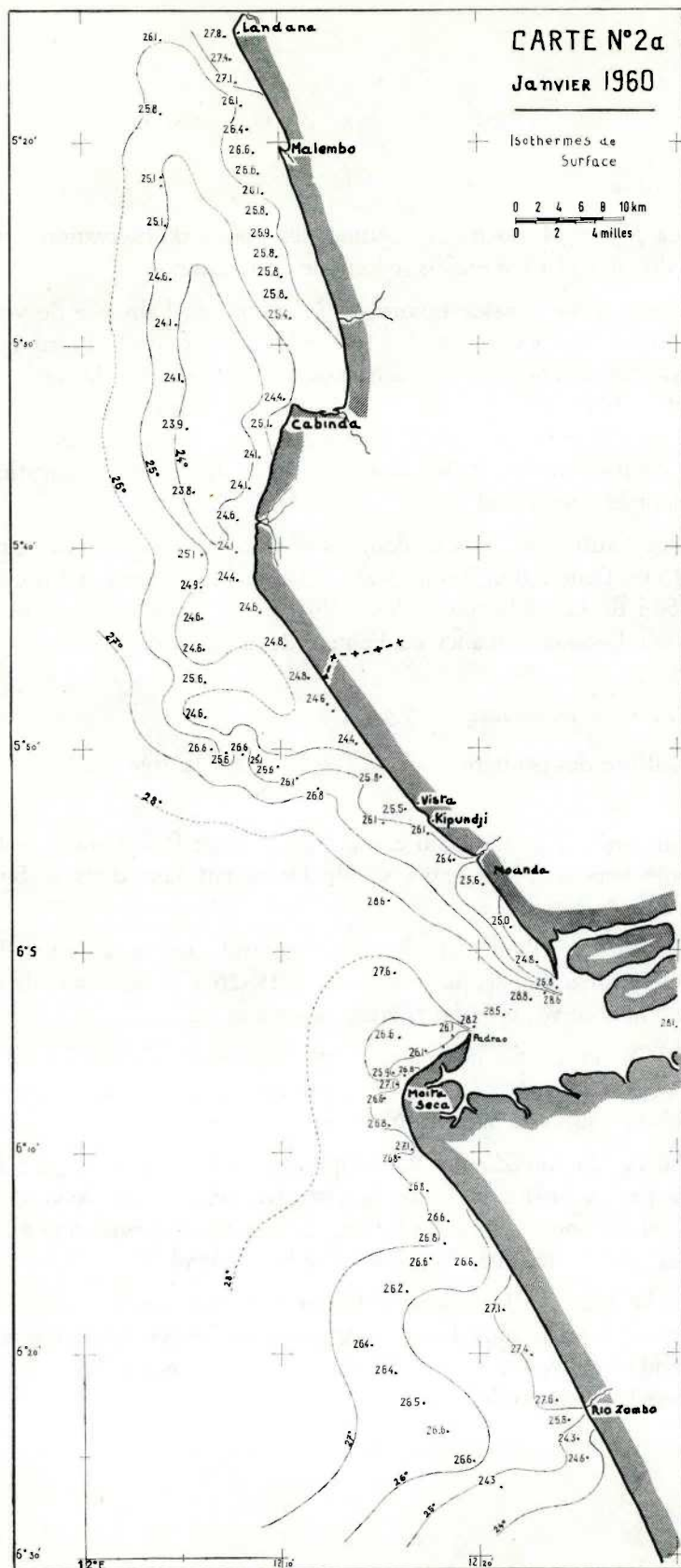
FIG. 22. — Janvier 1960. Isothermes de surface
