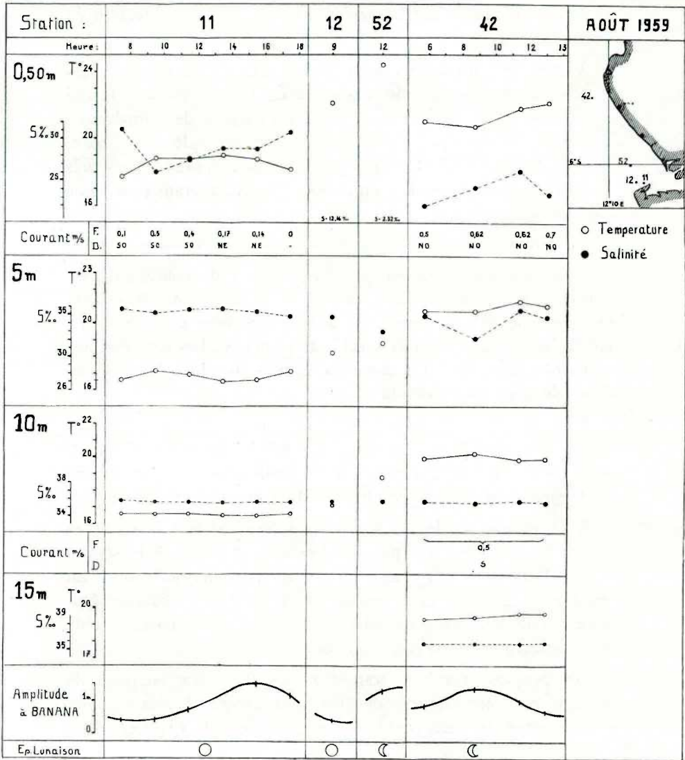
FIG. 19. -- Août 1959. Graphique des variations de salinité et température aux stations principales en fonction de la marée
