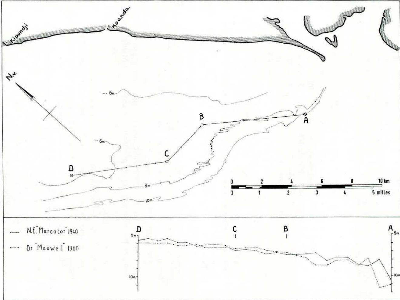
FIG. 5. — Comparaison des profils en 1940 et 1960
