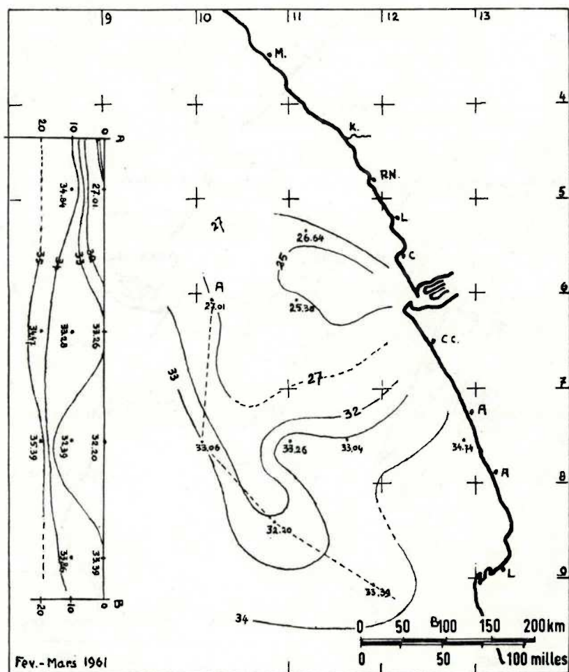
FIG. 46. — Isohalines de surface et profil, février-mars 1961
