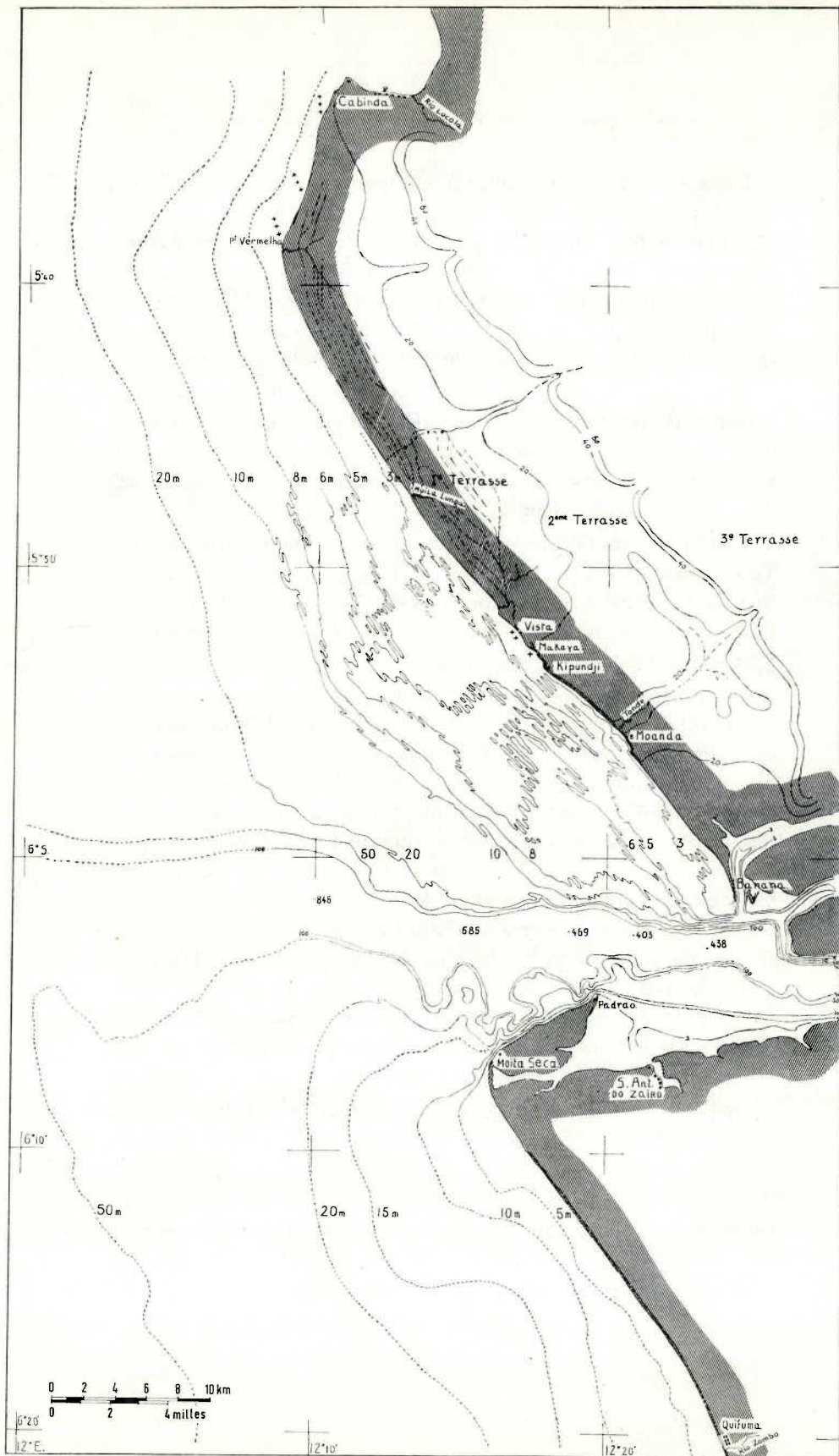
FIG. 3. — Topographie des fonds côtiers
