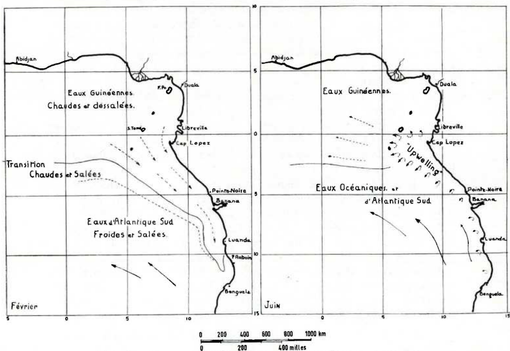
FIG. 6. — Mouvement schématique des masses d'eau au cours des saisons marines
