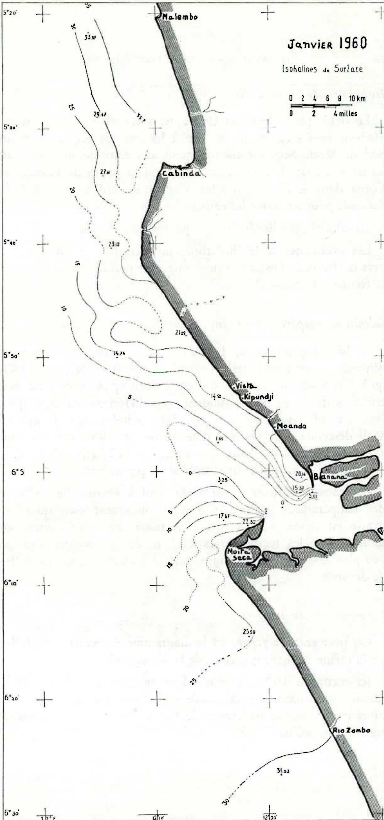
FIG. 23. — Janvier 1960. Isohalines de surface
