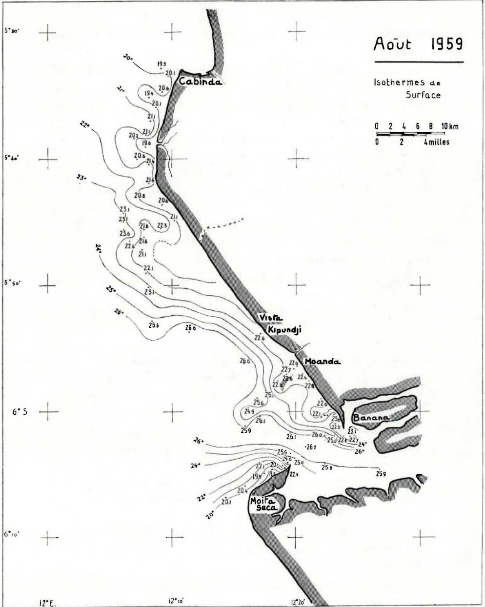
FIG. 16. — Août 1959. Isothermes de surface
