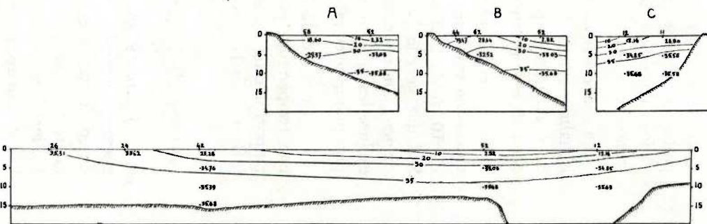
FIG. 18. — Août 1959. Bloc-diagramme donnant la situation générale. — Profil sur l'isobathe de 15 m; A, B et C, profils en travers
