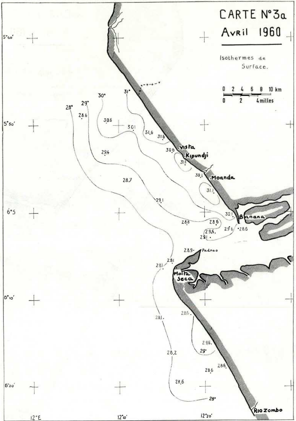
FIG. 28. — Avril 1960. Isothermes de surface
