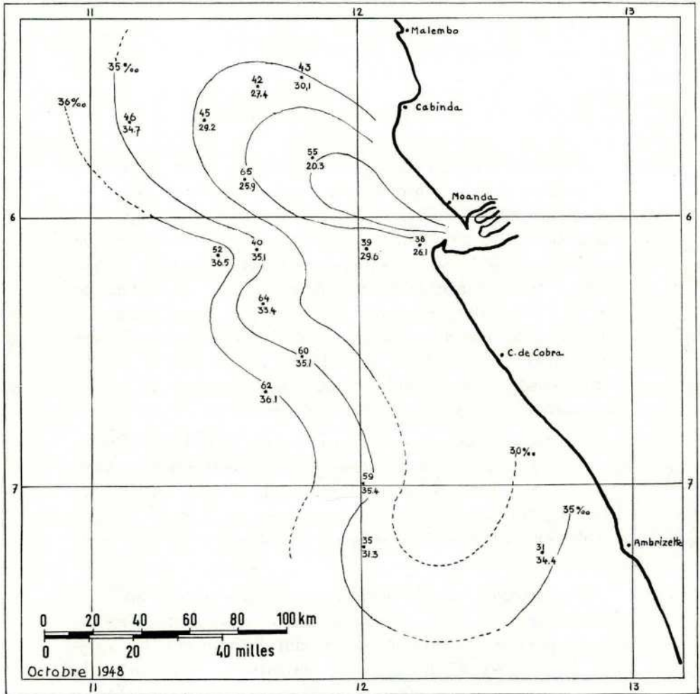
FIG. 43. — Position et salinité de surface des stations du NOORDEINDE , du 29 septembre au 13 novembre 1948
