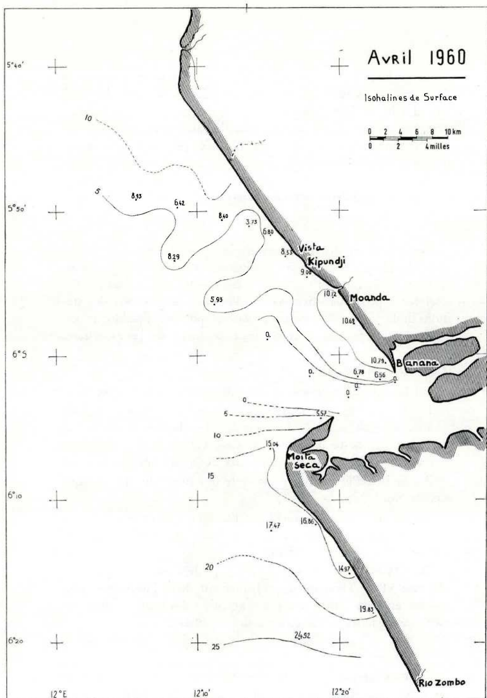
FIG. 29. — Avril 1960. Isohalines de surface
