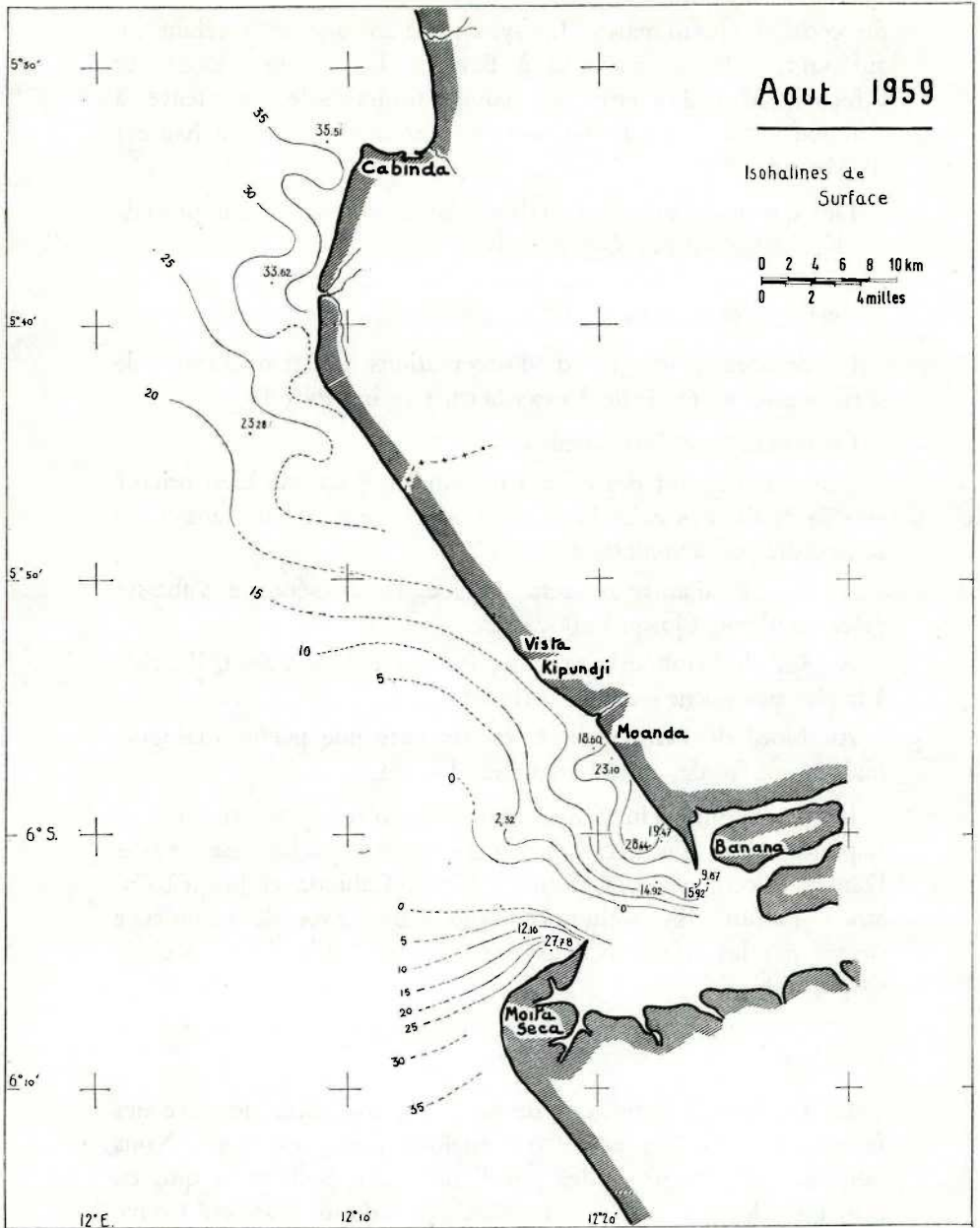
FIG. 17. — Août 1959. Isohalines de surface
