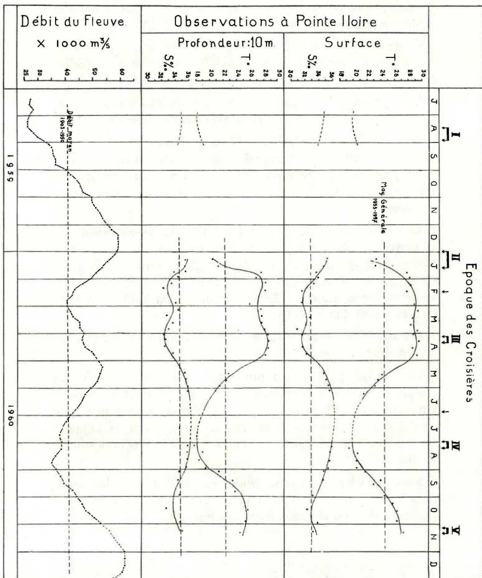
FIG. 14. — Conditions de température et salinité observées à Pointe-Noire et régime du fleuve d'août 1959 à novembre 1960
