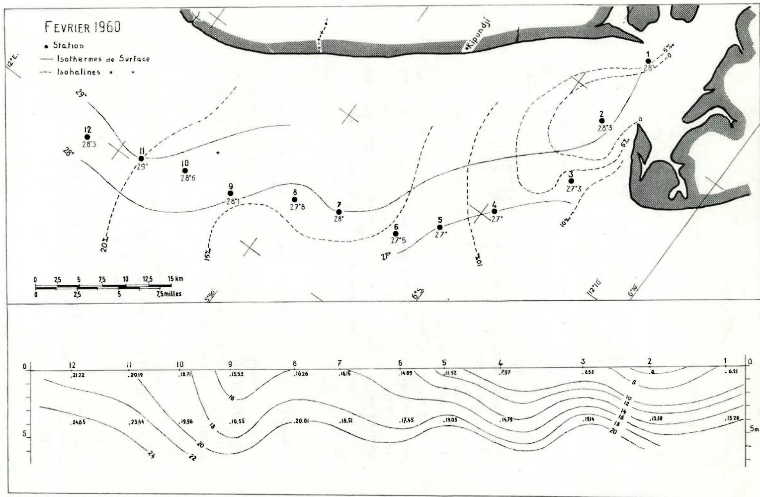
FIG. 26. — Février 1960. Isothermes et isohalines en surface, et isohalines en profondeur
