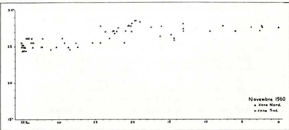
FIG. 20 D-E. — Diagramme t/S se rapportant aux différentes croisières:
