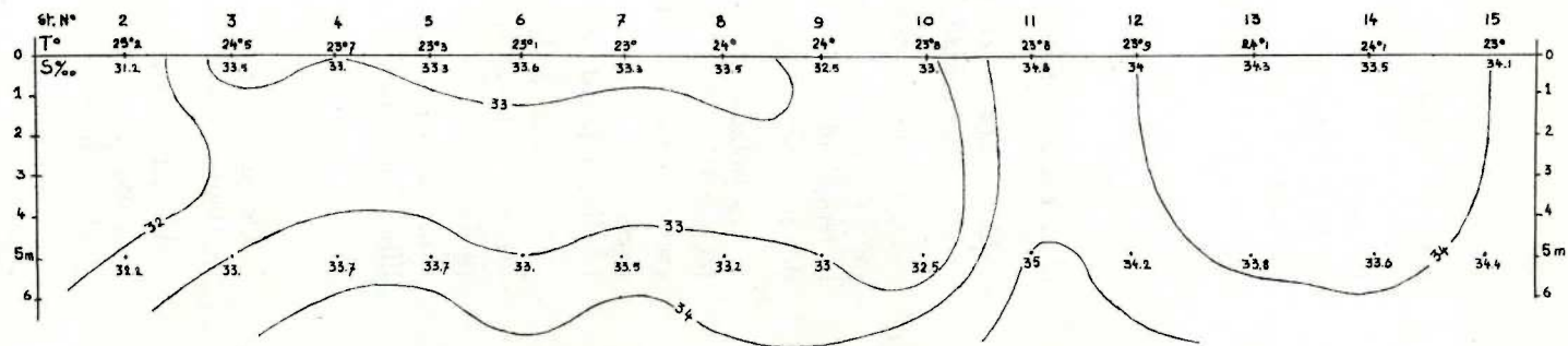
FIG. 48. — Situation de surface et profil dans le Sud, octobre 1962
