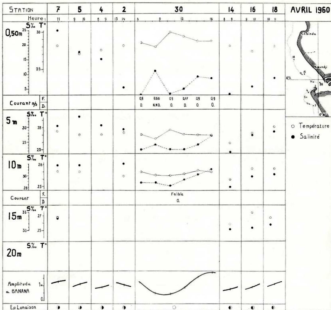
FIG. 31. — Avril 1960. Graphique des variations de salinité et température en fonction de la marée
