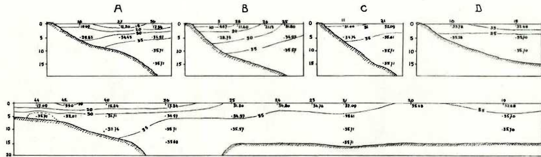
FIG. 36. — Août 1960. Bloc-diagramme donnant la situation générale. — Profil sur l'isobathe de 15 m; A, B, C et D, profils en travers
