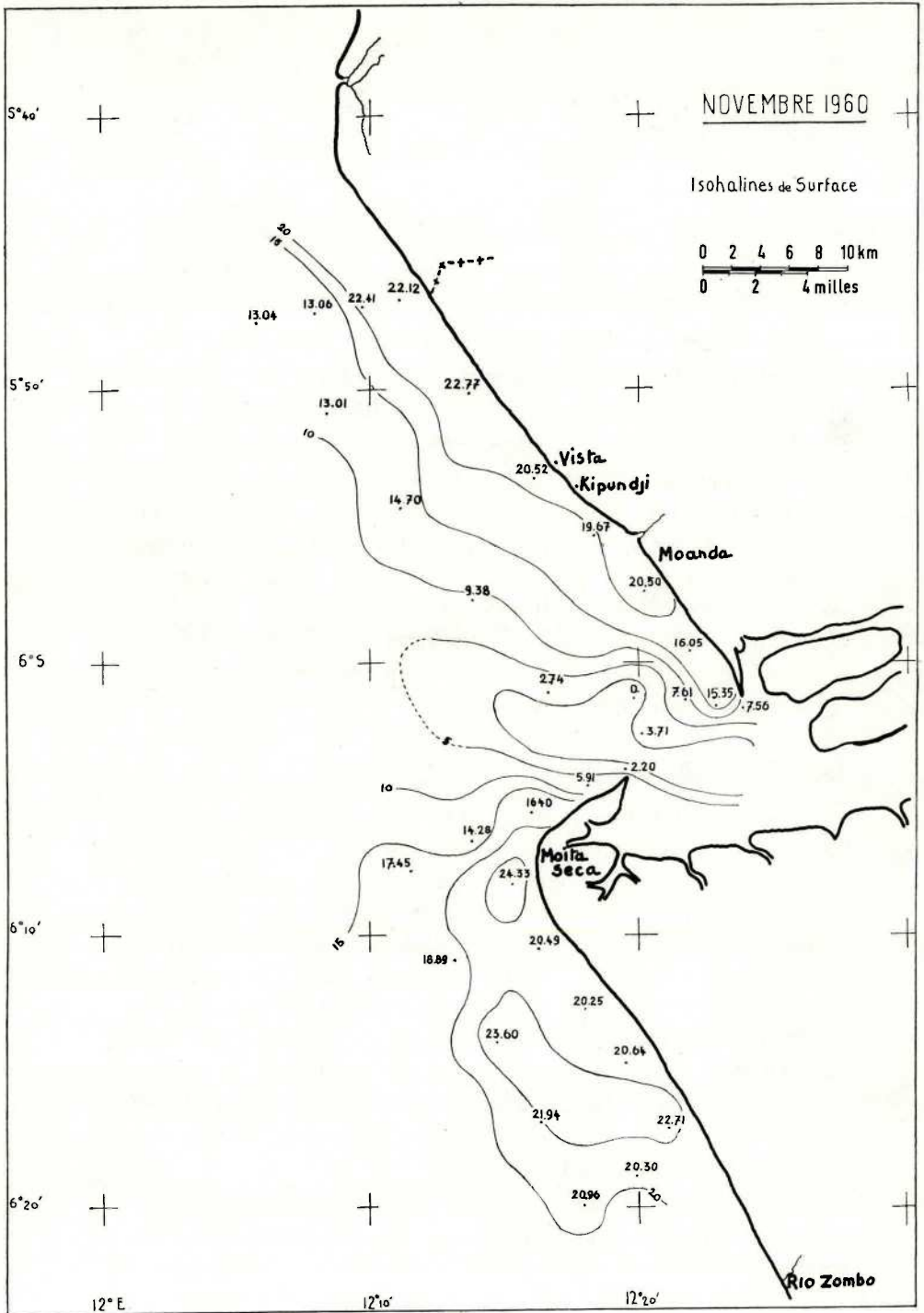
FIG. 40. — Novembre 1960. Isohalines de surface
