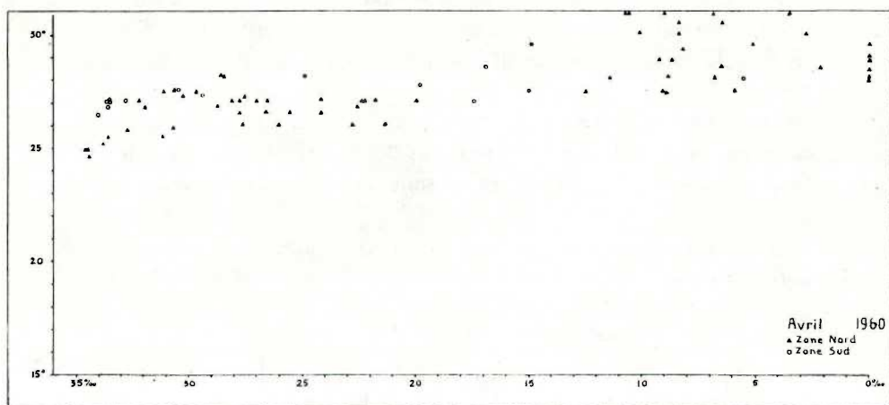
FIG. 20 A-B-C. — Diagramme t/S se rapportant aux différentes croisières:
