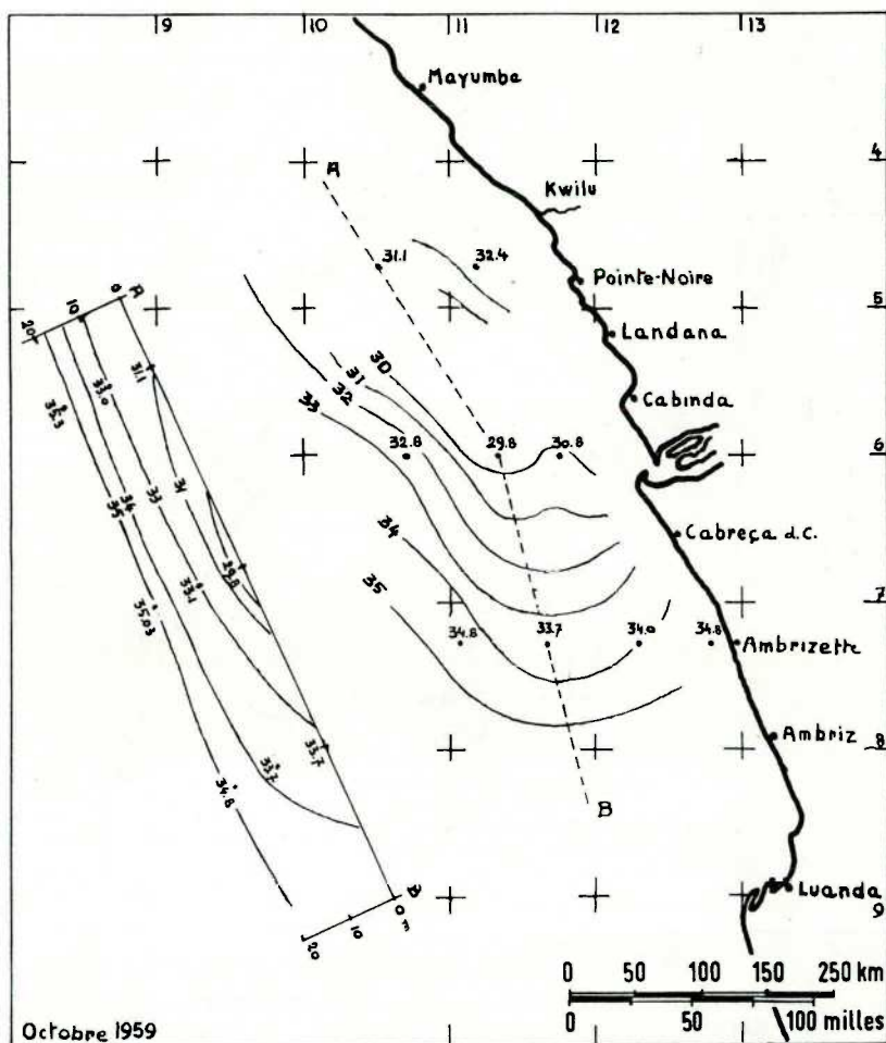
FIG. 45. — Isohalines de surface et profil, octobre 1959
