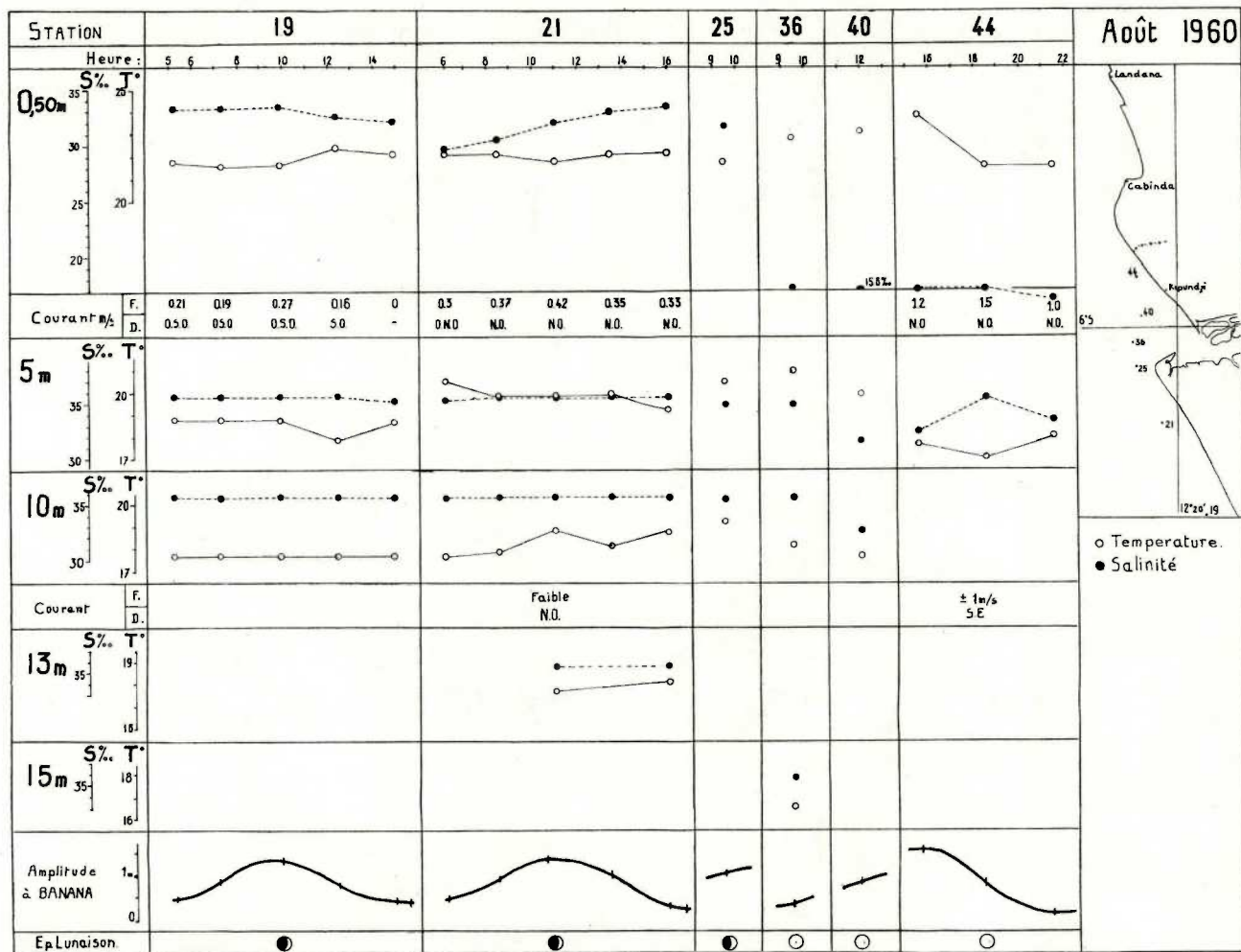
FIG. 37. — Août 1960. Graphique des variations de salinité et température aux stations principales, en fonction de la marée
