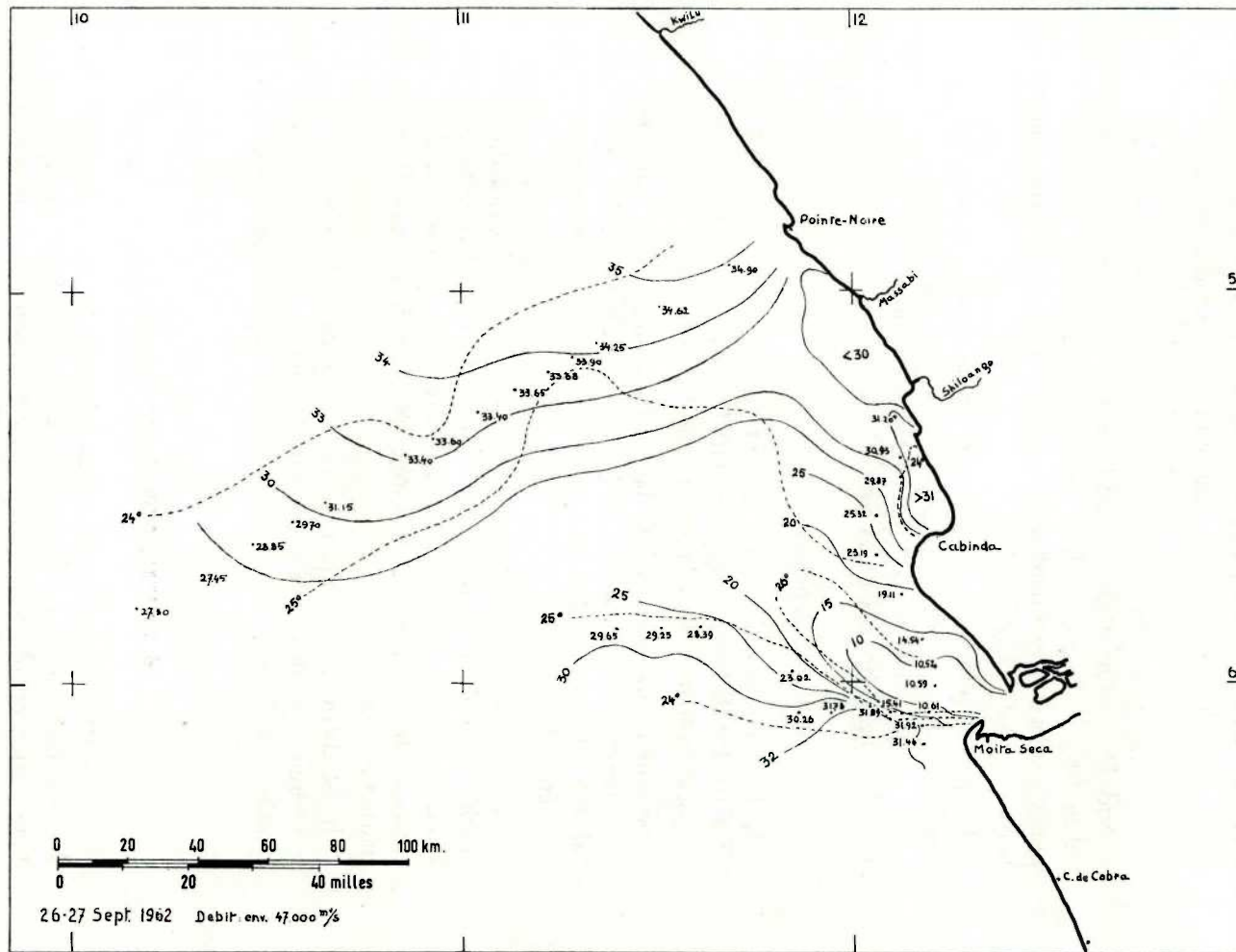
FIG. 47. — Situation de surface à l'embouchure, septembre 1962
