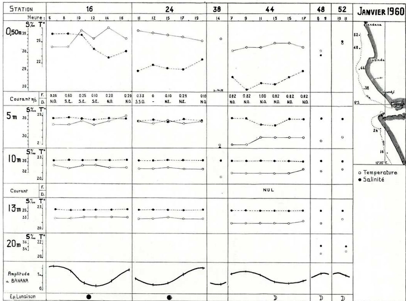
FIG. 25. — Janvier 1960. Graphique des variations de salinité et température aux stations principales en fonction de la marée
