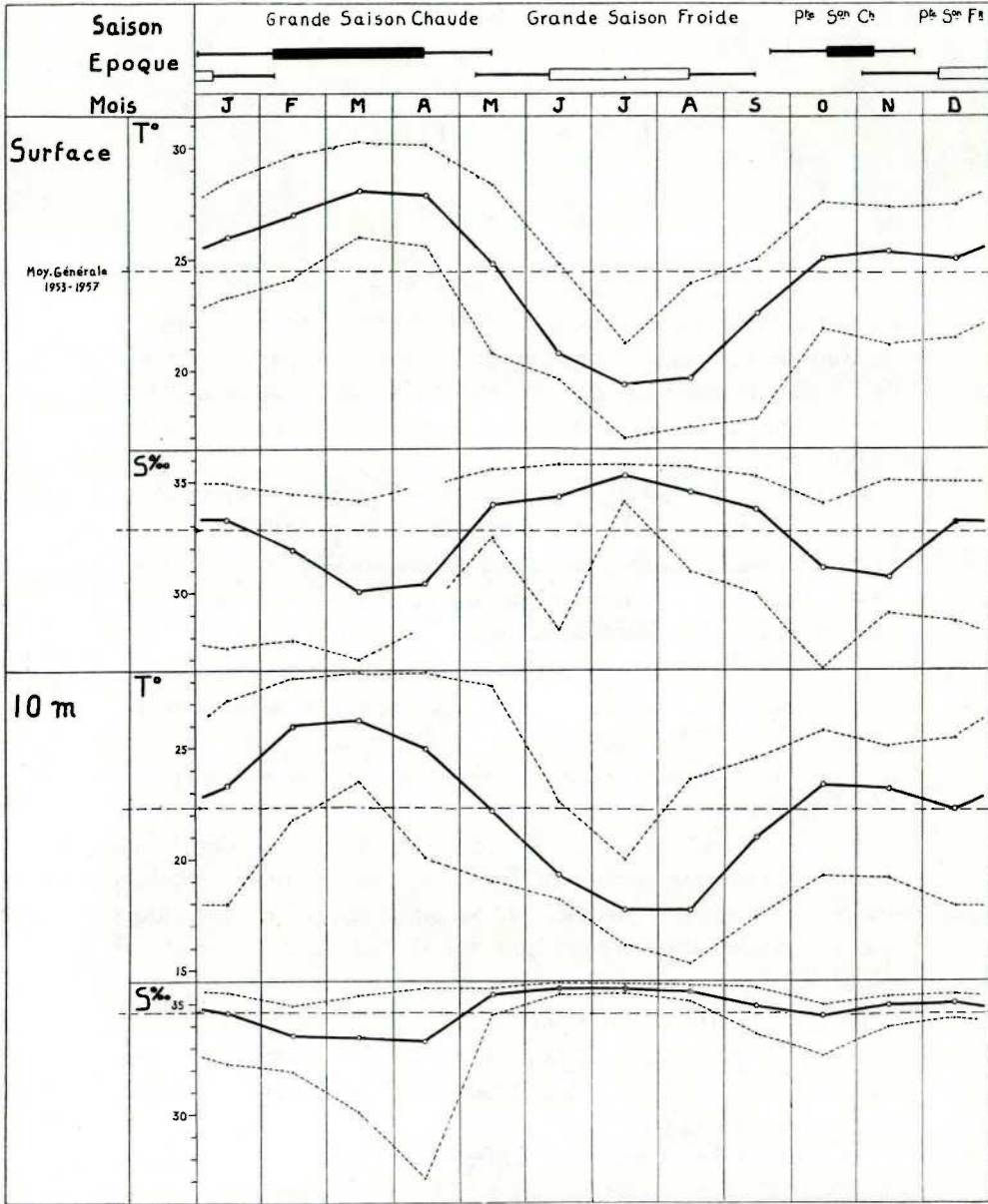
FIG. 8. — Graphique général des variations de température et de salinité en fonction des saisons marines à Pointe-Noire
