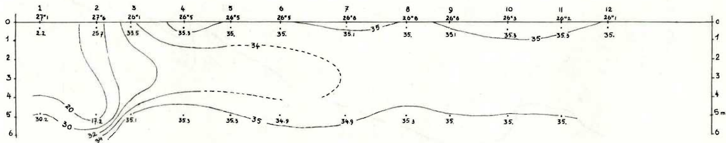
FIG. 49. — Situation de surface et profil dans le Sud, janvier 1963
