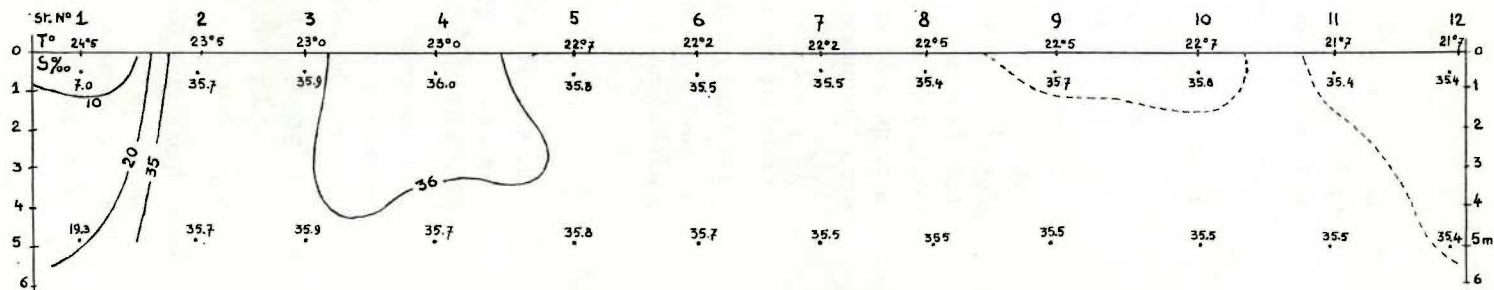
FIG. 51. — Situation de surface et profil dans le Sud, juillet 1963
