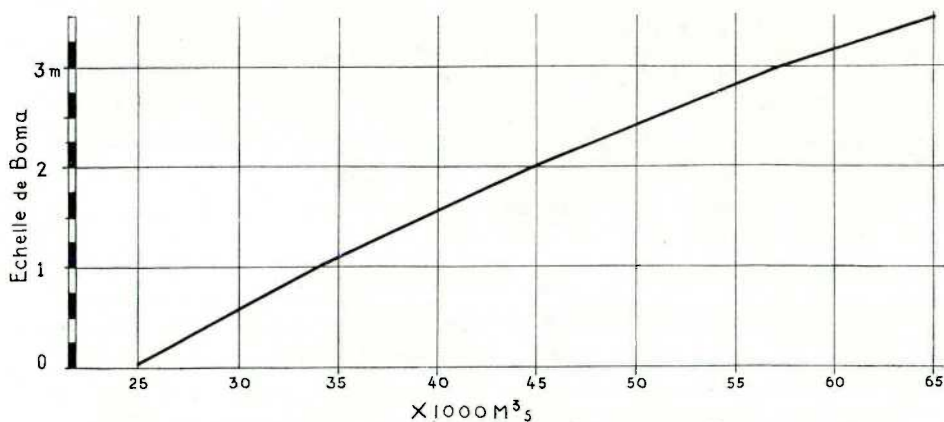
FIG. 9. — Variation de l'étiage à Boma et débit correspondant à cet étiage
