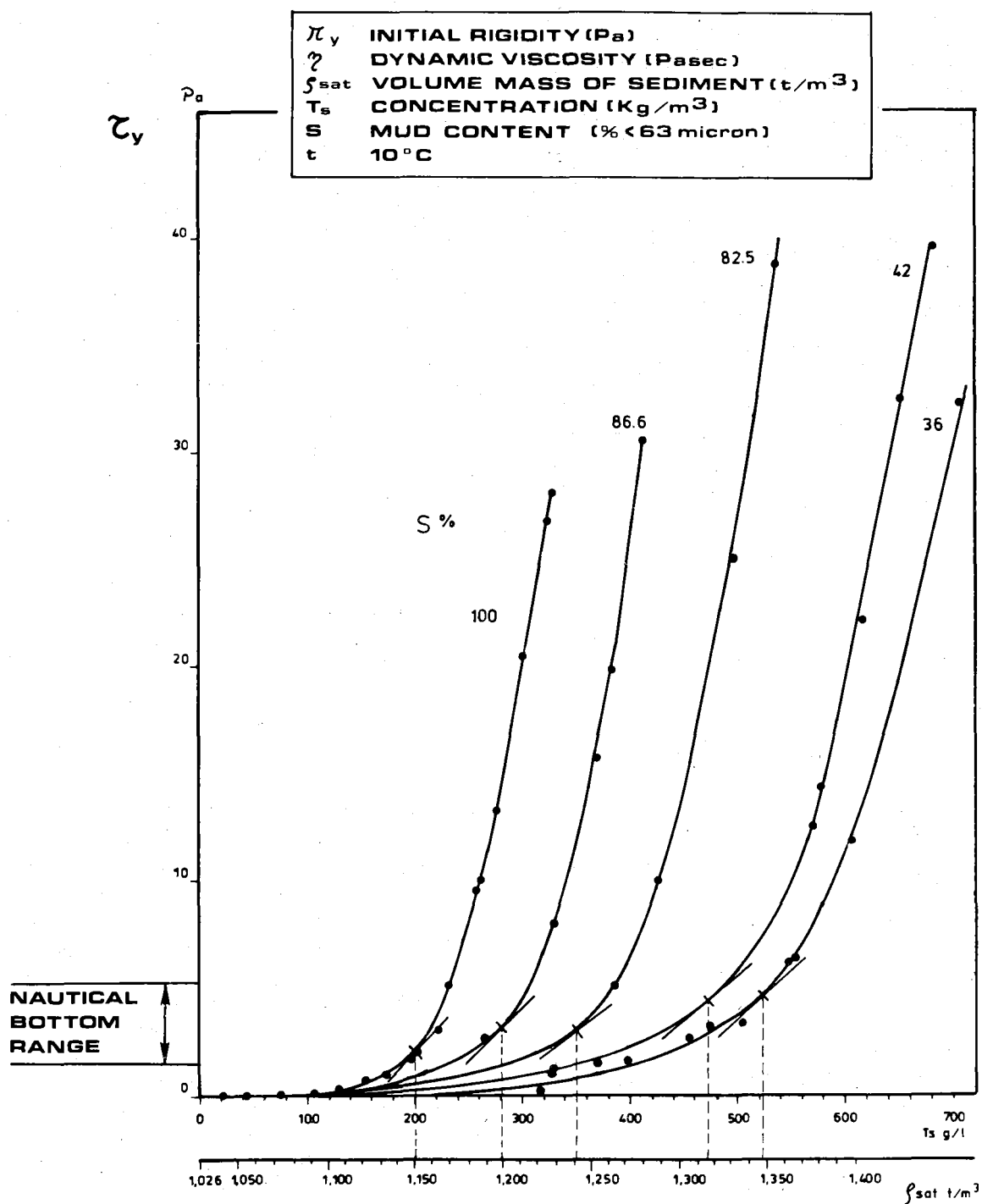
Figure 4 : Initial rigidity \tau_y in function of concentration and mud composition (Zeebrugge). Rigidité initiale \tau_y en fonction de la concentration et de la composition.
