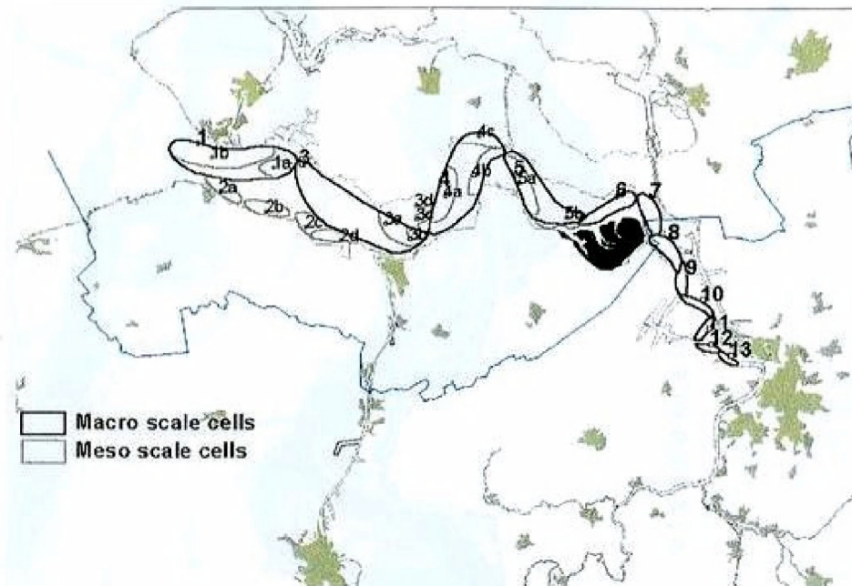
Figuur 2.1 Macro- en mesocellen in de Westerschelde (Winterwerp e.a., 2000).
