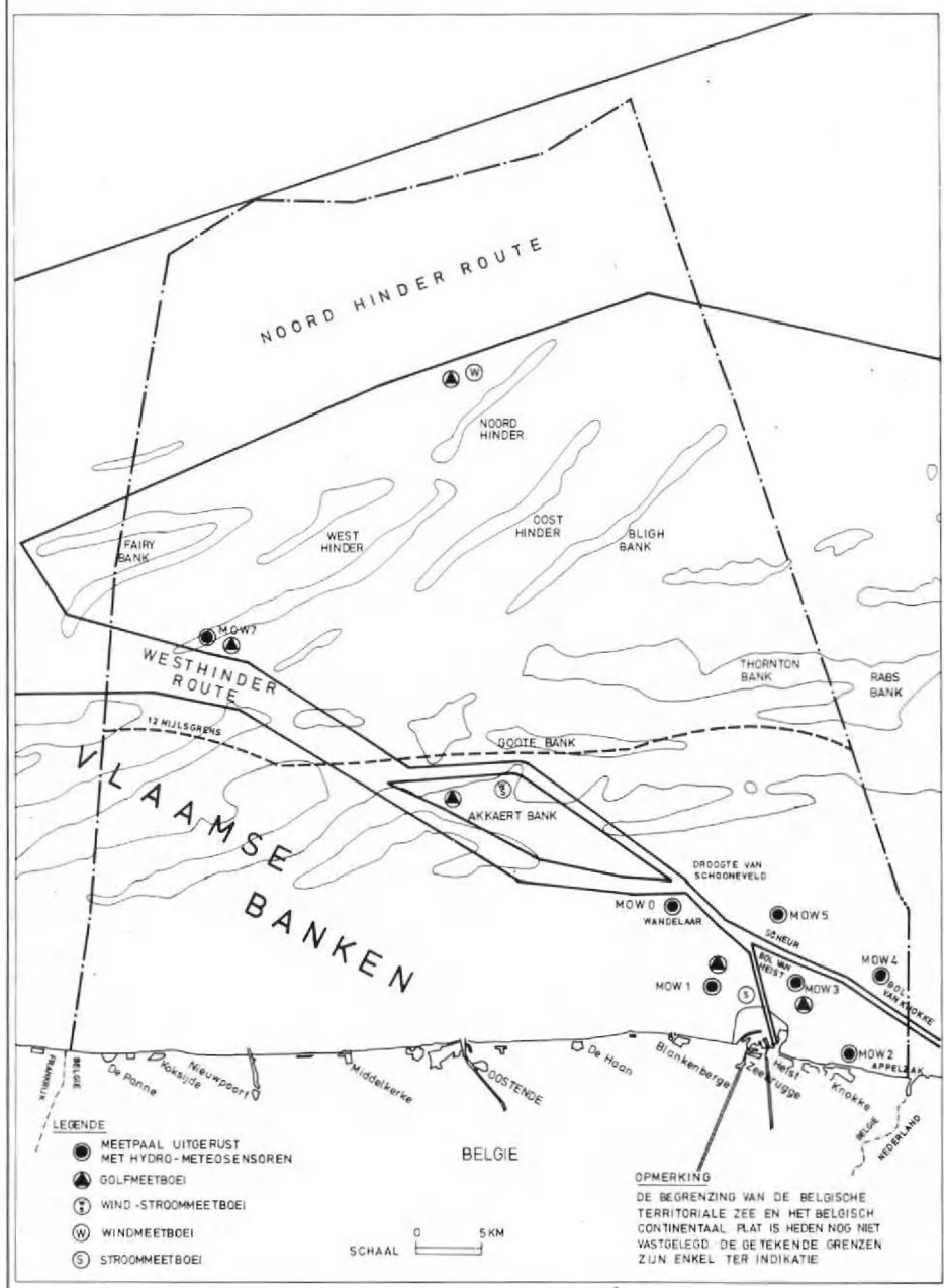
Fig. 2 Meetsensoren op het Belgisch Continentaal Plat.
