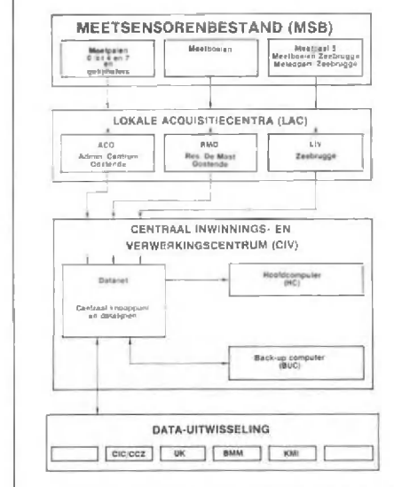
Fig. 1 Onderdelen van het meetnet «Vlaamse Banken»
