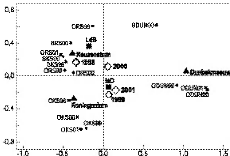
Fig. 19. Ordinatie diagram gebaseerd op distance based Redundancy Analysis (db-RDA) van 15 faecesmonsters van Reuzenster, Koningsster en Dunbekmeeuw van Ile aux Oiseaux en Langue de Barbarie uit de periode 1998-2001. De punten voor de klassen (vogelsoorten en gebieden) zijn de centroiden van de monsters waartoe ze behoren. De afstand tussen de punten is bepalend voor de mate van overeenkomst. Voor verdere uitleg zie tekst en bijlage 7.
