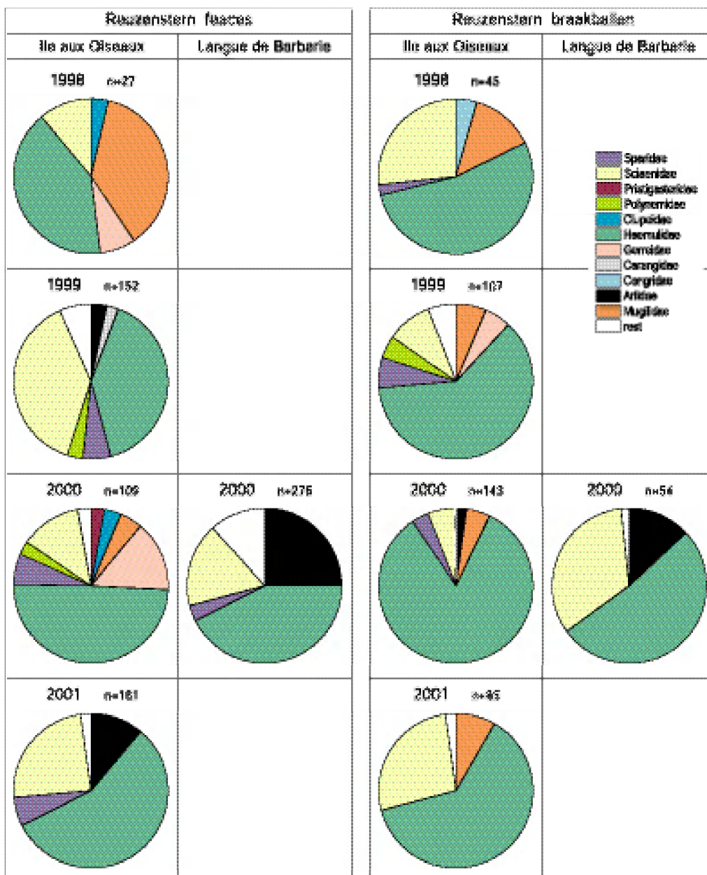
Fig. 17. Samenstelling van het voedsel van de Reuzenster op Ile aux Oiseaux (1998-2001) en de Langue de Barbarie (2000) gebaseerd op otolieten in braakballen en faeces. De diagrammen geven het percentage weer van alle vissenfamilies die meer dan 2% uitmaken van het monster uit een bepaald jaar.
