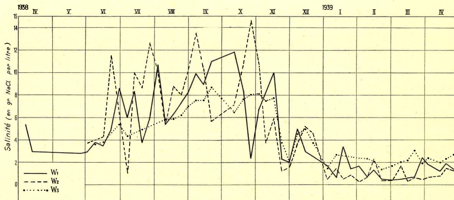
FIG. 22. — Variations hebdomadaires de la salinité du Watergang aux stations W 1 , W 2 et W 3 .
