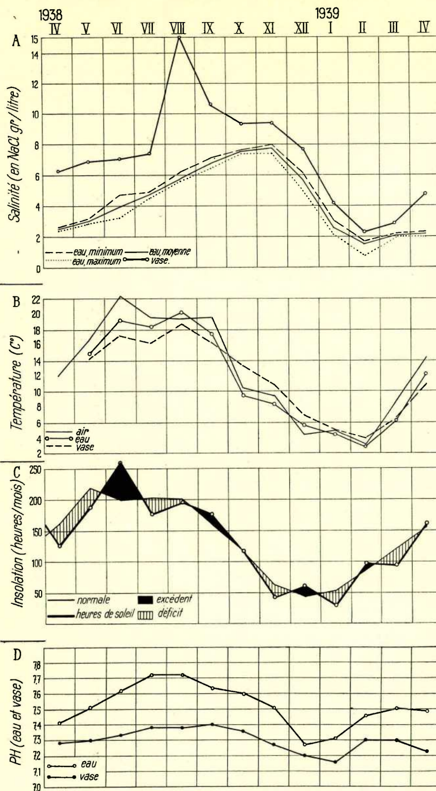
FIG. 7. — Variations saisonnières de la salinité, de la température, de l'insolation, du pH. (Dans le diagramme A, il faut lire : ---, max.; . . . , min.)
