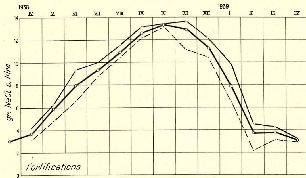
FIG. 25. — Variations saisonnières de la salinité (fossés des fortifications). —, maximum; ---, minimum; —, moyenne.
