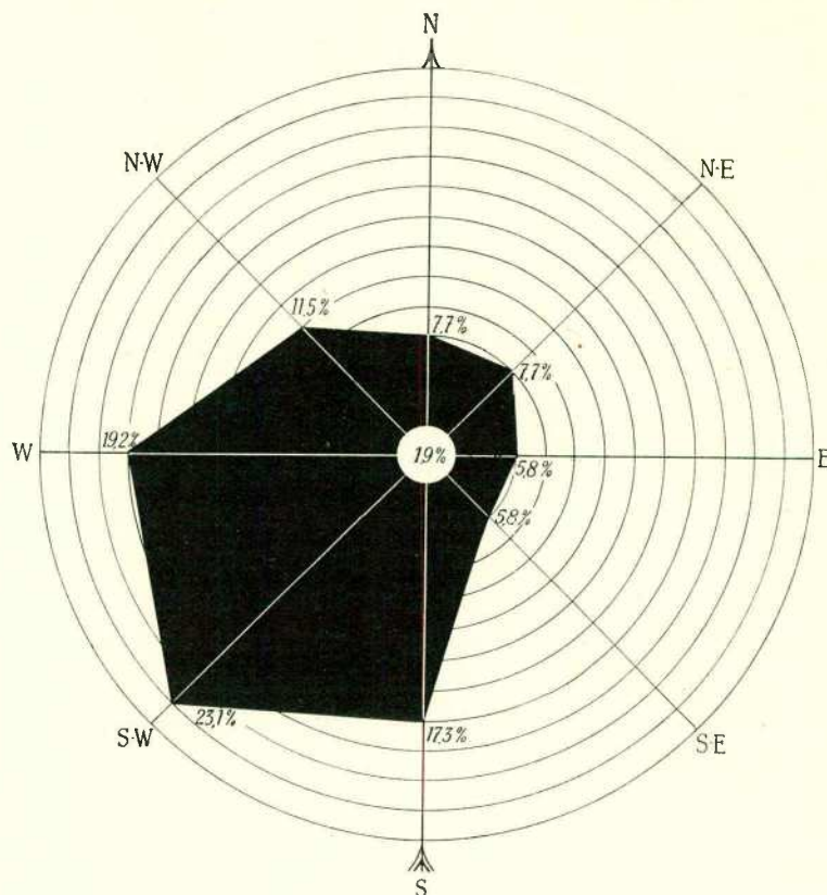
FIG. 4. — Rose de fréquence des vents.
