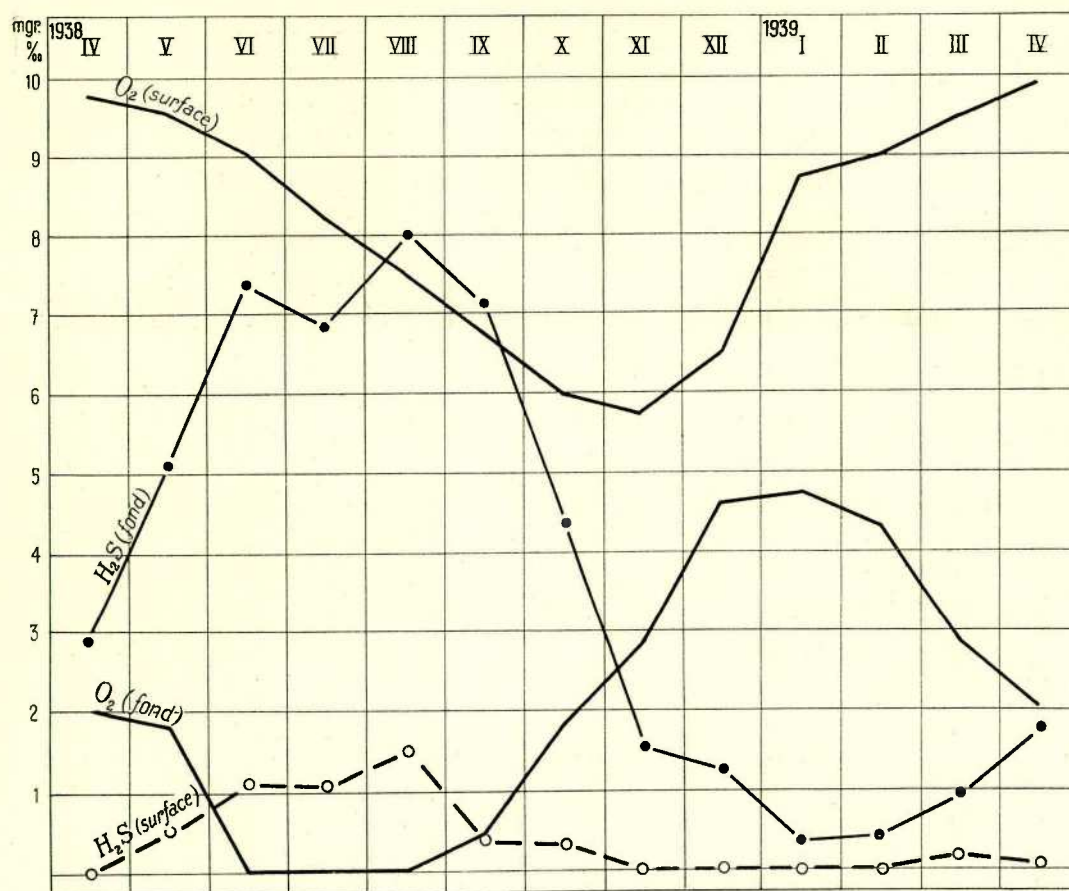
FIG. 13. — Variations saisonnières de O_2 et H_2S , à la surface et au fond de l'eau du Put.
