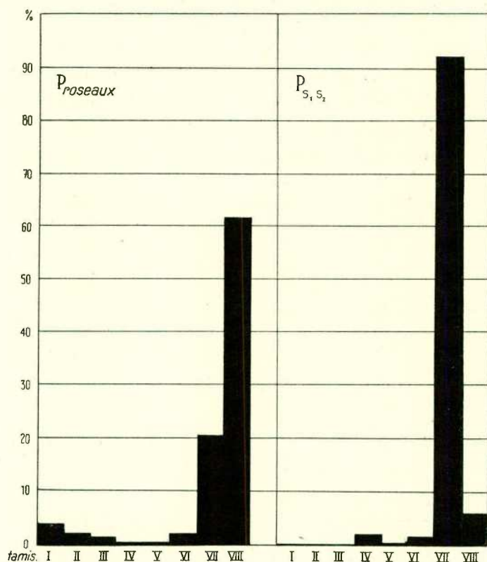
FIG. 20. — Triage mécanique de la vase.
