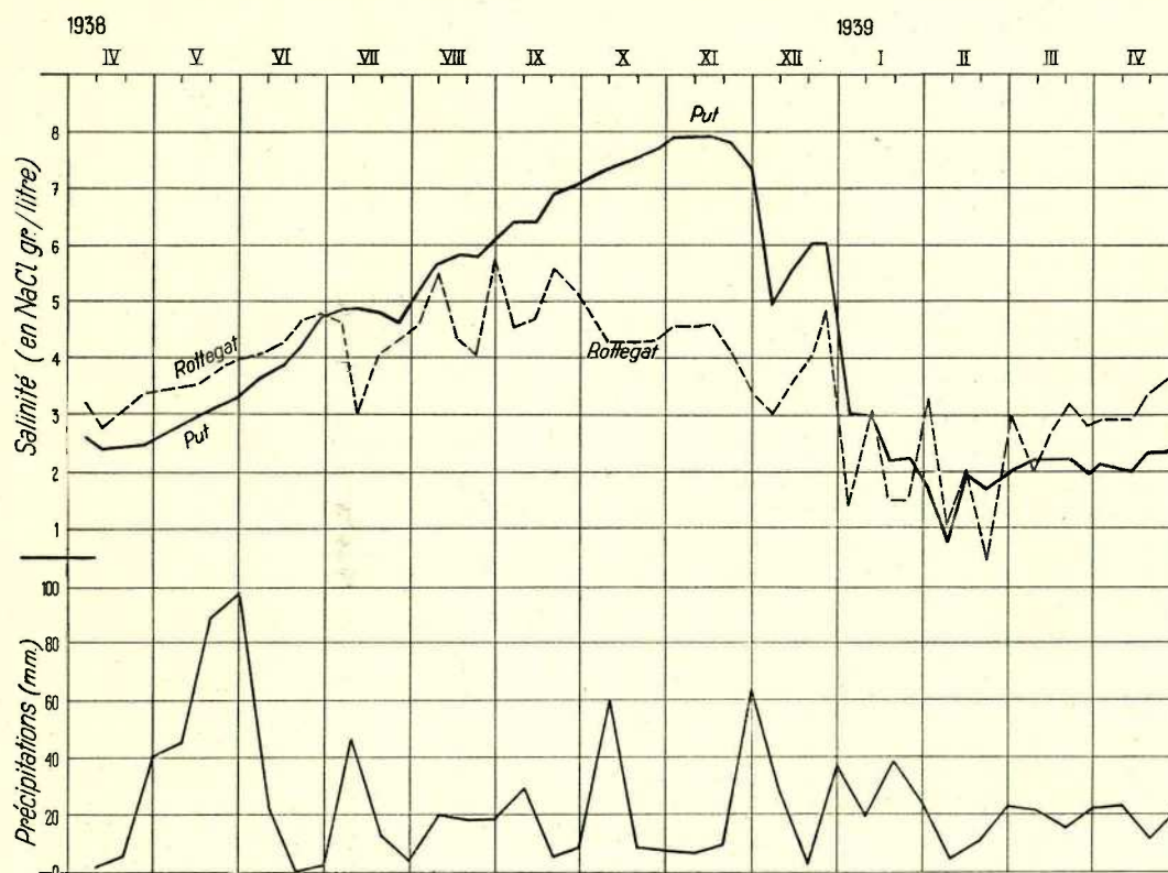
FIG. 12. — Variations de la salinité (analyses hebdomadaires) de l'eau du Put et du Rottegat. Précipitations.
