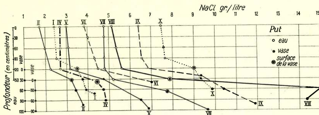
FIG. 11. — Variations verticales de la salinité.
