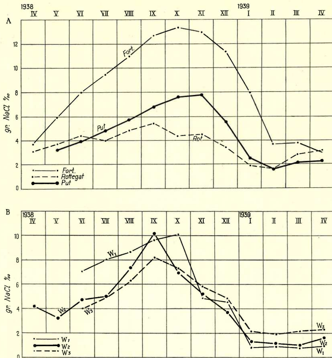
FIG. 28. — Salinité moyenne (mensuelle) des diverses stations explorées.
