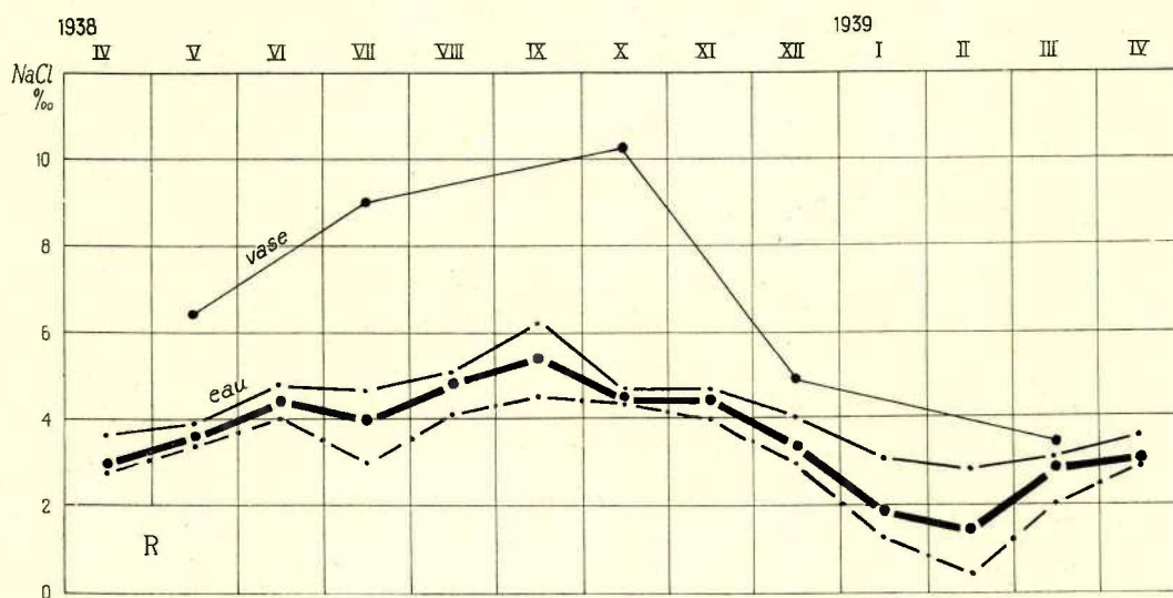
FIG. 21. — Variation saisonnière de la salinité (Rottegat).
