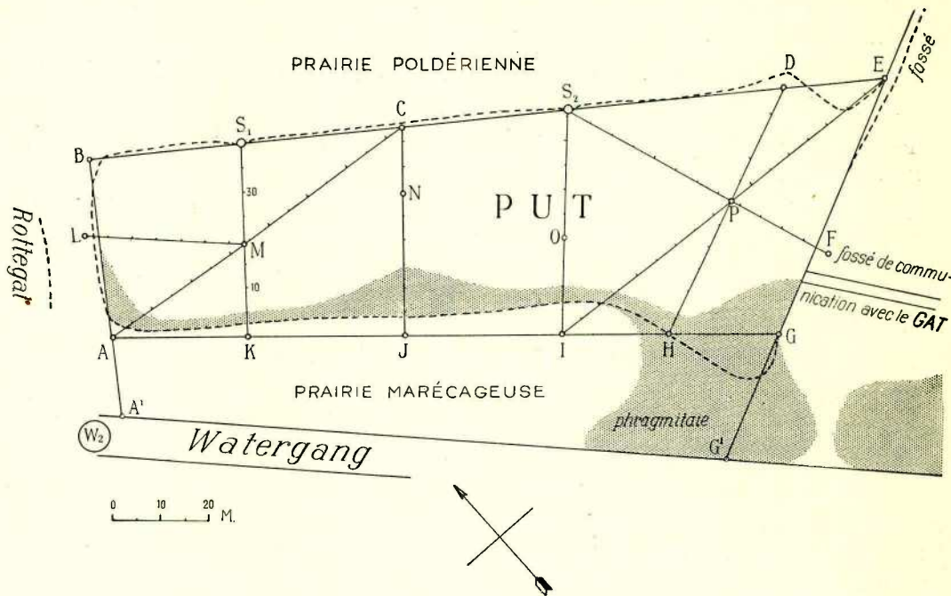
FIG. 3. — Étude hydrographique du Put.
