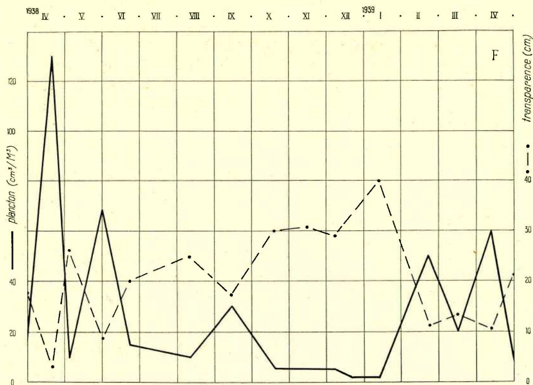
FIG. 24. — Quantité de plancton et transparence (fossés des fortifications).
