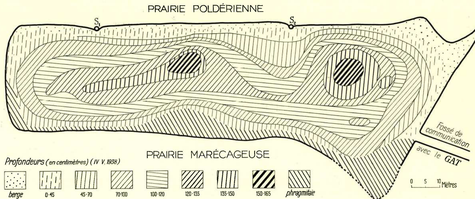
FIG. 17. — Considérations bathymétriques.
