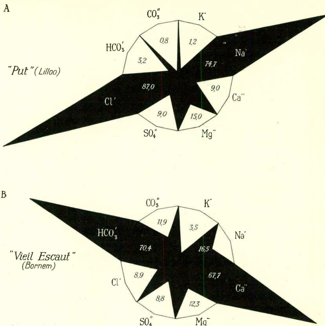
FIG. 10. — Représentation graphique des caractéristiques biochimiques d'une eau.
