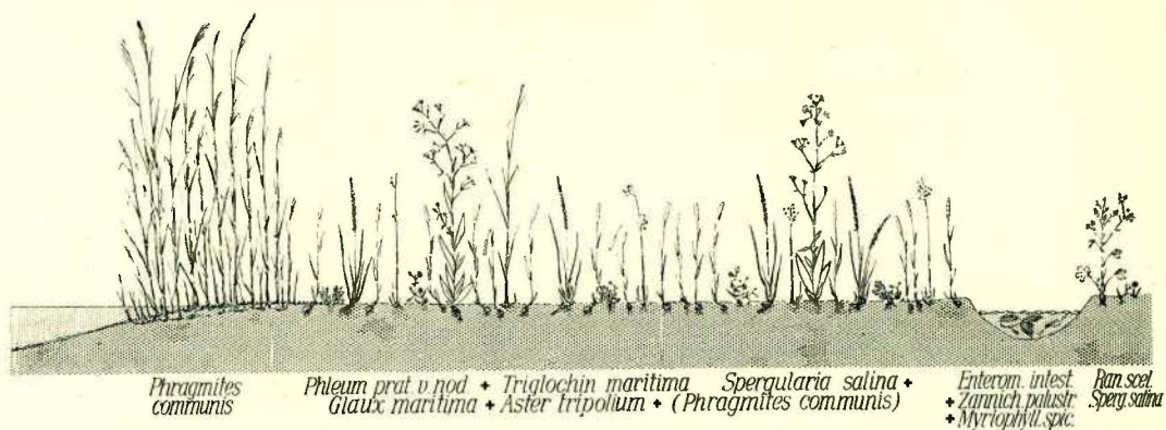
FIG. 15. — Schéma des associations végétales (berge sud et prairie marécageuse).
