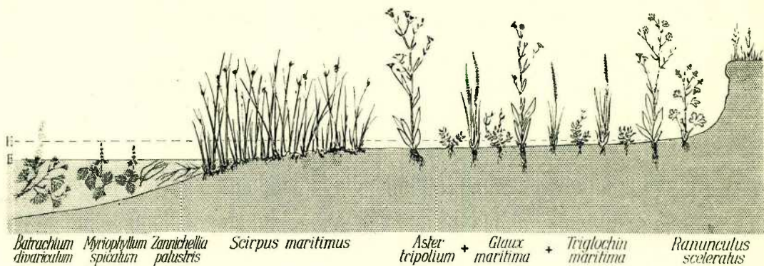
FIG. 16. — Schéma des associations végétales (berge poldérienne).
