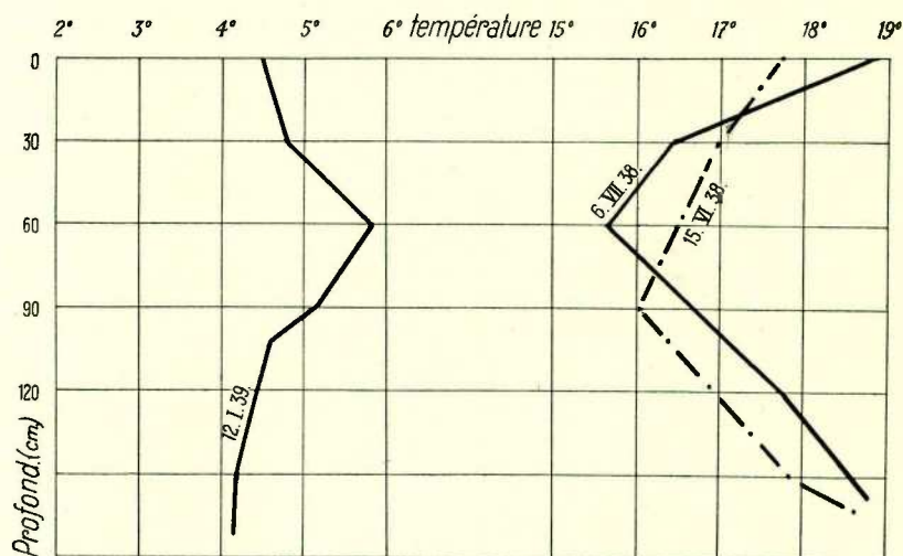
FIG. 8. — Variations verticales de la température dans la vase.
