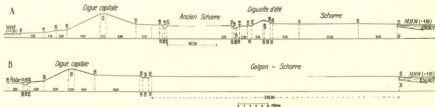
FIG. 18. — Coupe de la berge de l'Escaut, des digues, du schorre, etc. : A, à 800 mètres en amont de l'église de Lilloo; B, à 600 mètres en aval. (Due à l'obligeance du « Bijzondere Dienst der Zeeschelde », à Anvers.)
