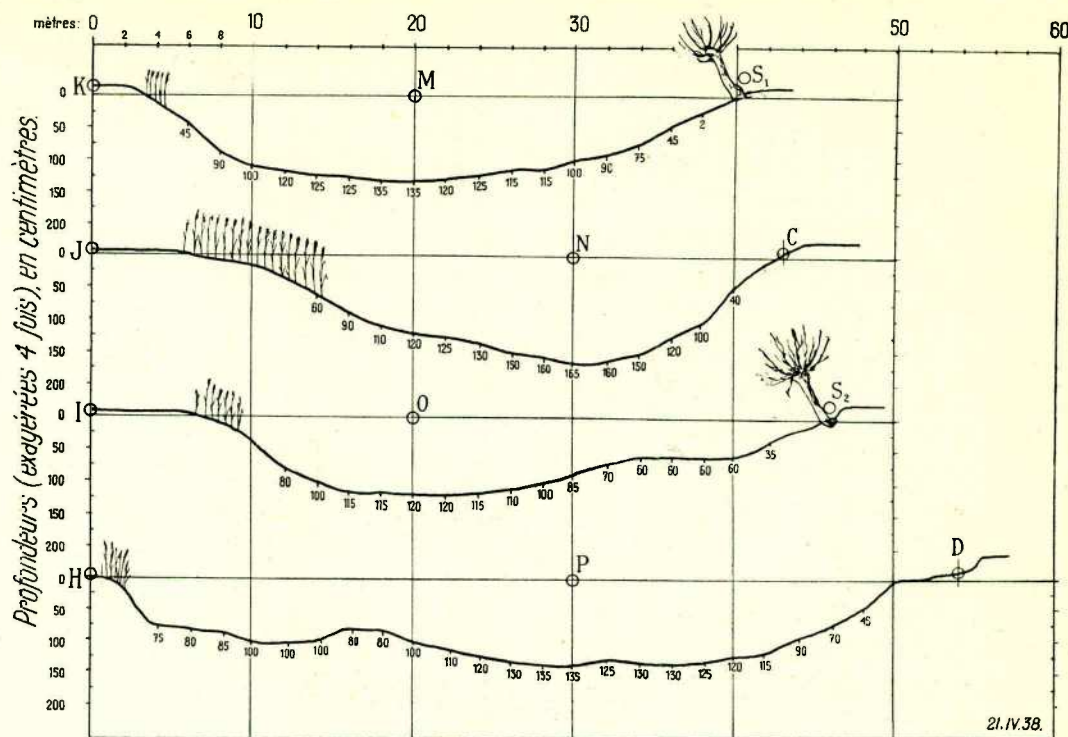
FIG. 5. — Coupes suivant divers profils. (Les profondeurs ont été exagérées 4 fois.)
