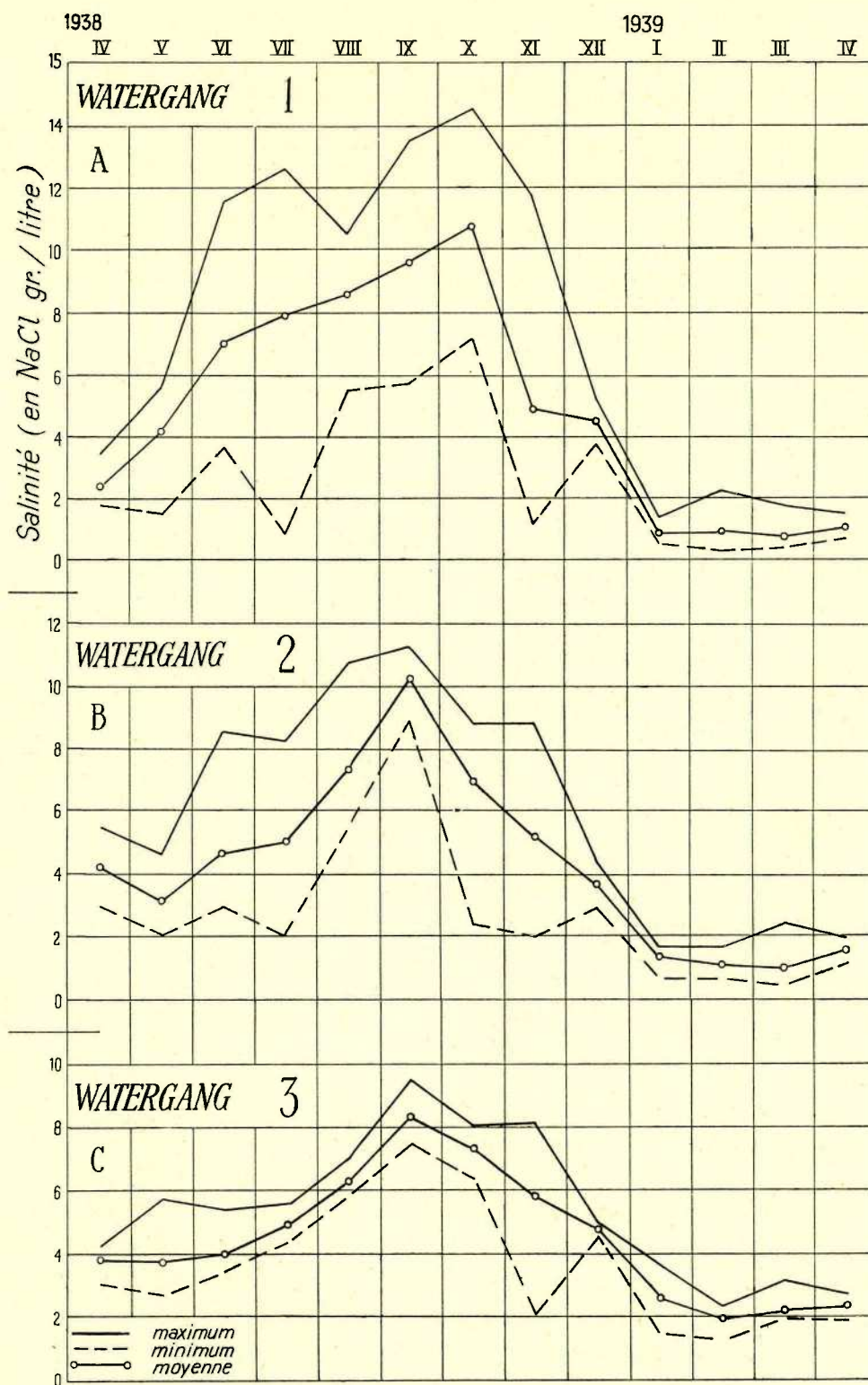
FIG. 23. — Variations saisonnières de la salinité du Watergang, aux stations W_1 , W_2 et W_3 (valeurs moyennes mensuelles).
