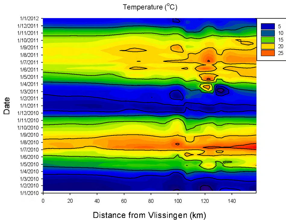
Figure 7.6. Contourplot temperatuursverloop.
