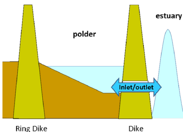
Figuur 10.2 Sluisprincipe bij de aantakking Burchtse Weel
