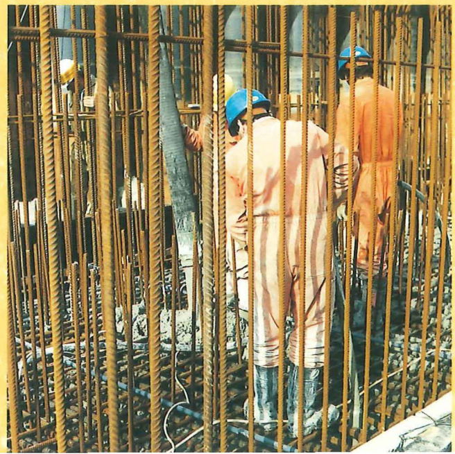
Betonwapening van scharnierfundatie: 'het wapeningsbos'
