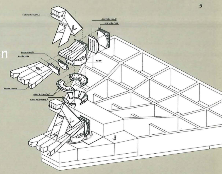
Bolscharnier
