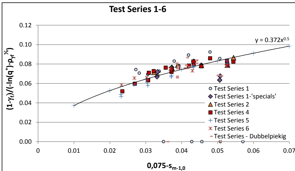
Figuur 4.21: Voor overslag en nieuwe ruwheidsdichtheid gecorrigeerde ruwheidsparameter ten opzichte van de lokale golfsteilheid; Testseries 1-6 + specials + dubbelpiekgige spectra
