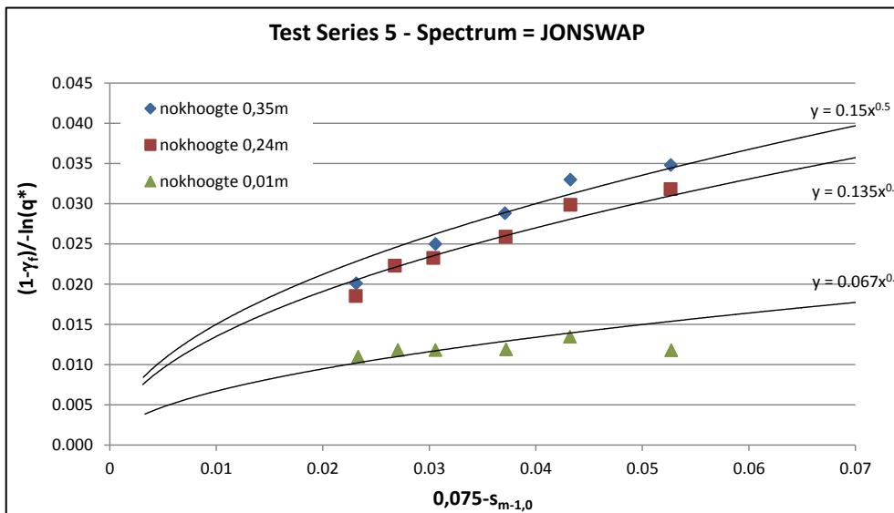
Figuur 4.4: Voor overslag gecorrigeerde ruwheidsparemeten ten opzichte van de lokale golfsteilheid: drie verschillende nokhoogtes
