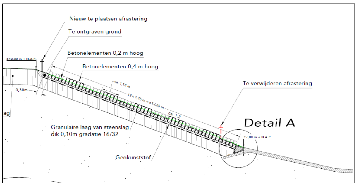
Figuur D.2: Dwarsdoorsnede dambordpatroon voorbeeld 1
