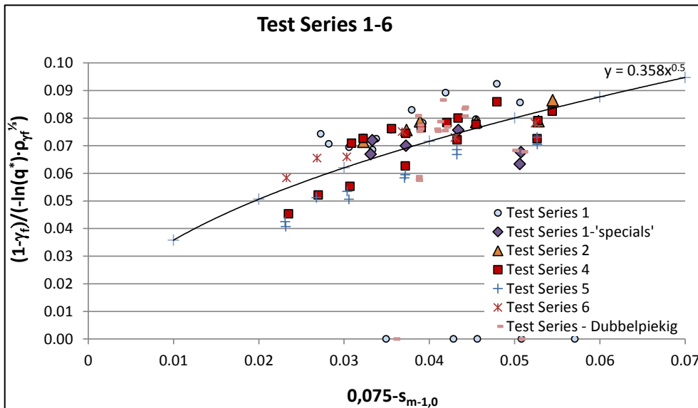
Figuur 4.15: Voor overslag en ruwheidsdichtheid gecorrigeerde ruwheidsparameter ten opzichte van de lokale golfsteilheid; Testseries 1-6 + specials + dubbelpiekgige spectra
