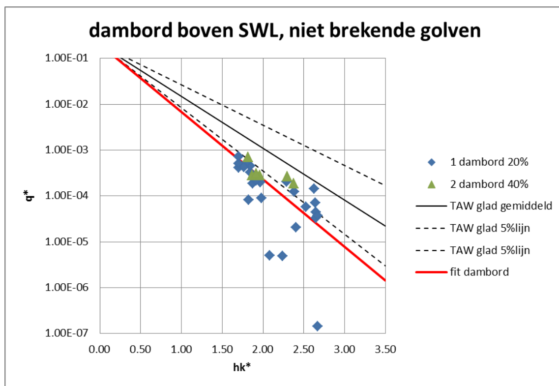
Figuur 7.6 Metingen t.o.v. TAW (2002) voor talud met dambord boven SWL en met niet-brekende golven
