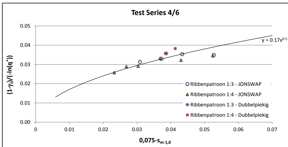
Figuur 4.14: Voor overslag gecorrigeerde ruwheidsparemeter ten opzichte van de lokale golfsteilheid; taludhelling 1:3 en 1:4
