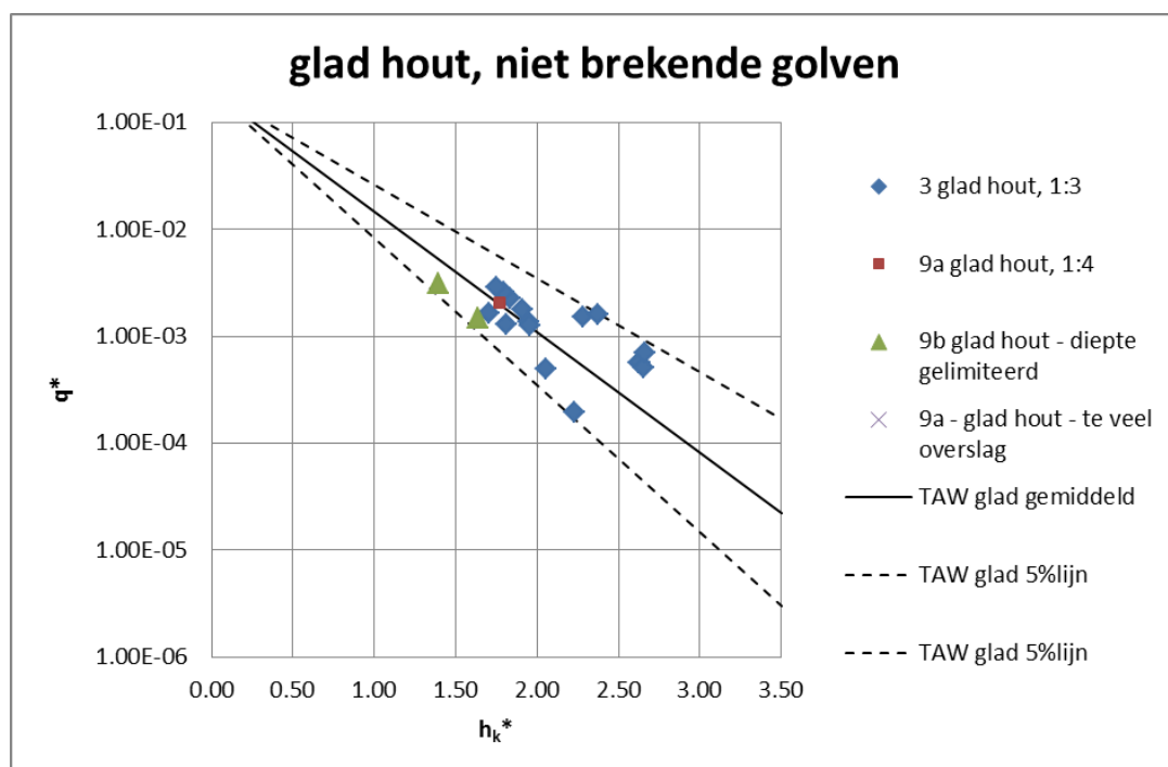
Figuur 7.2 Metingen t.o.v. TAW (2002) voor talud van glad hout met niet-brekende golven
