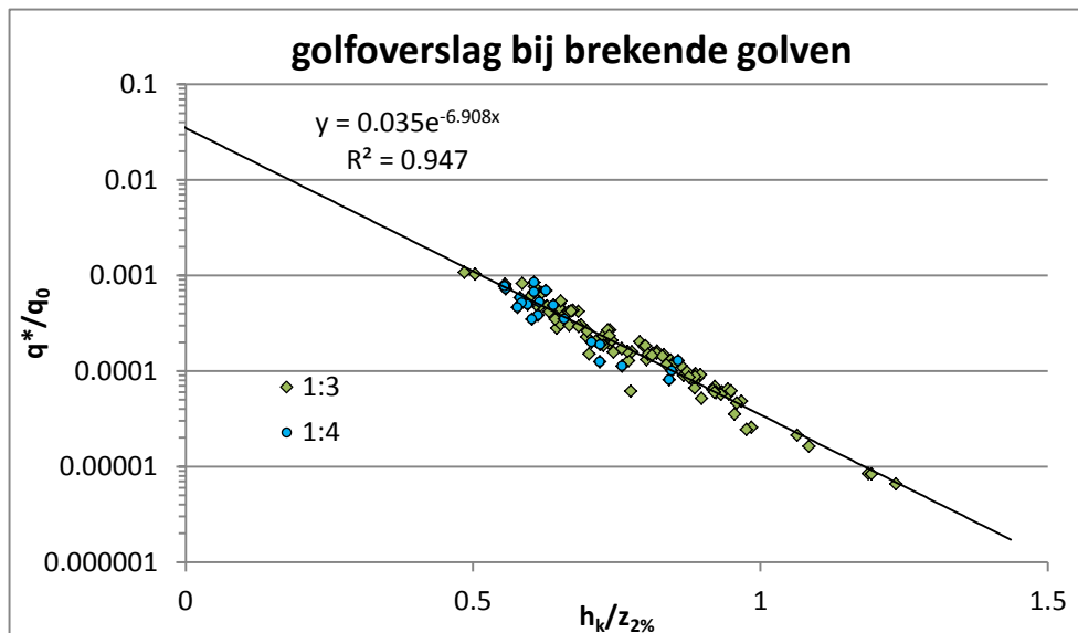
Figuur 4.29 Golfverslag bij brekende golven op basis nieuwe overslag formule.
