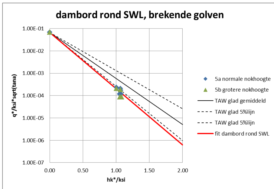
Figuur 7.9 Metingen t.o.v. TAW (2002) voor talud met dambord rond SWL en met brekende golven
